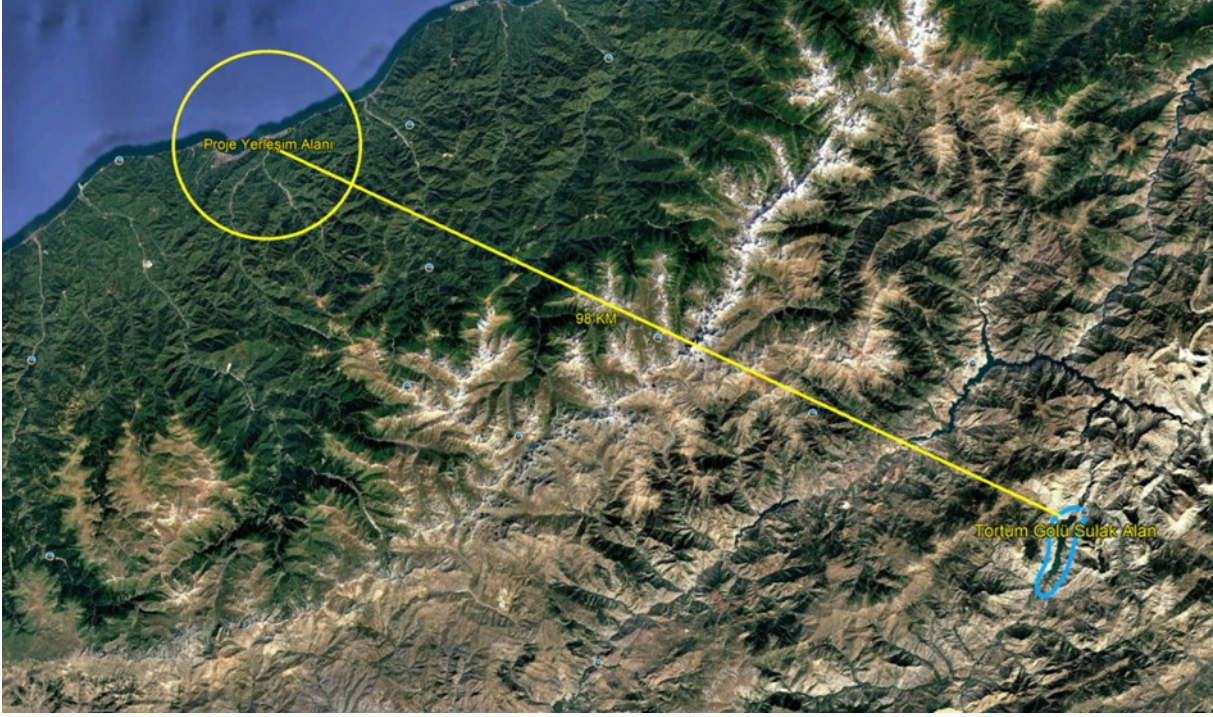
Şekil 7 Tortum Gölü Sulak Alanı'nın Konumunu Gösterir Uydu Görüntüsü
