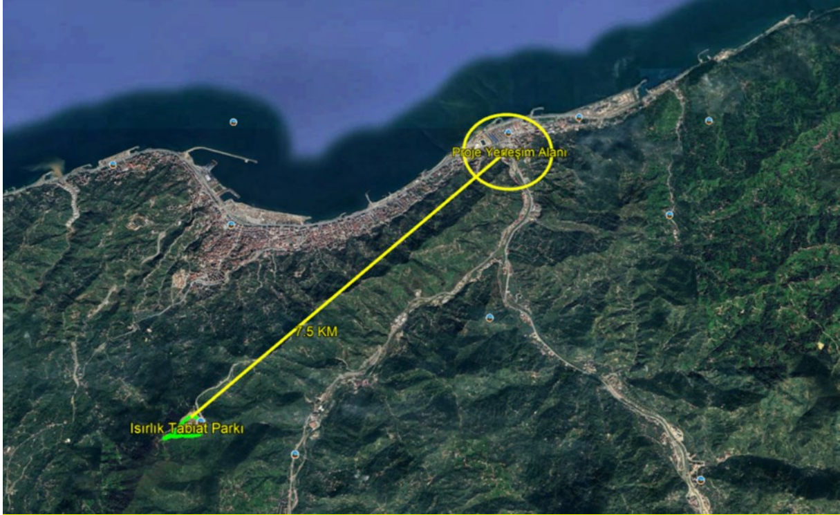
Şekil 6 Isırlık Tabiat Parkı'nın Konumunu Gösterir Uydu Görüntüsü
