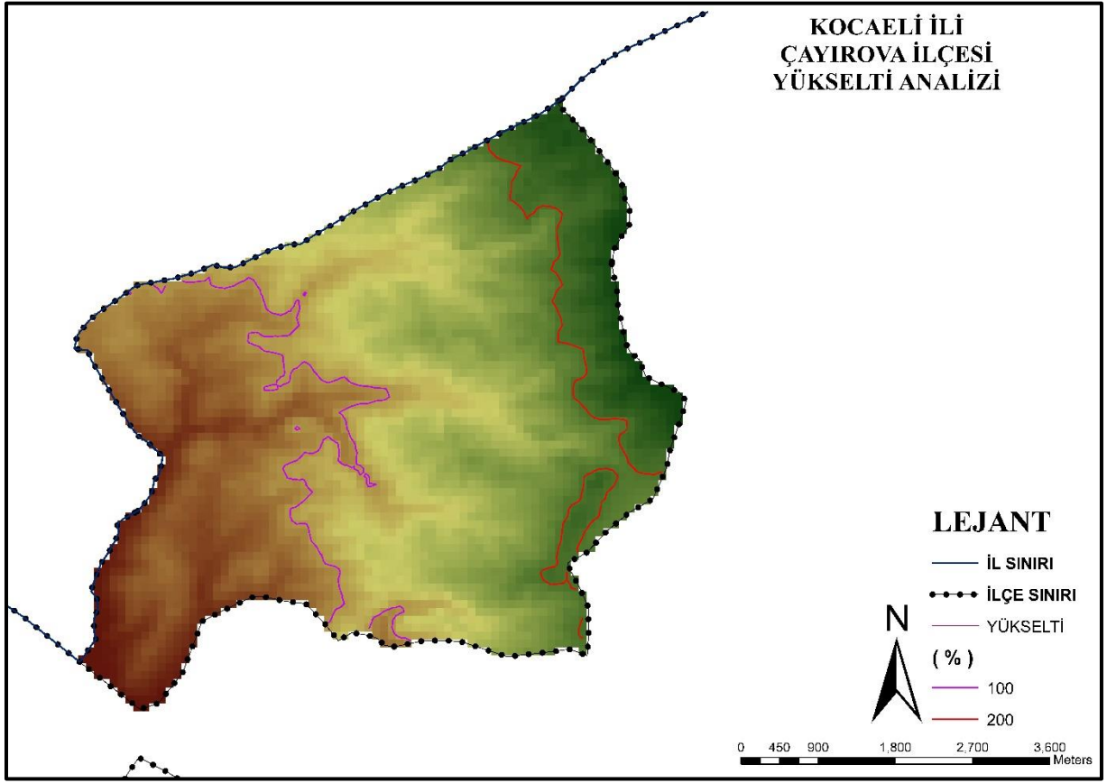
Harita 8:Kocaeli İlçesi Çayirova İlçesi Yükselti Analizi
