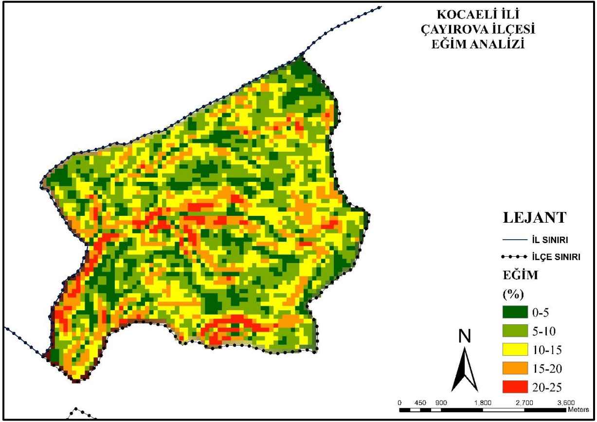
Harita 7:Kocaeli İli Çayirova İlçesi Eğim Analizi
