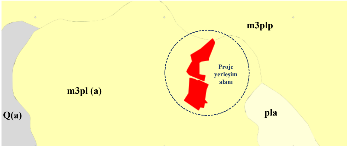
Şekil 5 .GES ve Yakın Çevresinin Genel Jeolojisi
