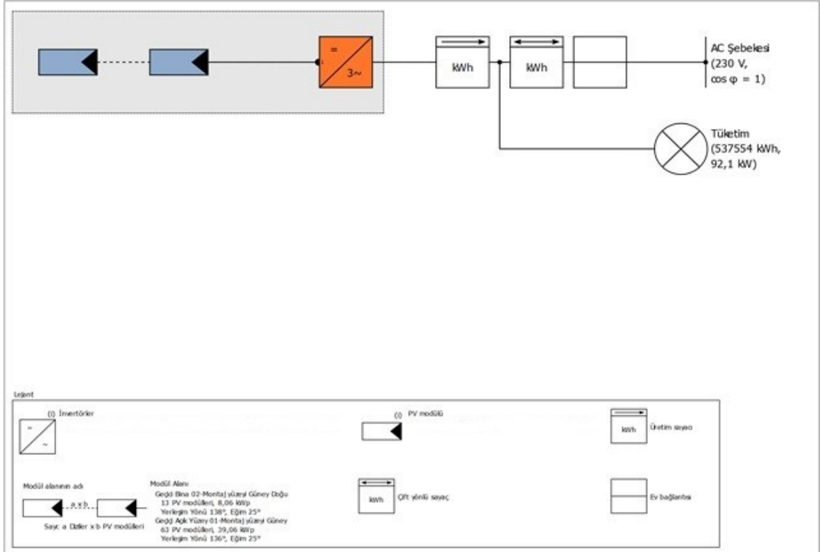
Şekil 3 Tek Hat Şeması
