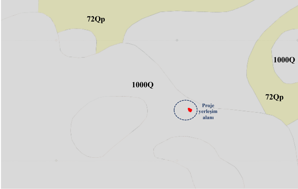
Şekil 5 .GES ve Yakın Çevresinin Genel Jeolojisi
