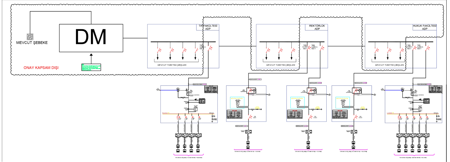
Şekil 6. Tek Hat Şeması
