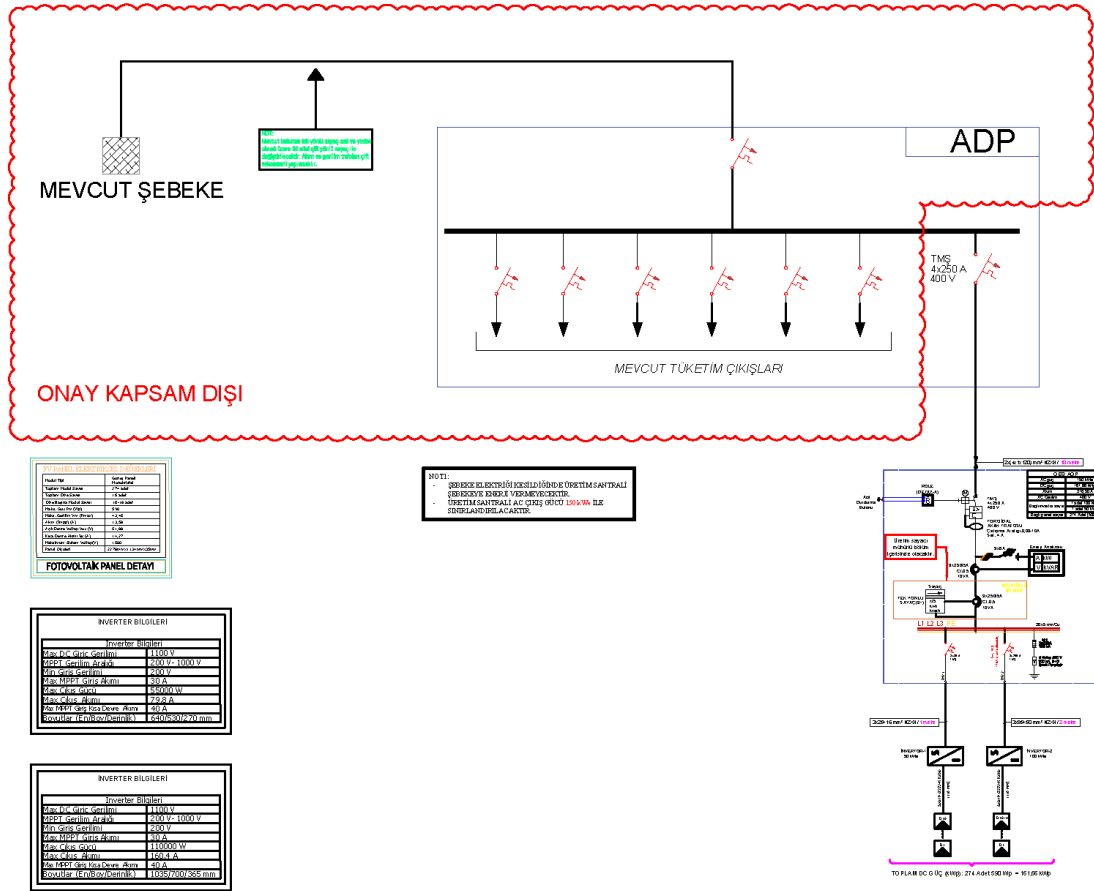
Şekil 3. Tek Hat Şeması
