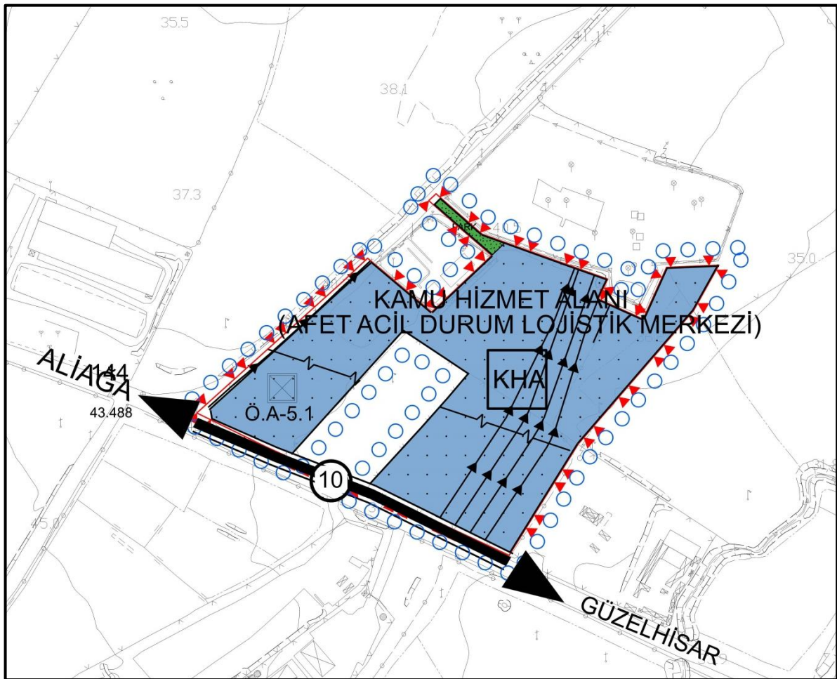
Şekil 10. 1/5000 Ölçekli Nazım İmar Planı
