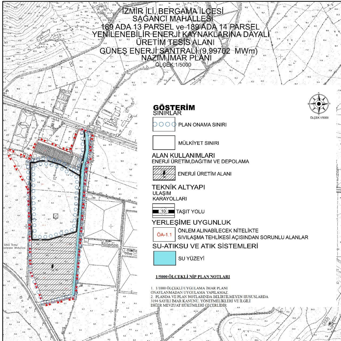
Şekil 6. 1/5000 Ölçekli Nazım İmar Planı
