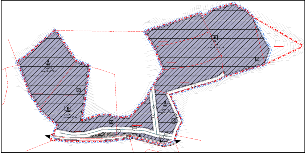
Harita 4,1/1000 Ölçekli Uygulama İmar Planında GES Alanı
