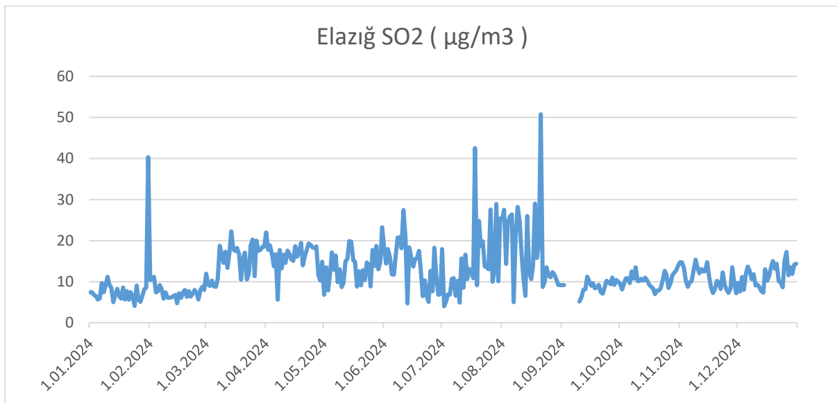
Grafik 2- 2024 yılında Elazığ istasyonu SO 2 parametresi günlük ortalama değer grafiği* (havaizleme.gov.tr, 2025)
