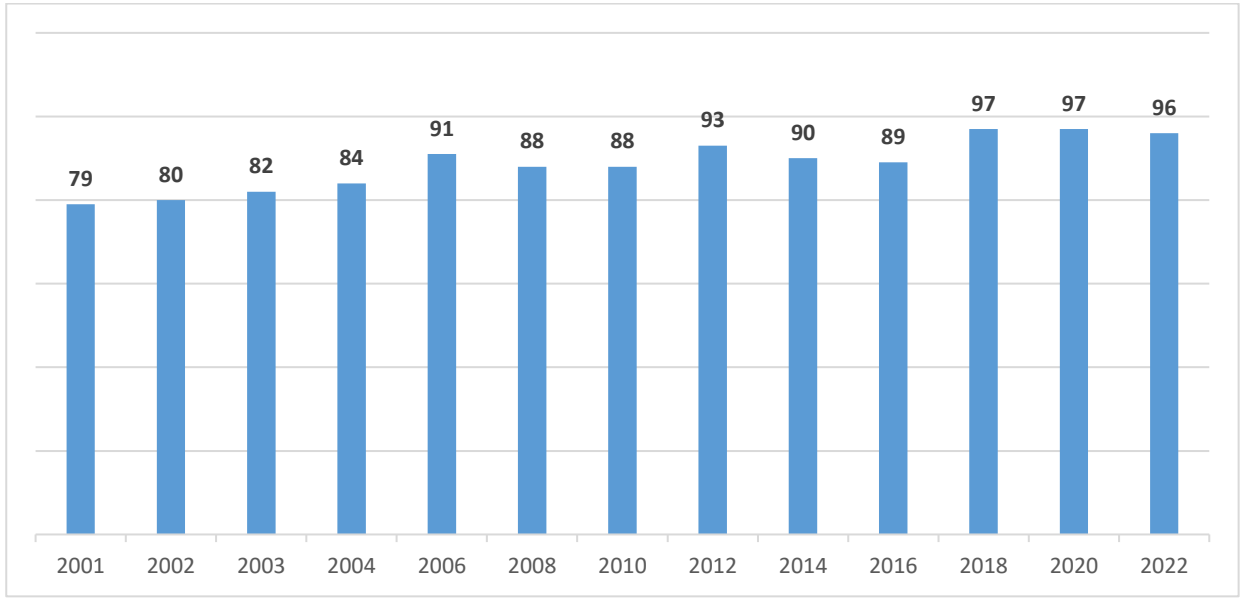
Grafik 5 – Yıllar bazında kanalizasyon şebekesi tesisi ile hizmet verilen belediye nüfusunun toplam nüfusa oranı
