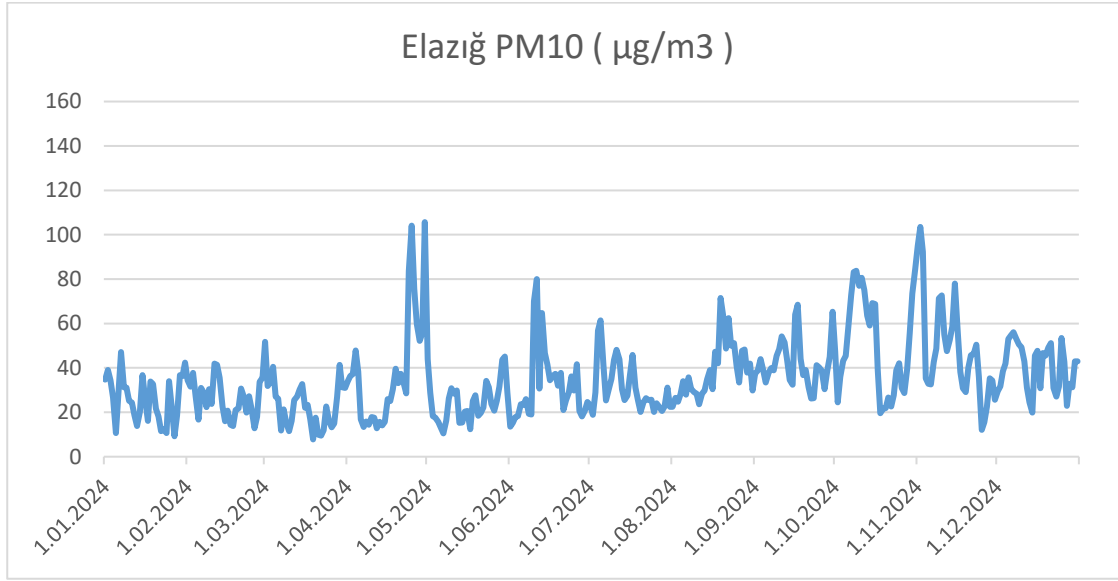
Grafik 1- 2024 yılında Elazığ istasyonu PM 10 parametresi günlük ortalama değer grafiği* (havaizleme.gov.tr, 2025)
