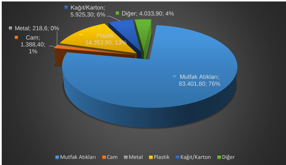
Grafik 8 – 2024 yılı itibariyle Belediye atık karakterizasyonu (Elazığ Belediye Başkanlığı, 2025)
