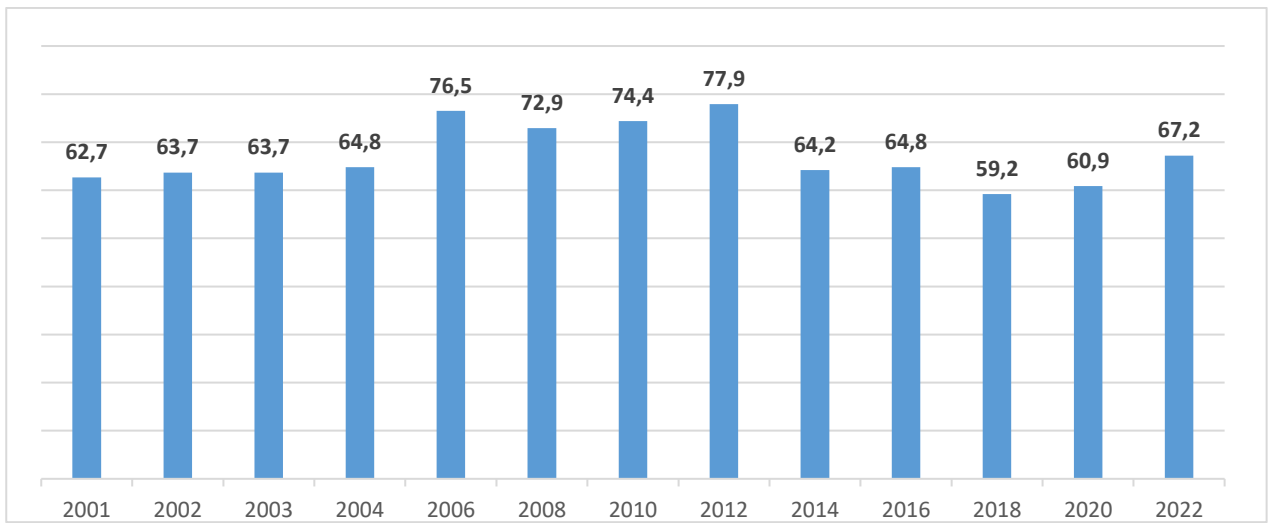
Grafik 6 – Yıllar bazında atıksu arıtma tesisi ile hizmet verilen belediye nüfusunun toplam belediye nüfusuna oranı
