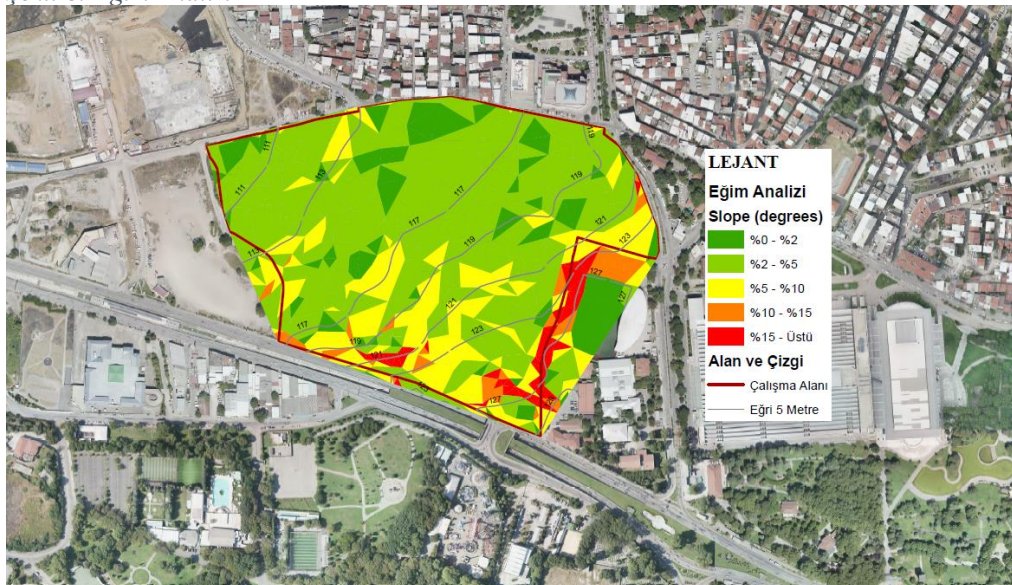
Şekil 6: Eğim Analizi
