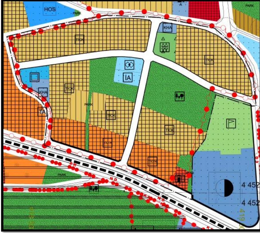
Şekil 10: 1/5.000 ölçekli Osmangazi Nazım İmar Planı Değişikliği
