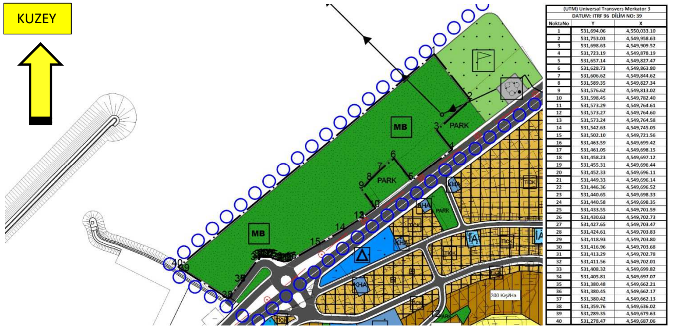
Şekil 18. Trabzon İli, Çarşıbaşı İlçesi, Burunbaşı ve Çarşıbaşı Mahallesi "Millet Bahçesi" 1/5000 Ölçekli Nazım İmar Planı Değişikliği Teklifi Alanına Ait Köşe Kırık Noktaları ve Bu Noktalara Ait Koordinat Değerleri
