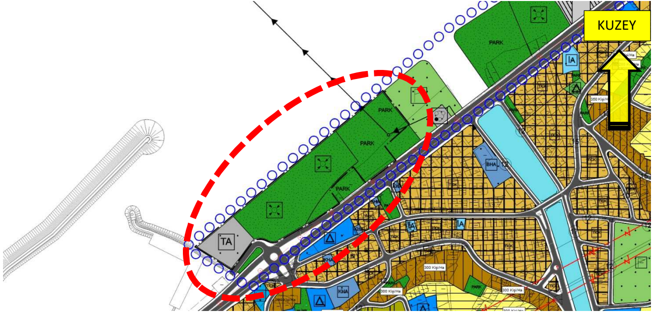
Şekil 14. Planlama Alanı Yakın Çevresini Kapsayan Kent Bütününe Yönelik Plan ile Kıyı Kenar çizgisinin kuzeyindeki Düzenleme Alanına ait 1/5000 Ölçekli Mer’i Nazım İmar Planı
