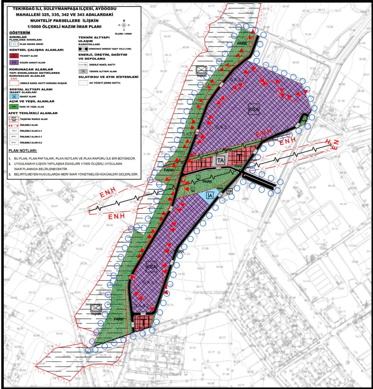
Harita 32: 1/5.000 Ölçekli Nazım İmar Planı
