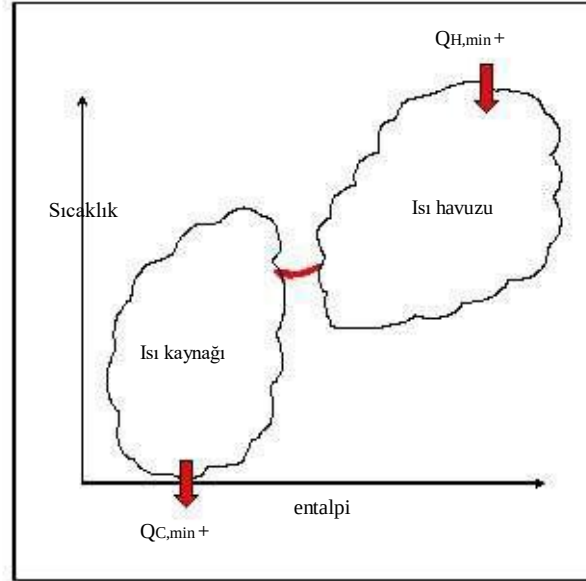
Şekil 2.15: Pinç boyunca ısı havuzundan ısı kaynağına ısı transferi
