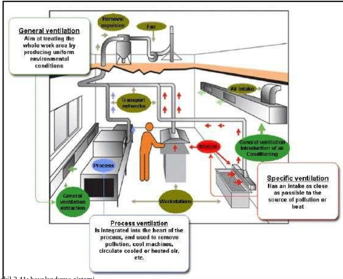
Şekil 3.41: havalandırma sistemi
