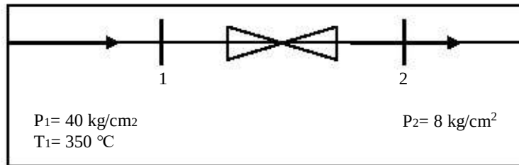
Şekil 7.2: Buhar kısma prosesi
