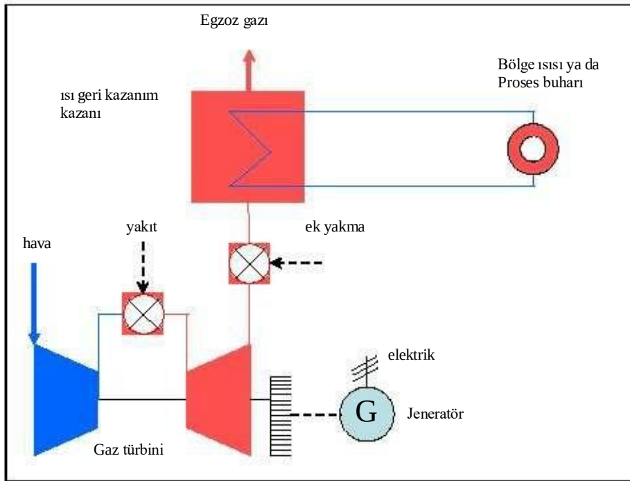
Şekil 3.14: gaz türbinli ısı geri kazanım kazanı [65, Nuutila, 2005]
