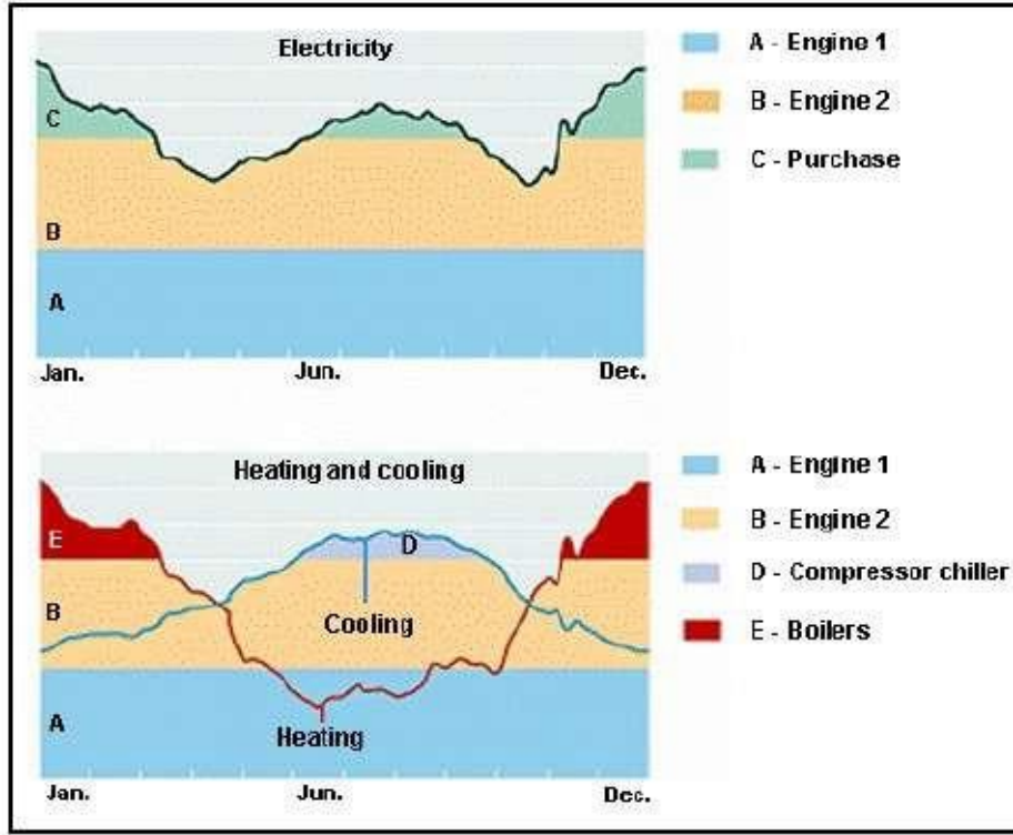
Şekil 3.19: trijenerasyon, yıl boyunca optimize tesis işletimi sağlar [64, Linde, 2005]
