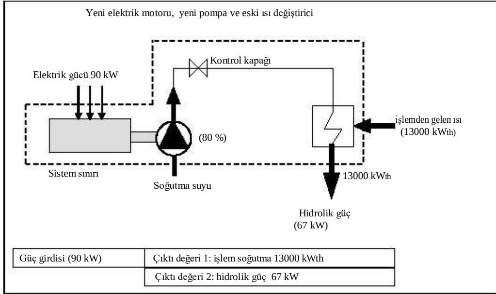
Şekil 1.15: yeni elektrik motoru, yeni pompa ve eski ısı değiştirici
