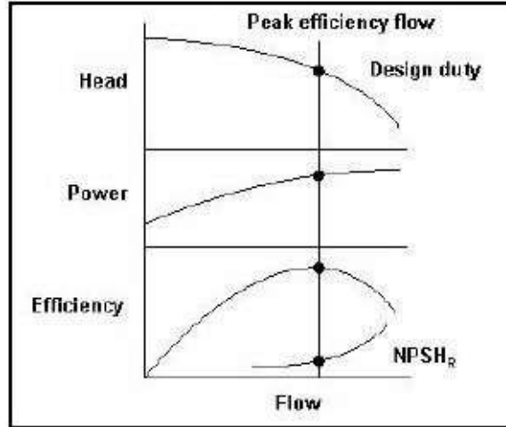
Şekil 3.35: en üst seviye verimlilik akışı karşısında yük, güç ve verimlilik [199, TWG]
