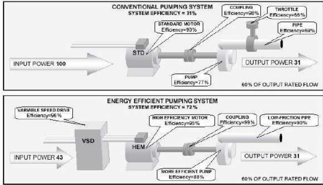
Şekil 3.25: konvansiyonel ve enerji tasarruflu pompalama sistemleri [246, ISPRA, 2008]
