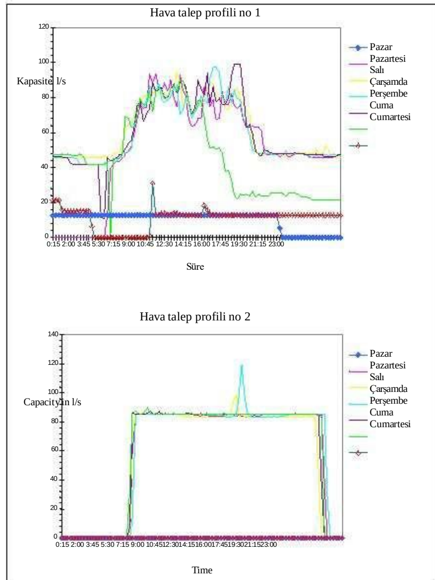
Şekil 3.33: farklı talep profilleri [168, PNEUROP, 2007]
