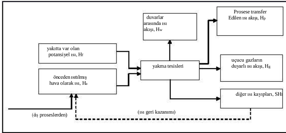
Şekil 3.1: Yakma tesisinin enerji dengesi [91, CEFIC, 2005]
