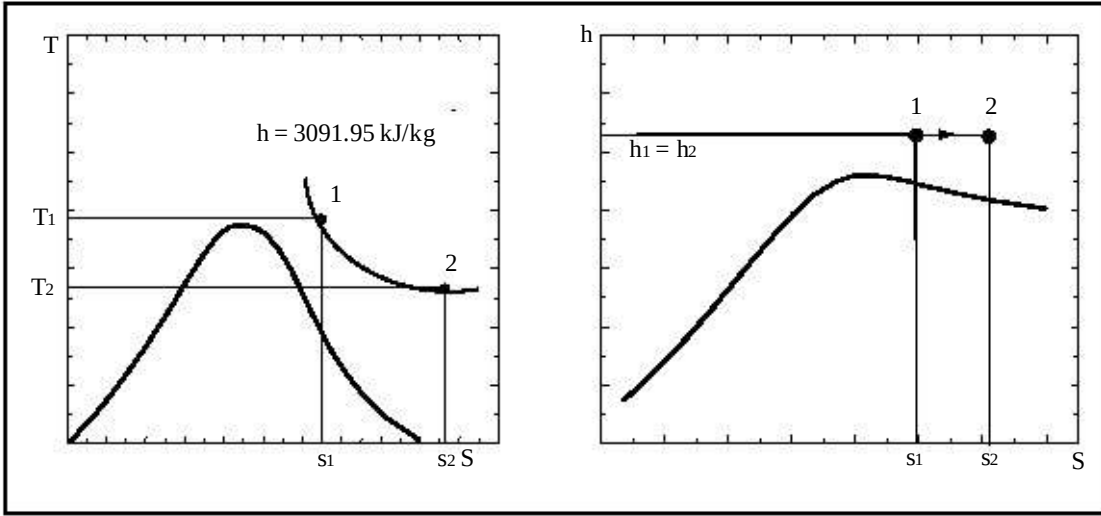
Şekil 7.3: örnek buhar kısma prosesinin T-S ve h-S diyagramları
