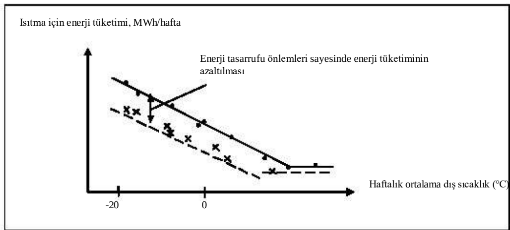
Şekil 1.17: Dış sıcaklığa bağlı olarak enerji tüketimi
