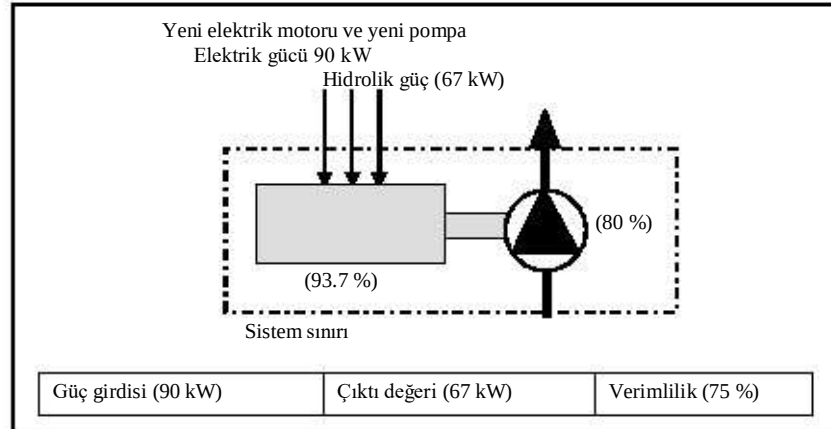
Şekil 1.13: sistem sınırı-yeni elektrik motoru ve yeni pompa
