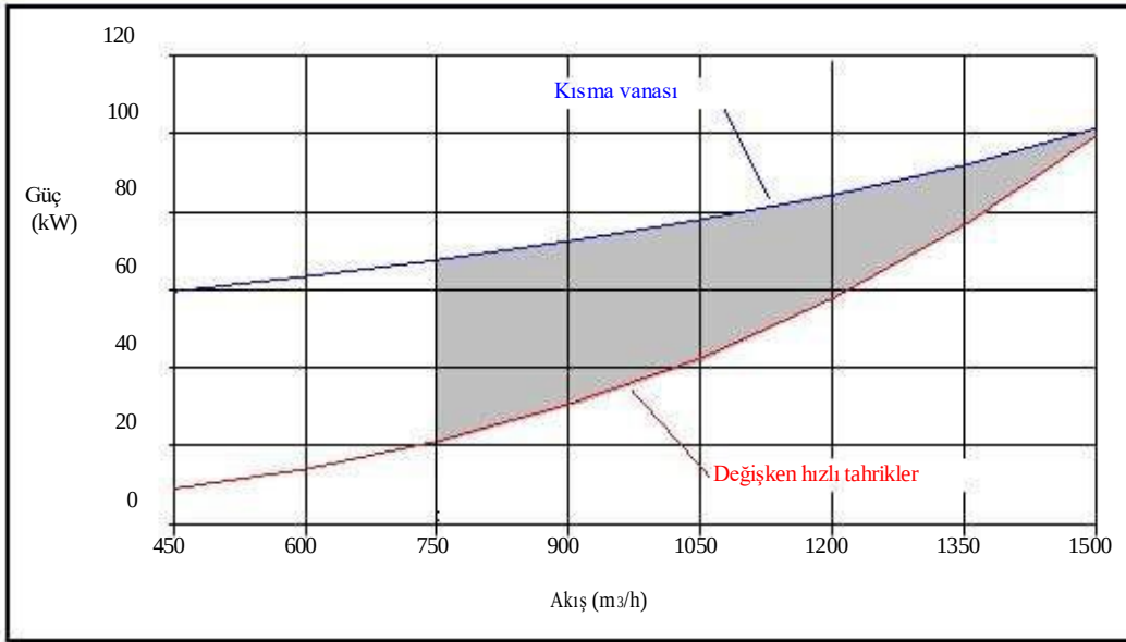
Şekil 3.38: rotodinamik pompa için iki adet pompalama düzenleme sisteminin enerji tüketimine ilişkin örnek
