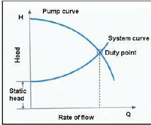
Şekil 3.37: pompa yükü karşısında akış oranı
