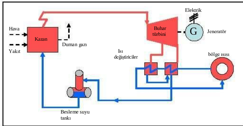
Şekil 3.12: geri basınç tesisi [65, Nuutila, 2005]
