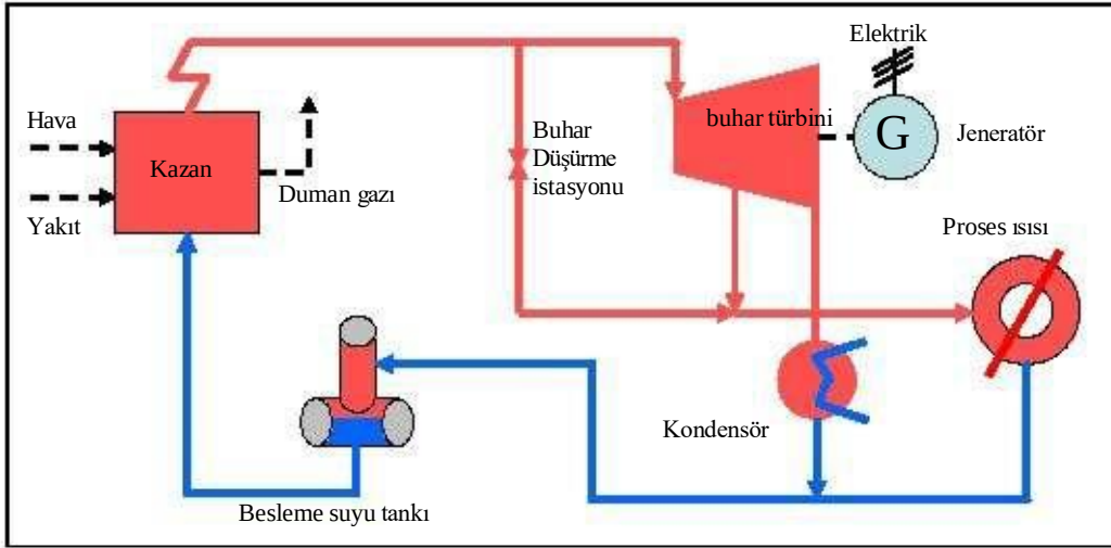
Şekil 3.13: ara buharlı kondensasyon tesisi [65, Nuutila, 2005]
