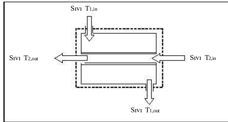
Şekil 7.4: ısı değıştircinin ters akışlı
