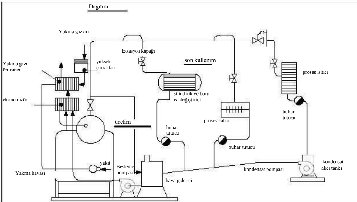
Şekil 3.5: buhar üretimi ve dağıtım sistemi [123, US_DOE]
