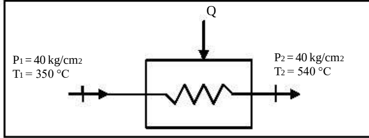
Şekil 7.5: buhar akışının ara ısıtma prosesi
