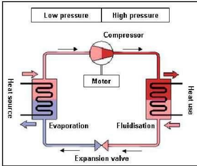
Şekil 3.8: sıkıştırma ısı pompası [28, Berger, 2005]
