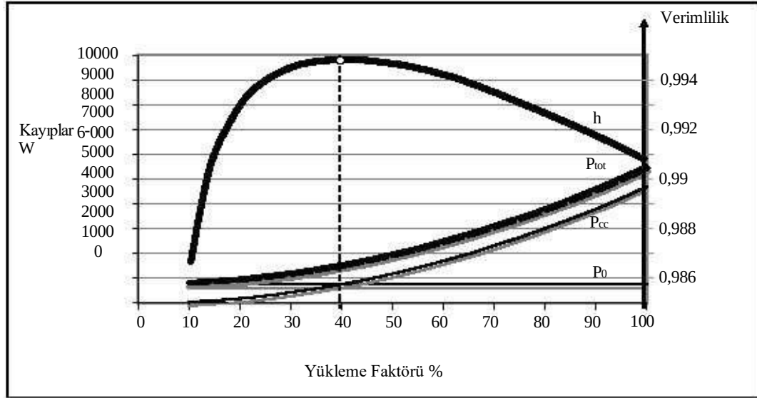
Şekil 3.24: demir, bakır, verimlilik ve yük faktörü kayıpları arasındaki ilişki [245, Di Franco, 2008]
