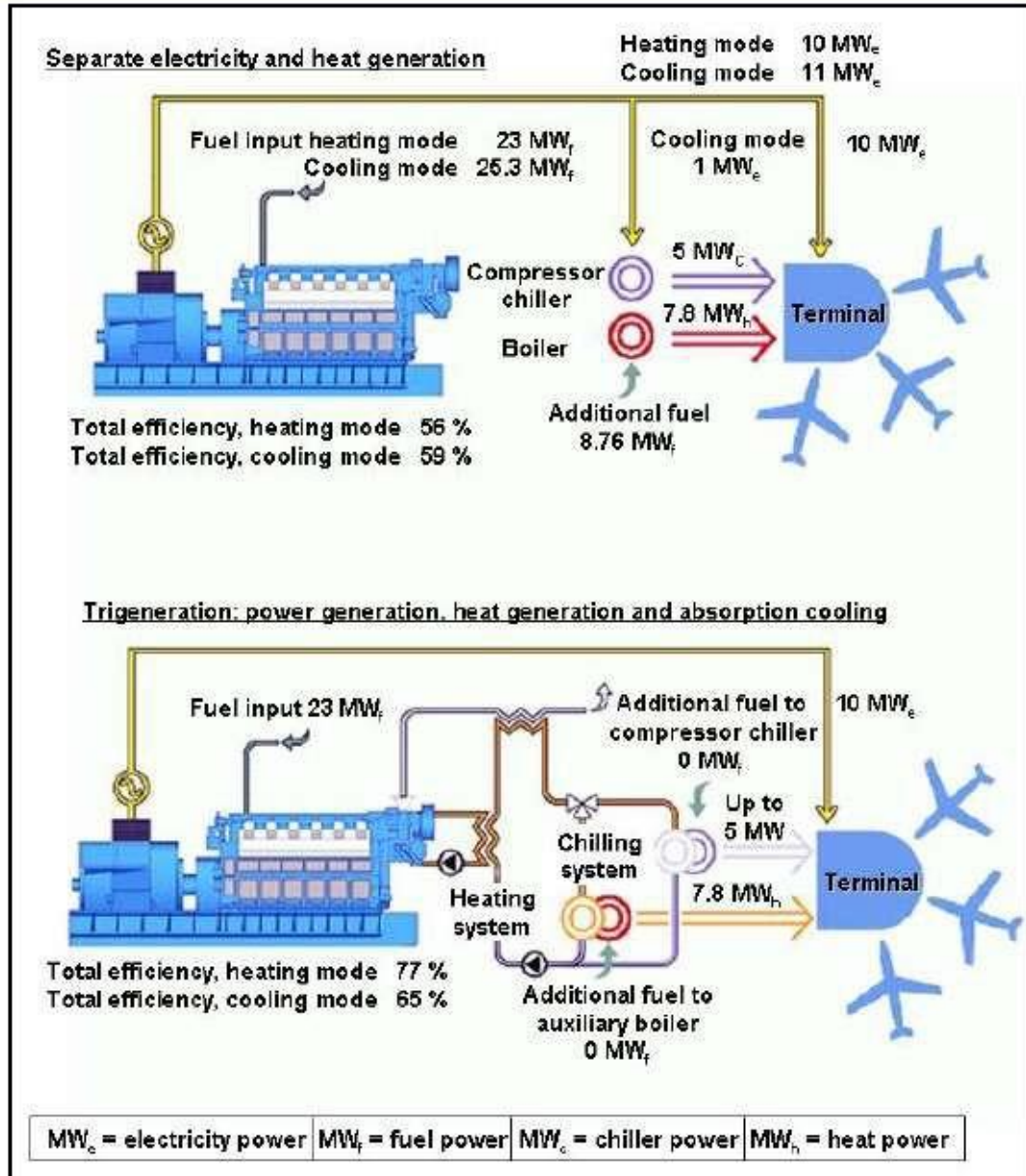
Şekil 3.18: bir havalimanı için ayrı enerji üretimi ile karşılaştırılan trijenerasyon [64, Linde, 2005]
