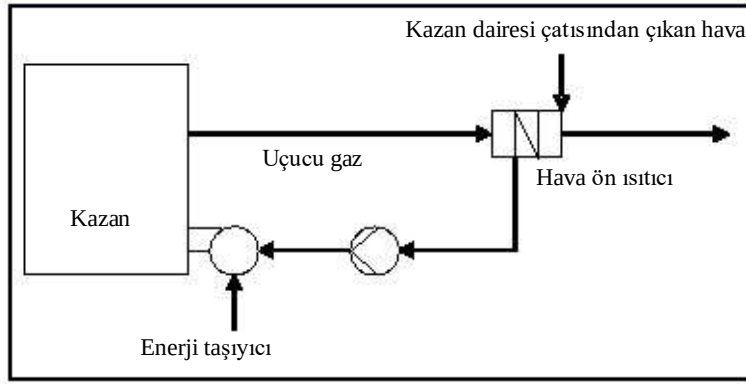
Şekil 3.2.: hava ön ısıtıcının bulunduğu yakma sistemi şeması [28, Berger, 2005]
