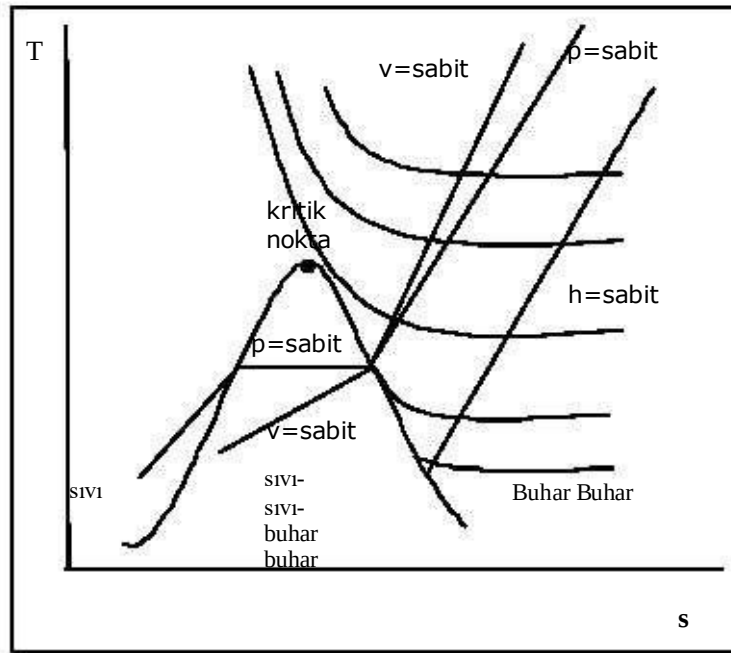
Şekil 7.1: Sıcaklık-entropi diyagramı
