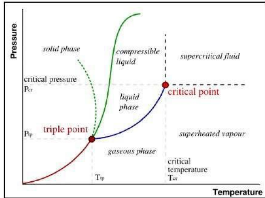
Şekil 1.5: Basınç – sıcaklık (faz) diyagramı [153, Wikipedia]
