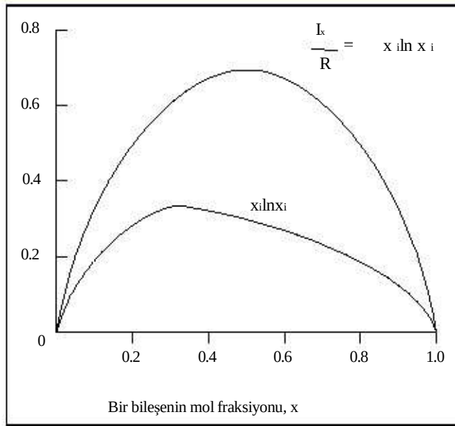
Şekil 7.7: I_k/RT_0 karşısında karışımdaki bir bileşenin Molar fraksiyonu
