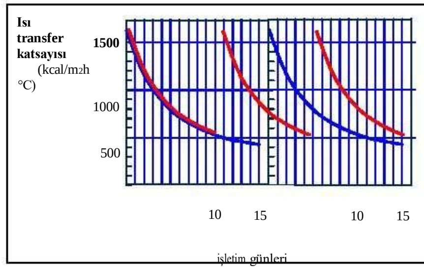
Şekil 7.15: ısıtıcıların işletim devri [48, Teodosi, 2005]
