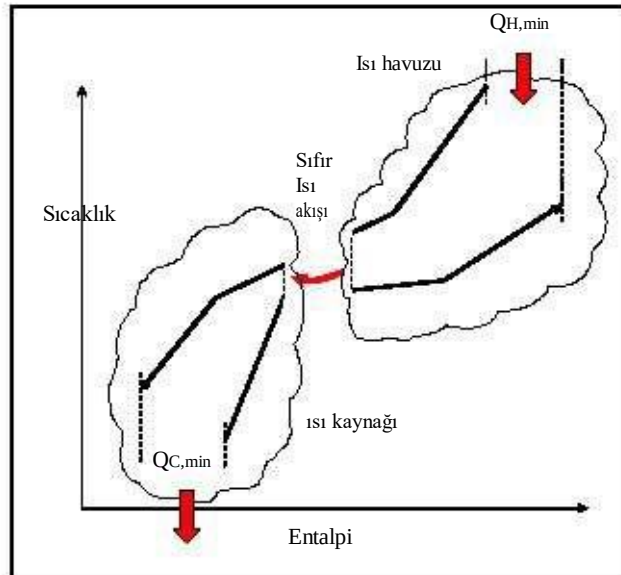
Şekil 2.14: Pinç altı ve piç üstü sistemlerinin şematik olarak gösterilmesi
