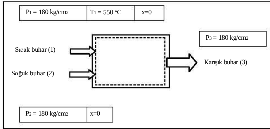
Şekil 7.8: İki akışın karışım haznesi
