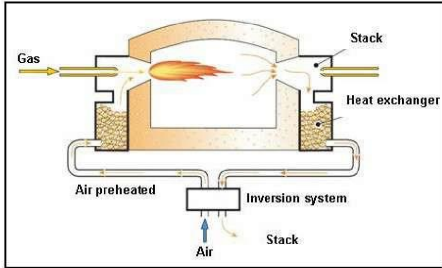
Şekil 5.1: regeneratif kazanların çalışma ilkesi [277, ADEME]
