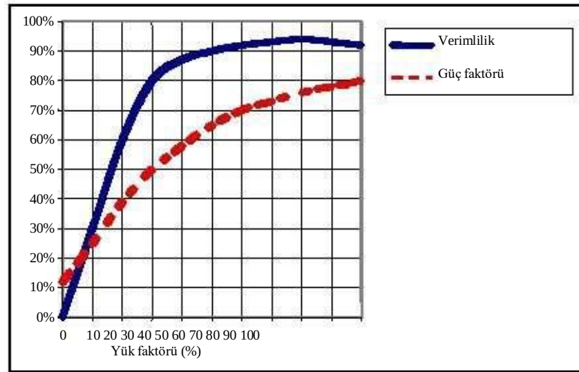
Şekil 2.17: yük faktörüne bağlı olan bir aracın güç faktörü [11, Franco, 2005]
