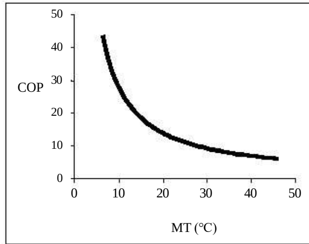
Şekil 3.11: MRV sisteminde COP karşısında sıcaklık yükselişi [18, Åsbland, 2005]
