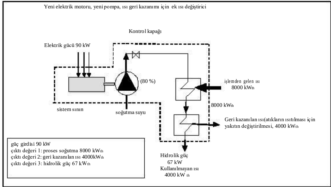
Şekil 1.16: yeni elektrik motoru, yeni pompa ve iki adet ısı değiştirici
