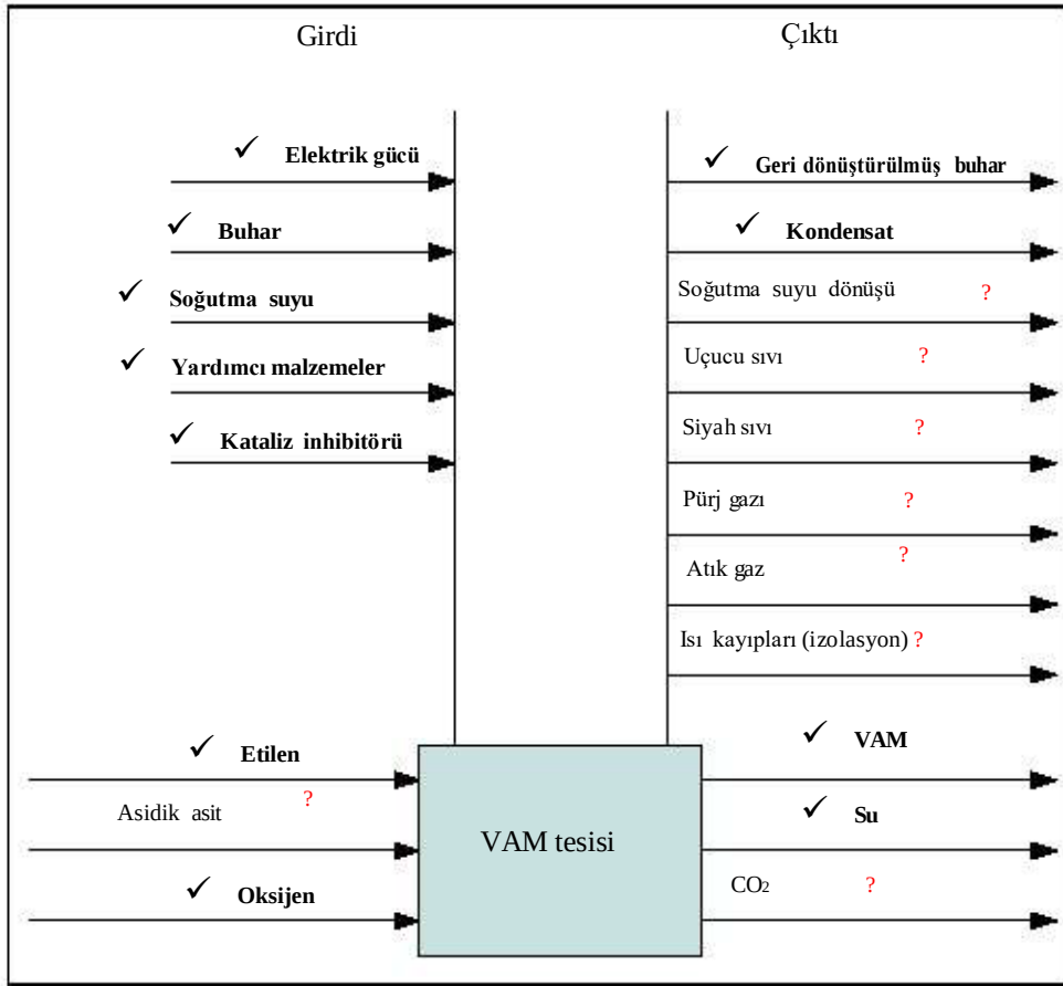
Şekil 7.10: Vinil asetat monomer tesisi (VAM) için girdi ve çıktılar
