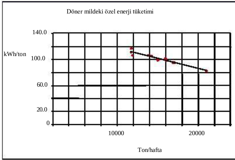
Şekil 7.12: döner mildeki özel enerji tüketimi
