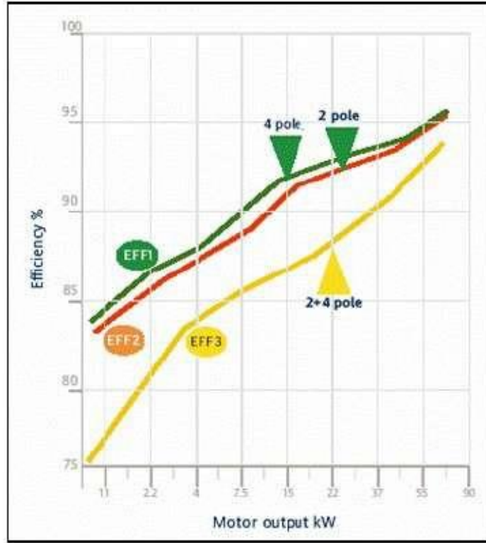
Şekil 3.27: Üç fazlı AC endüksiyon motorlarının enerji verimliliği
