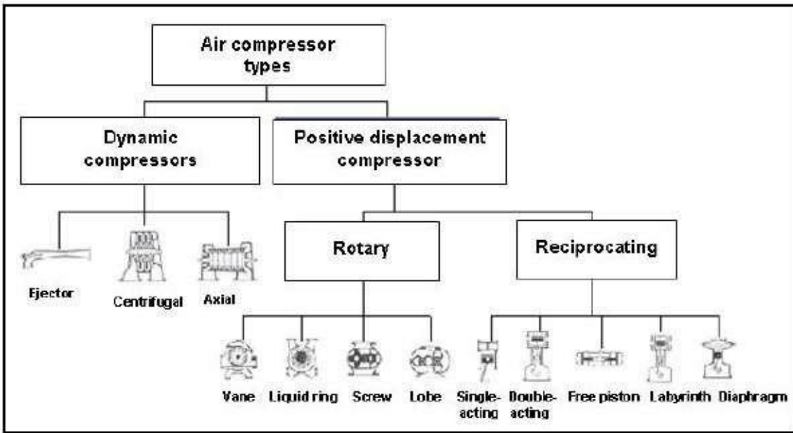
Şekil 3.32: kompresör çeşitleri [168, PNEUROP, 2007]
