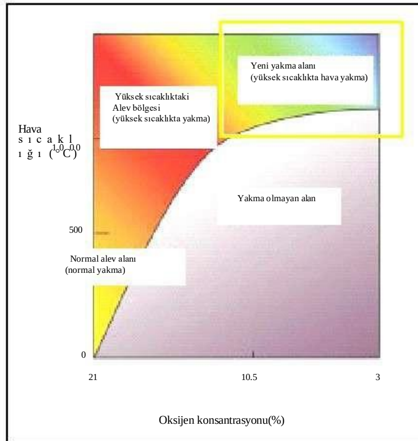
Şekil 3.4: yakma işlemindeki farklı bölgeler [17, Åsbländ, 2005]
