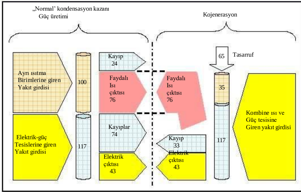
Şekil 3.17: kondensasyon gücü tesisi ile kombine ısı ve güç tesisinin verimliliğinin kıyaslanması [65, Nuutila, 2005]
