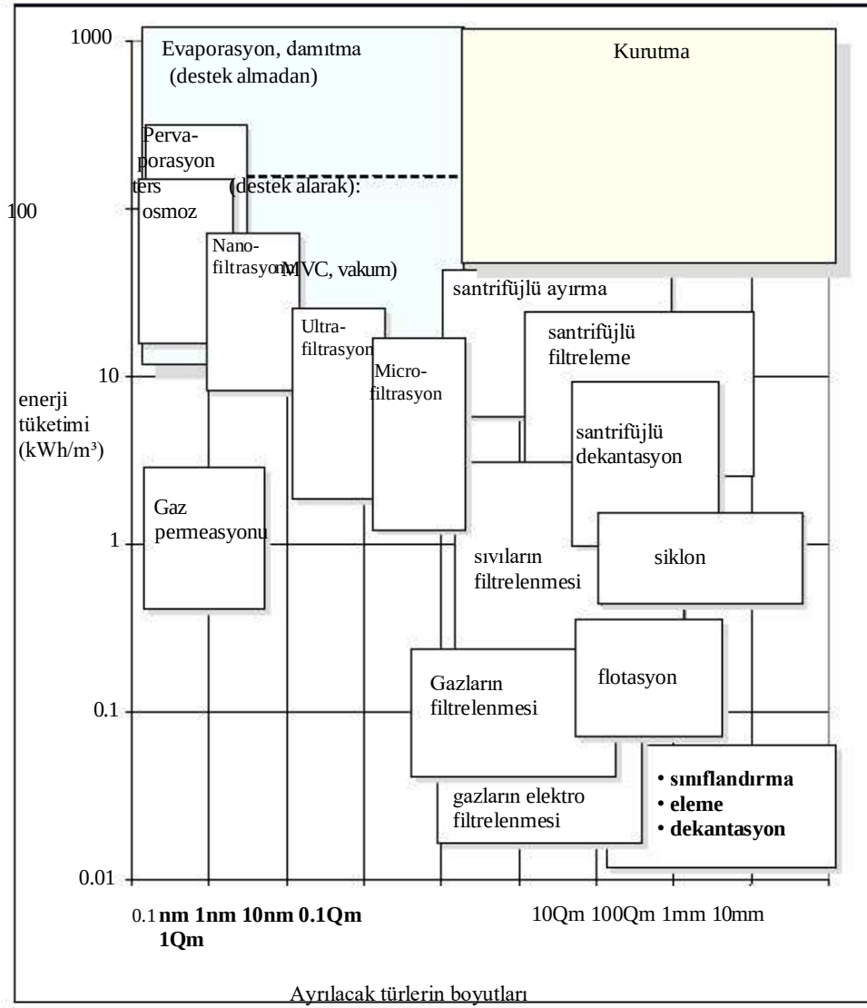
Şekil 3.44: bazı ayırma proseslerinin enerji tüketimi [248, ADEME, 2007]
