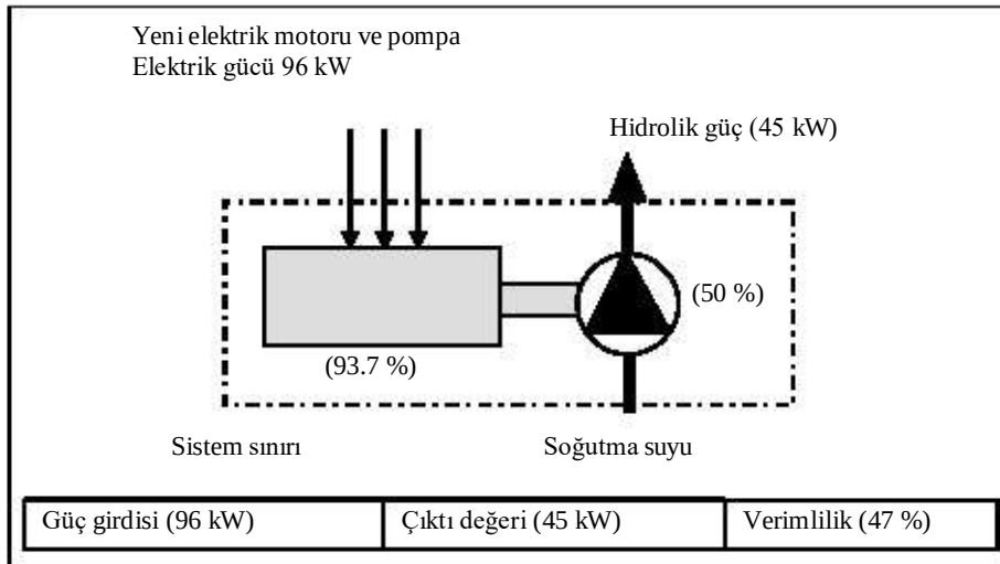
Şekil 1.12: sistem sınırı – yeni elektrik motoru ve eski pompa
