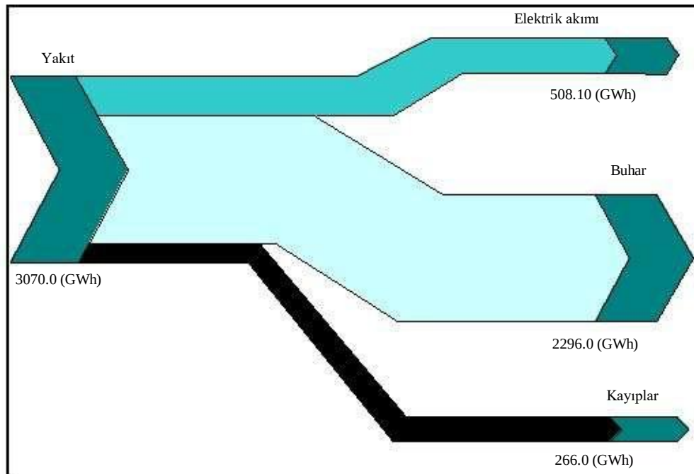
Şekil 2.7: Sankey diyagramı: tipik fabrikada yakıt ve kayıplar [186, UBA_AT]
