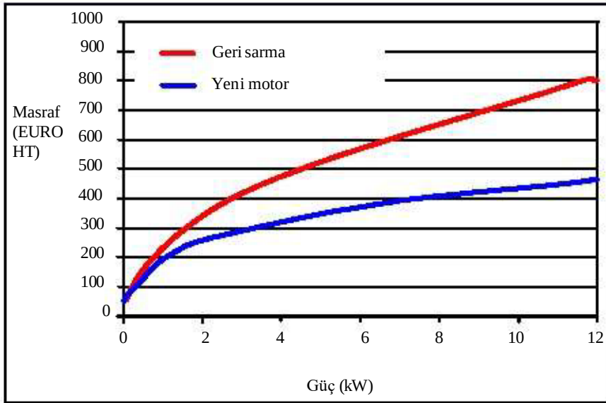
Şekil 3.29: geri sarma ile kıyaslandığında yeni motorun maliyeti
