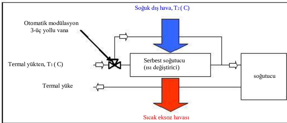
Şekil 3.43: serbest soğutma işleminin uygulanmasına ilişkin şema
