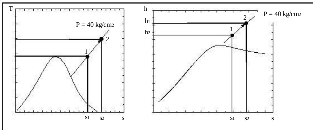
Şekil 7.6: örnek buhar ara ısıtma prosesinde T-s ve h-s diyagramları
