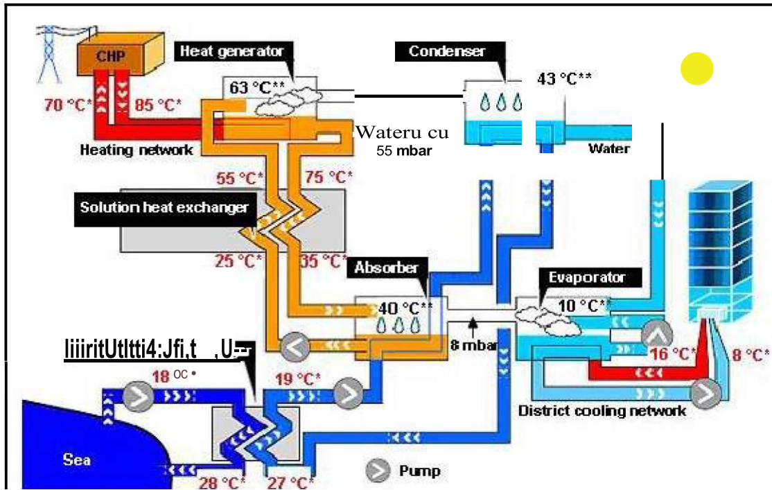
Şekil 3.20: serbest soğutma teknolojisiyle kış mevsiminde bölge soğutma [93, Tolonen, 2005]
