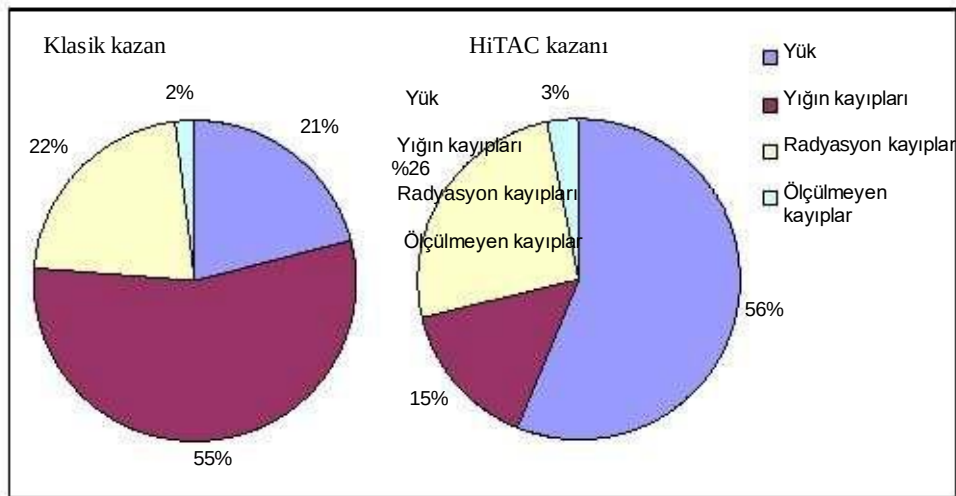
Şekil 5.2: Klasik ve HiTAC kazanları üzerinde yapılan araştırmalar sonucunda net ısı çıktısı sonuçları [17, Åsbländ, 2005]
