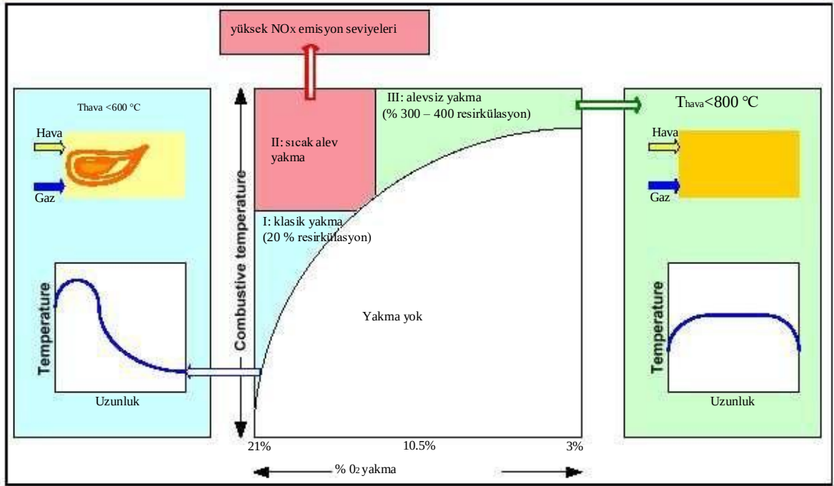
Şekil 5.3: Alevsiz yakma koşulları
