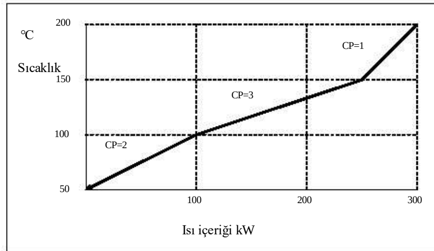
Şekil 2.12: Sıcak bileşen eğrisi
