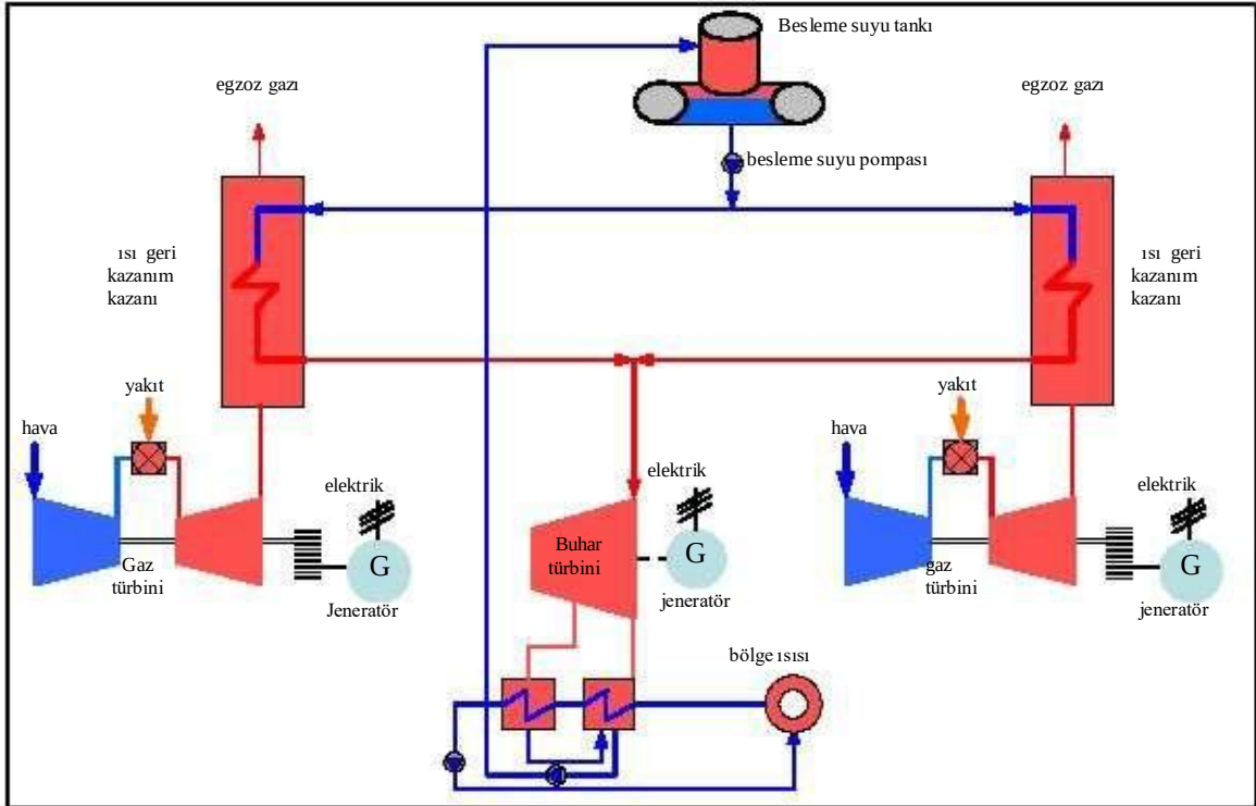
Şekil 3.15: kombine çevrim güç tesisi [65, Nuuttila, 2005]
