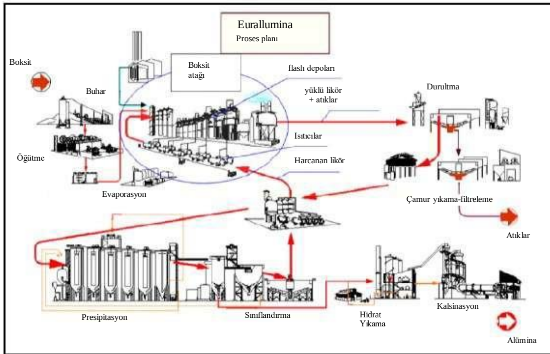
Şekil 7.14: Eurallumina alümina rafinerisinin proses planı [48, Teodosi, 2005]
