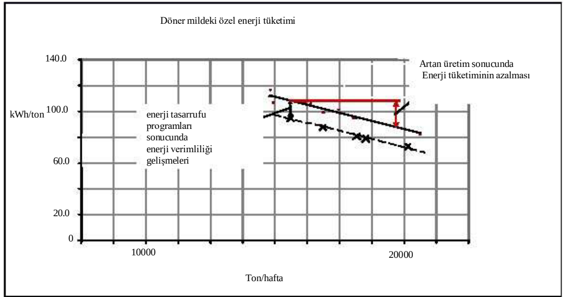
Şekil 7.13: Döner mildeki özel enerji tüketimindeki değişiklikler
