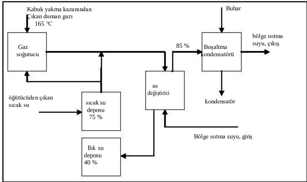
Şekil 7.16: Bölge ısıtma sistemine bağlı ısı geri kazanım sistemi [20, Åsbländ, 2005]
