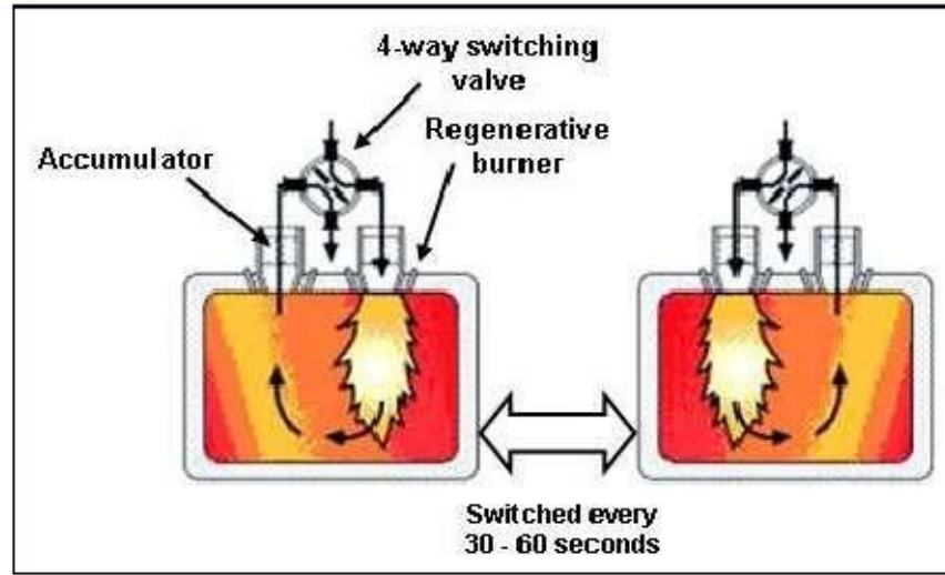
Şekil 3.3.yenileyici kazanların çalışma prensipleri [17, Åsbländ, 2005]
