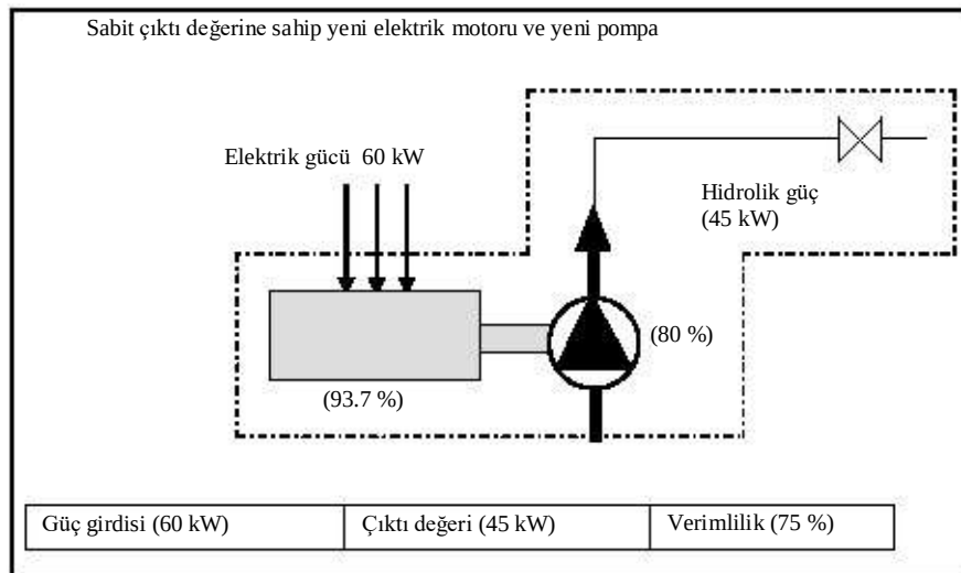
Şekil 1.14: sabit çıktı değerine sahip yeni elektrik motoru ve yeni pompa
