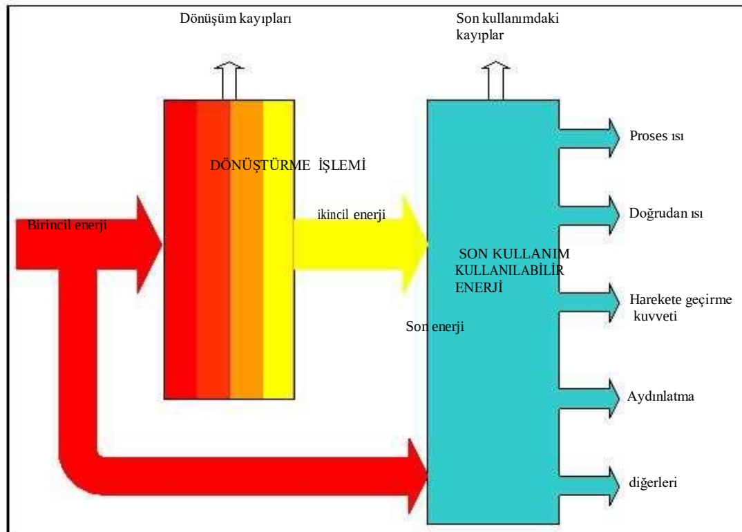
Şekil 1.6: Birincil, ikincil ve son enerjilerin tanımı [260, TWG, 2008]
