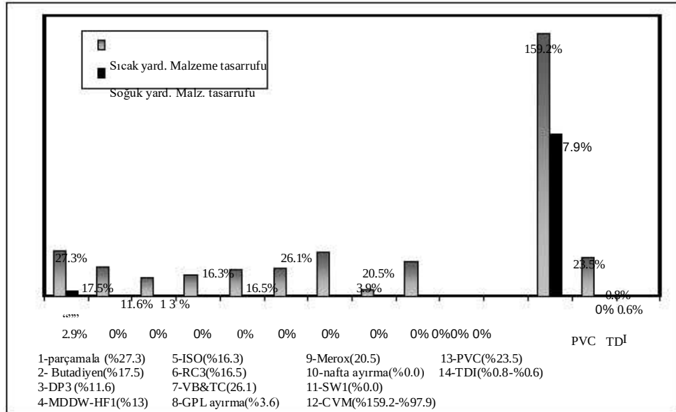
Şekil 2.16: Pinç metoduyla belirlenen enerji tasarrufları
