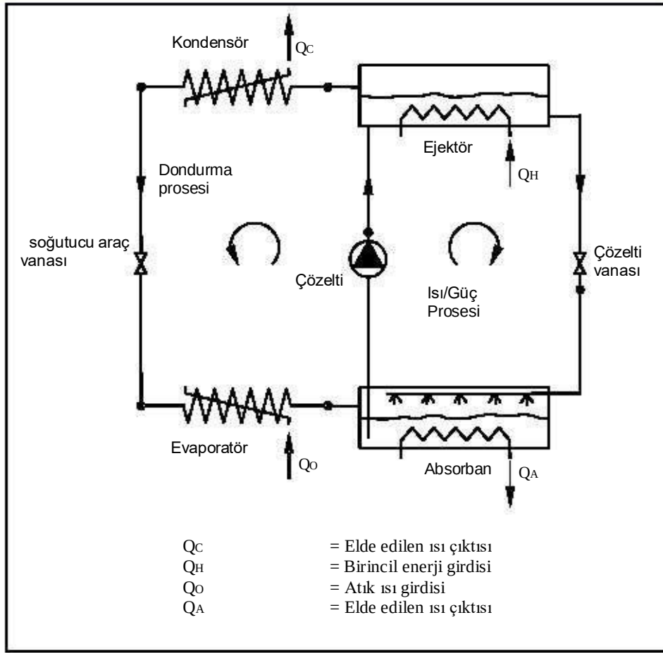
Şekil 3.9: Absorpsiyon ısı pompası [28, Berger, 2005]
