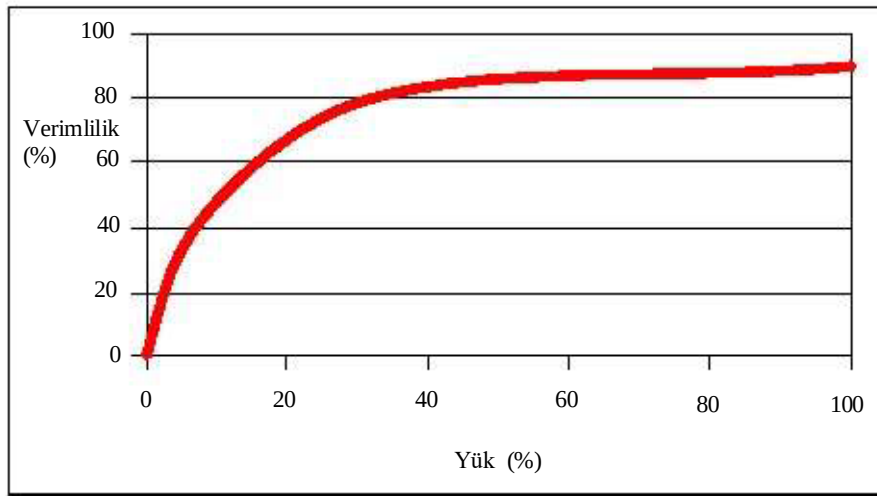
Şekil 3.28: elektrik motoru için verimlilik karşısında yük
