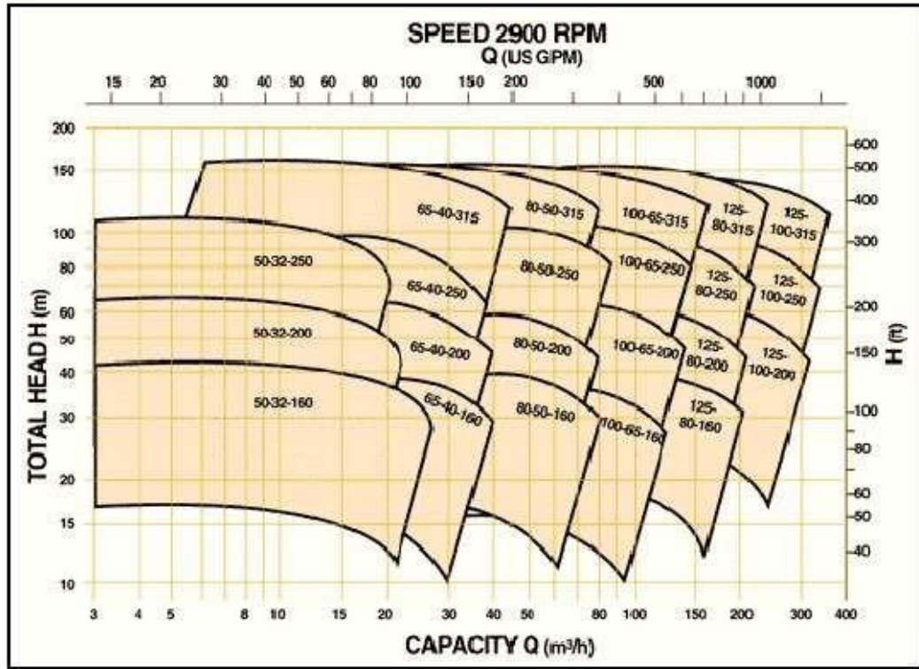
Şekil 3.36: pompa kapasitesi karşısında yük [199, TWG]
