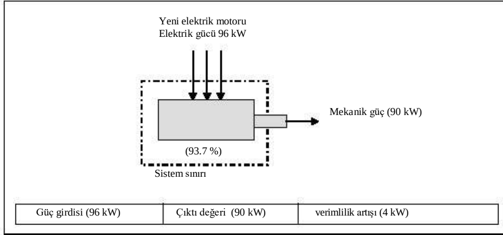
Şekil 1.11: sistem sınırı – yeni elektrik motoru
