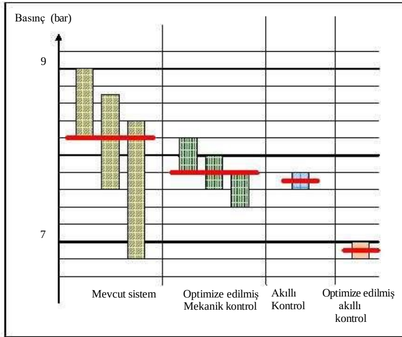
Şekil 3.34: farklı kompresör kontrol yöntemleri [28, Berger, 2005]
