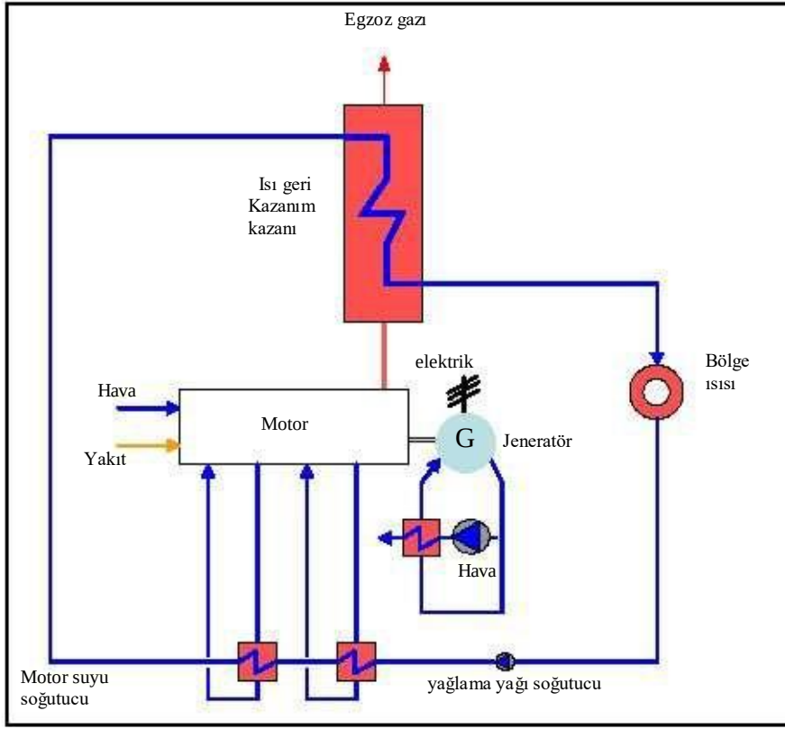
Şekil 3.16: içten yakmalı ya da yenileyici motor [65, Nuutila, 2005]
