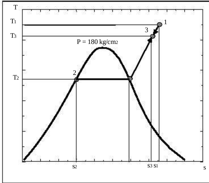
Şekil 7.9: örnek karıştırma prosesine ilişkin T-s diyagramı
