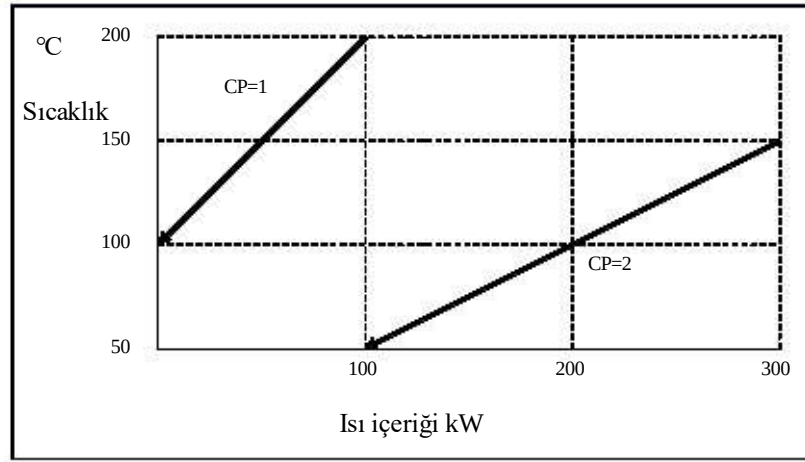
Şekil 2.11: iki sıcak buhar
