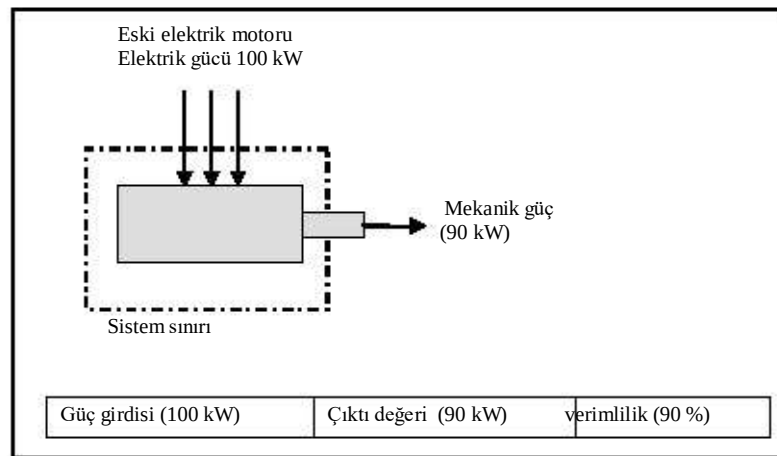
Şekil 1.10: sistem sınırı-eski elektrik motoru
