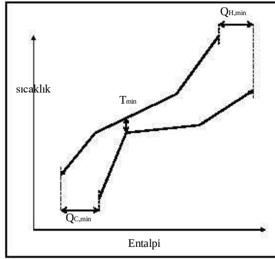
Şekil 2.13:Pinç ve enerji hedeflerini gösteren eğri
