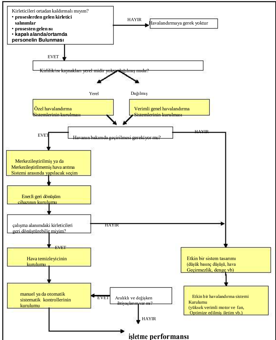
Şekil 3.42: havalandırma sistemlerinde enerji kullanımının optimize edilmesine ilişkin diyagram
