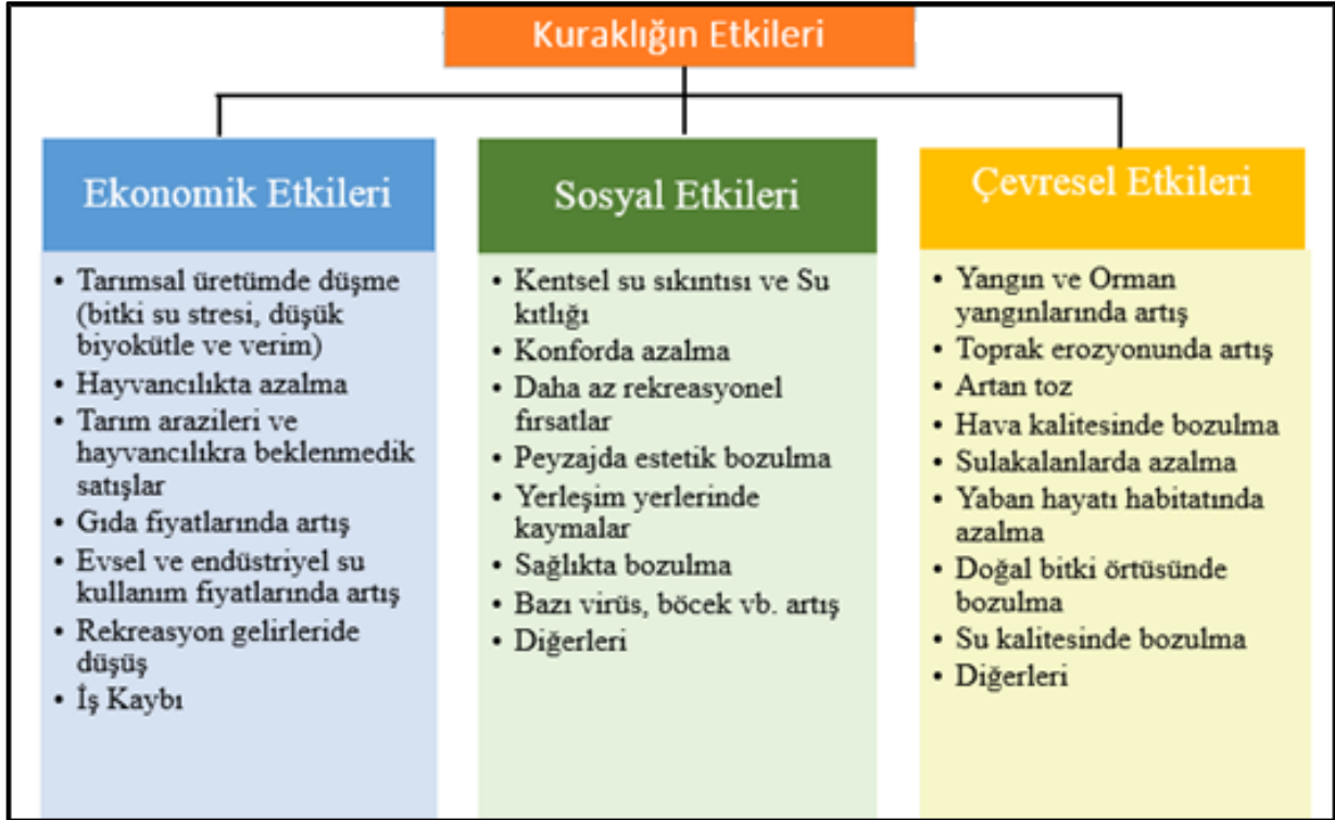
Şekil 37. Kuraklığın Etkileri
