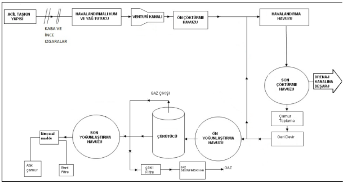
Şekil 3-7 Batı Adana Atıksu Arıtma Tesisi Proses Akım Şeması
