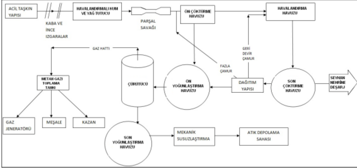
Şekil 3-10 Doğu Adana Atıksu Arıtma Tesisi Proses Akım Şeması
