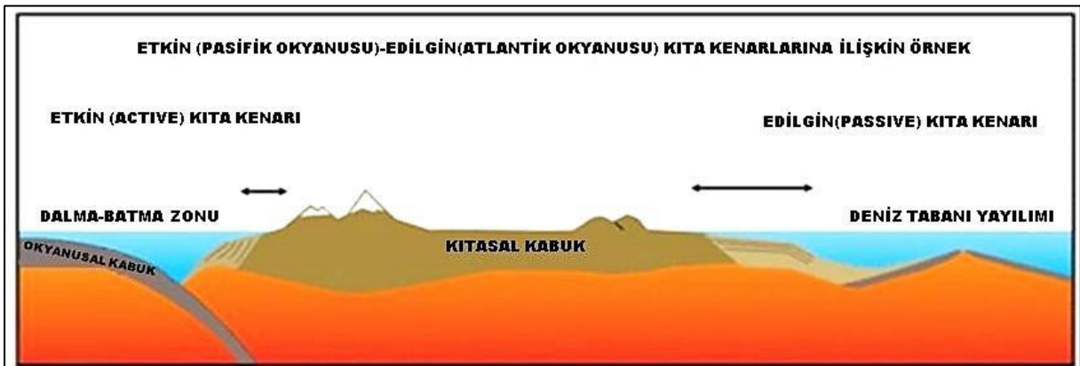
Şekil 3-9 Kıta kenarlarına iki güncel örnek: Pasifik okyanusu etkin (active) kıta kenarı ve Atlantik okyanusu edilgen (passive) kıta kenarı
