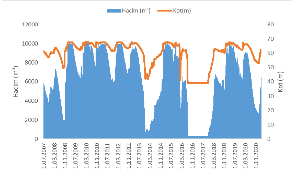
Şekil 10. Elmalı-II Barajı Kot-Hacim Grafiği (DSİ, 2021)
