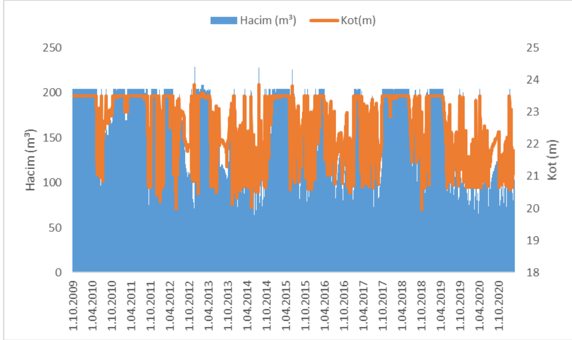
Şekil 13. Düzdere Barajı Kot-Hacim Grafiği (DSİ, 2021)
