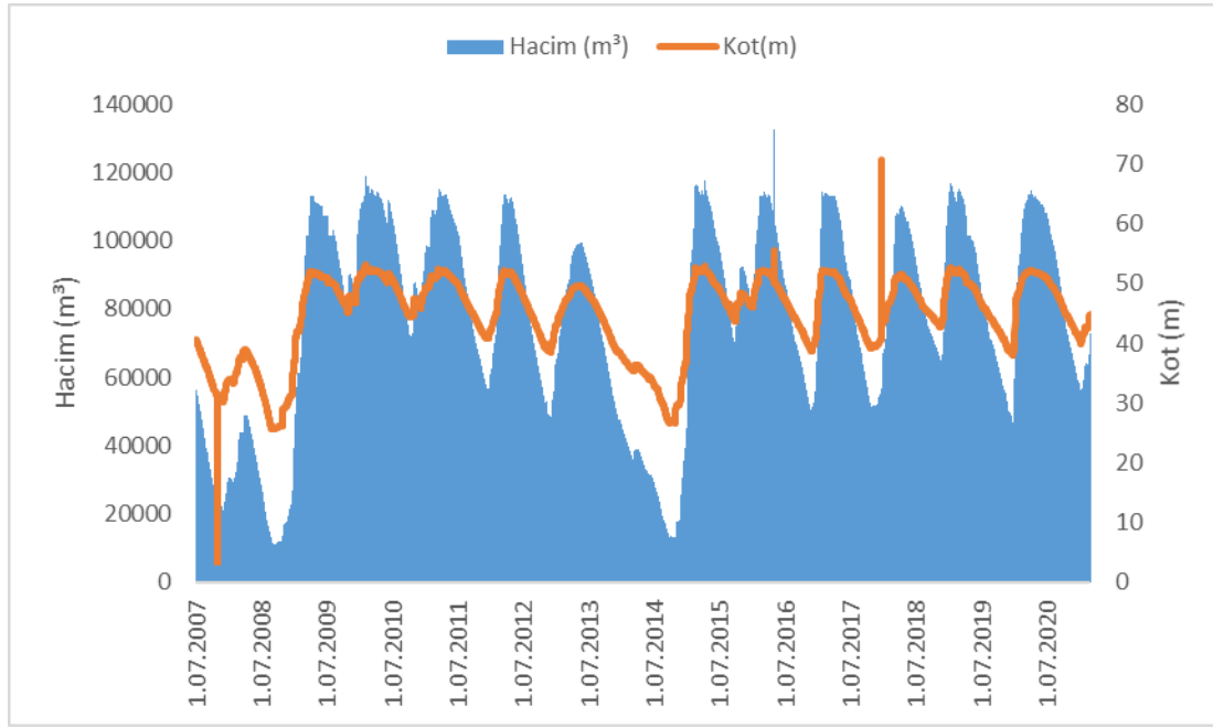
Şekil 8. Darlık Barajı Kot-Hacim Grafiği (DSİ, 2021)
