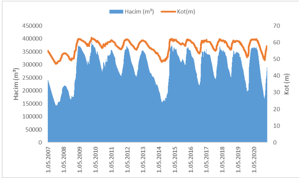
Şekil 9. Ömerli Barajı Kot-Hacim Grafiği (DSİ, 2021)
