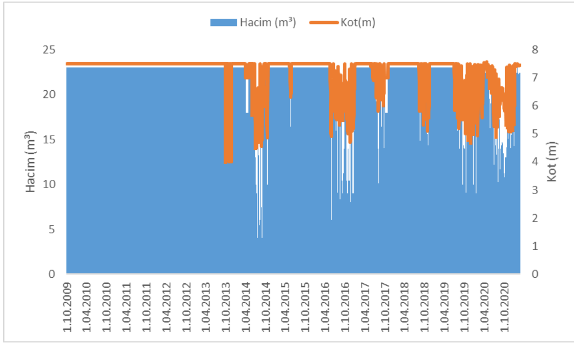
Şekil 14. Elmalıdere Barajı Kot-Hacim Grafiği (DSİ, 2021)
