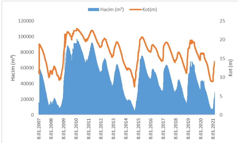
Şekil 12. Sazlıdere Barajı Kot-Hacim Grafiği (DSİ, 2021)
