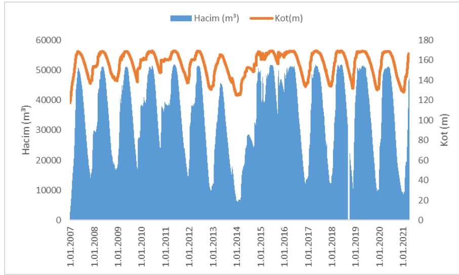
Şekil 11. Kirazdere (Yuvacık) Barajı Kot-Hacim Grafiği (DSİ, 2021)
