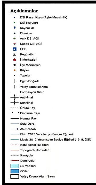
Şekil 3-9 Konya Havzası Hidrojeolojik Haritası (KKH SSTPH-MDAR)
