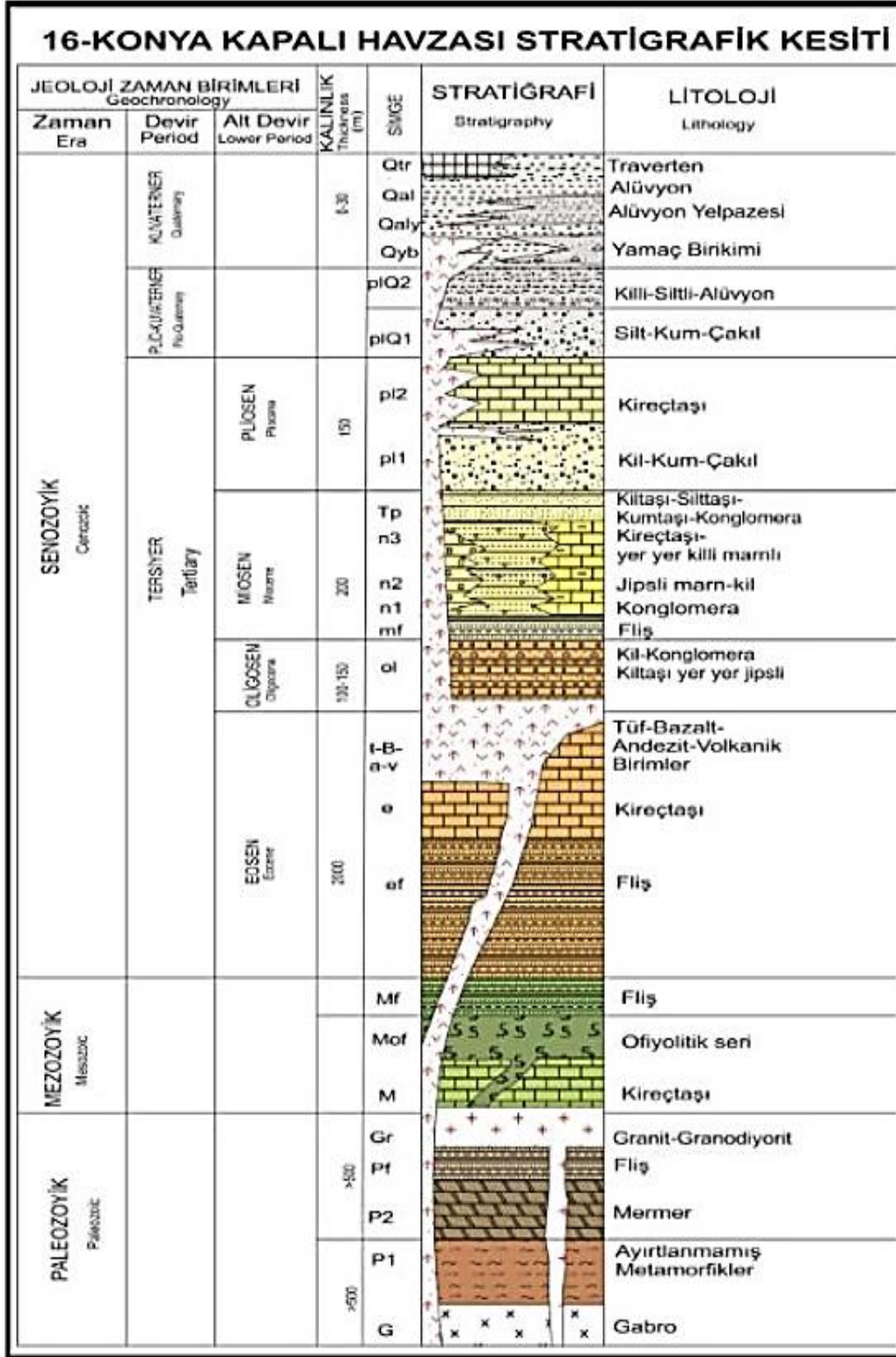
Şekil 3-2 Konya Havzası Genel Stratigrafik Kolon Kesiti
