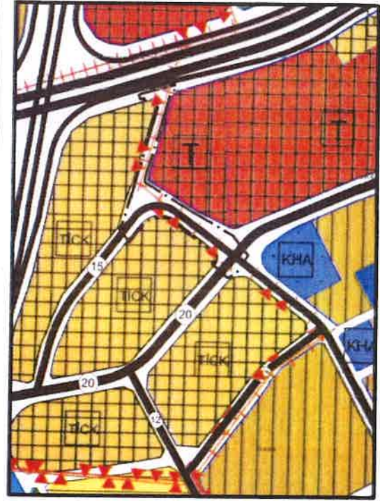
İtiraz Sonrası Düzeltilen Nazım İmar Planı Örneği
