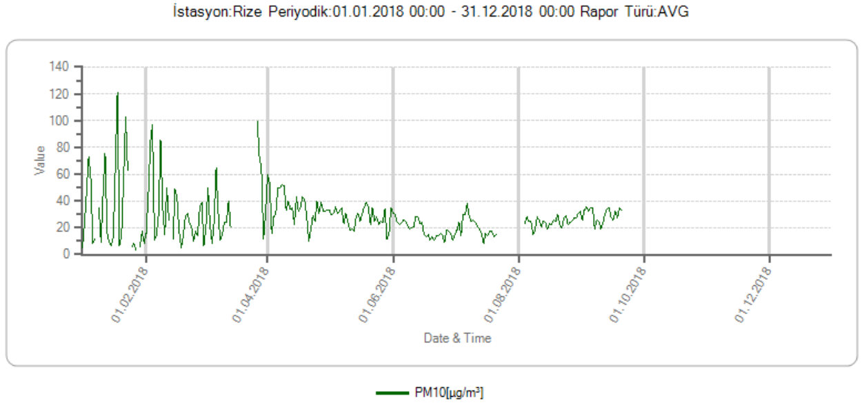
Grafik A.1 - Rize ilinde Rize istasyonu PM 10 parametresi günlük ortalama değer grafiği (laboratuvar.cevre.gov.tr, 2019)
