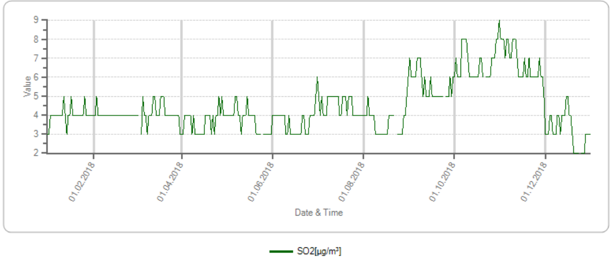
Grafik A.8 - Rize ilinde Ardeşen istasyonu SO 2 parametresi günlük ortalama değeri grafiği (laboratuvar.cevre.gov.tr, 2019)
