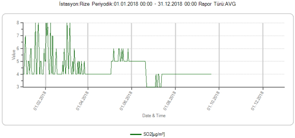
Grafik A.2 - Rize ilinde Rize istasyonu SO 2 parametresi günlük ortalama değer grafiği (laboratuvar.cevre.gov.tr, 2019)
