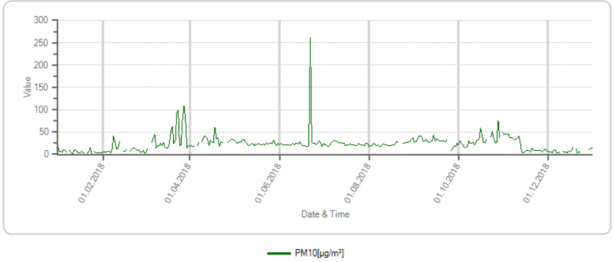
Grafik A.6 - Rize ilinde Ardeşen istasyonu PM 10 parametresi günlük ortalama değeri grafiği (laboratuvar.cevre.gov.tr, 2019)
