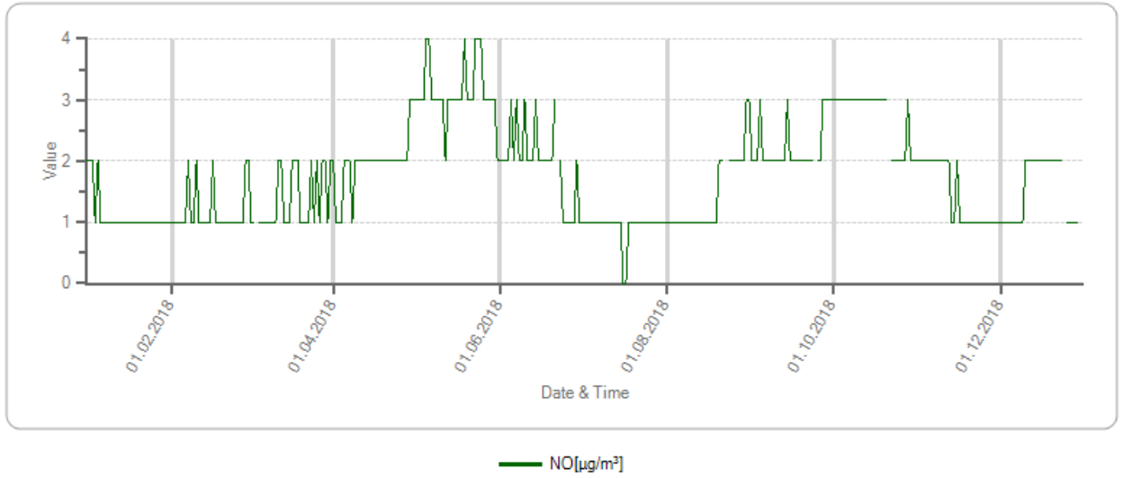
Grafik A.9 - Rize ilinde Ardeşen istasyonu NO parametresi günlük ortalama değeri grafiği (laboratuvar.cevre.gov.tr, 2019)
