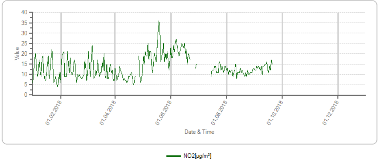
Grafik A.4 - Rize ilinde Rize istasyonu NO₂ parametresi günlük ortalama değer grafiği (laboratuvar.cevre.gov.tr, 2019)
