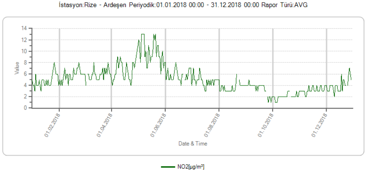
Grafik A.10 - Rize ilinde Ardeşen istasyonu NO 2 parametresi günlük ortalama değer grafiği (laboratuvar.cevre.gov.tr, 2019)
