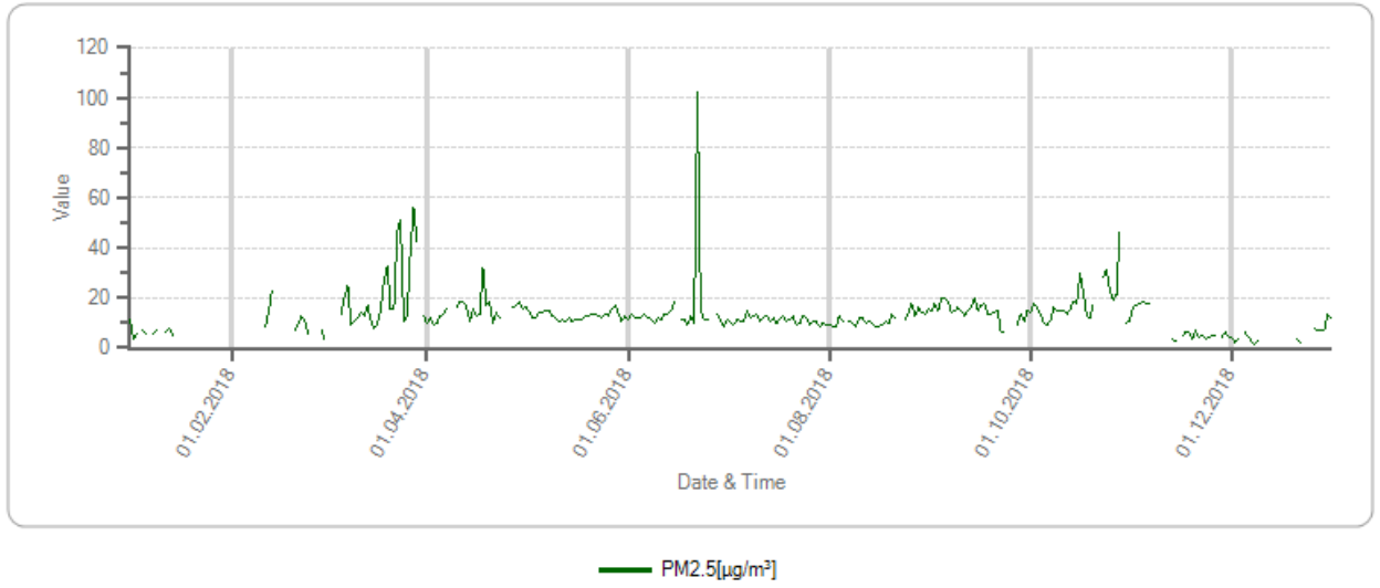
Grafik A.7 - Rize ilinde Ardeşen istasyonu PM 2,5 parametresi günlük ortalama değeri grafiği (laboratuvar.cevre.gov.tr, 2019)
