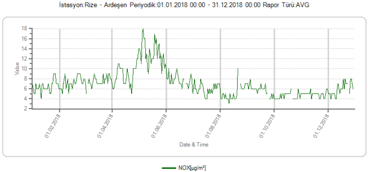
Grafik A.11 - Rize ilinde Ardeşen istasyonu NO x parametresi günlük ortalama değer grafiği (laboratuvar.cevre.gov.tr, 2019)
