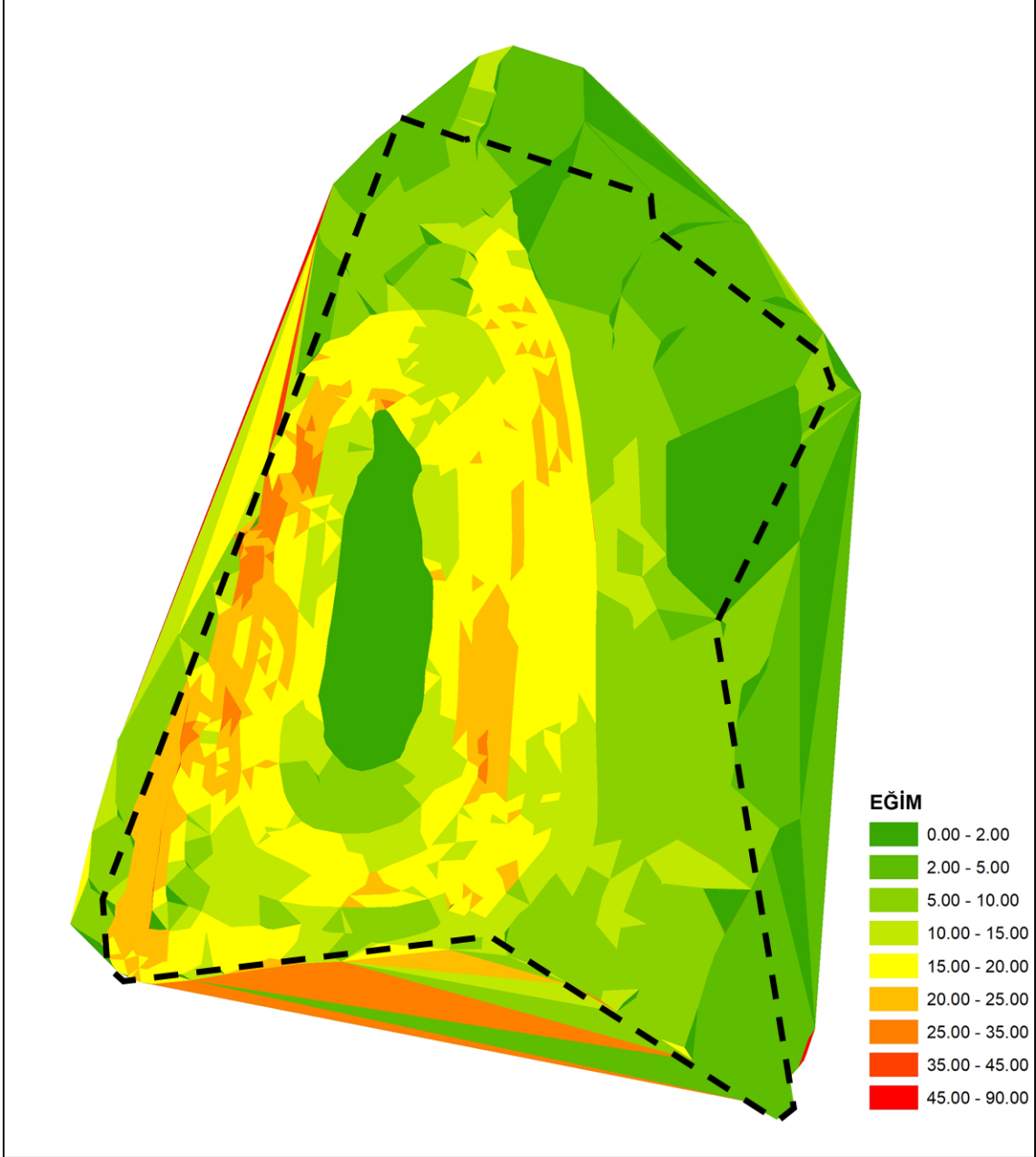
Şekil 34 Eğim Analizi
