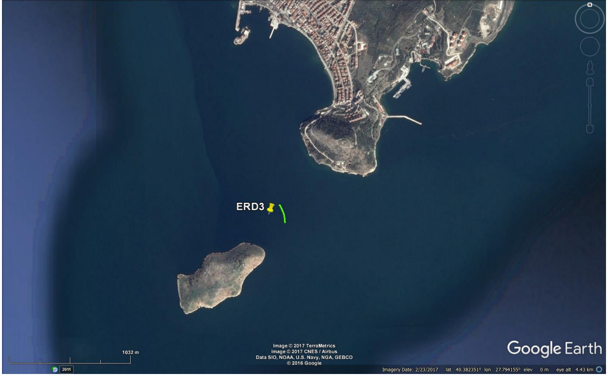
Şekil 48. 12 Nisan 2017 tarihinde ERD3’de bırakılan yüzeğin izlediği yol.
