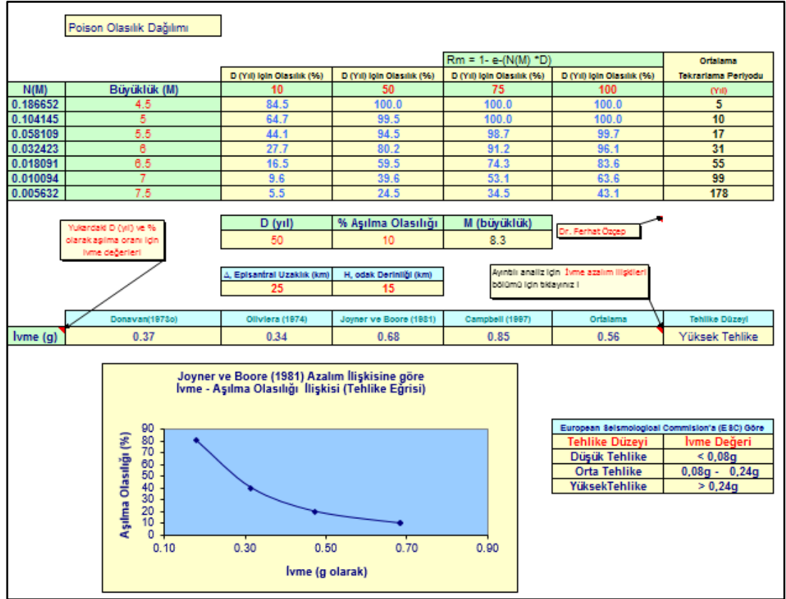
Şekil 28: 1. Bölge Poisson olasılık dağılımına göre deprem risk analizi ( M_s \geq 4,5 )
