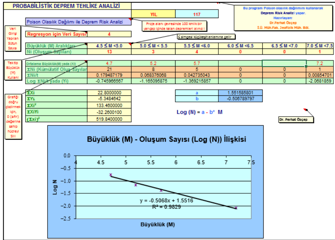
Şekil 27: 1. Bölge Probabilistik Deprem Tehlike Analizi
