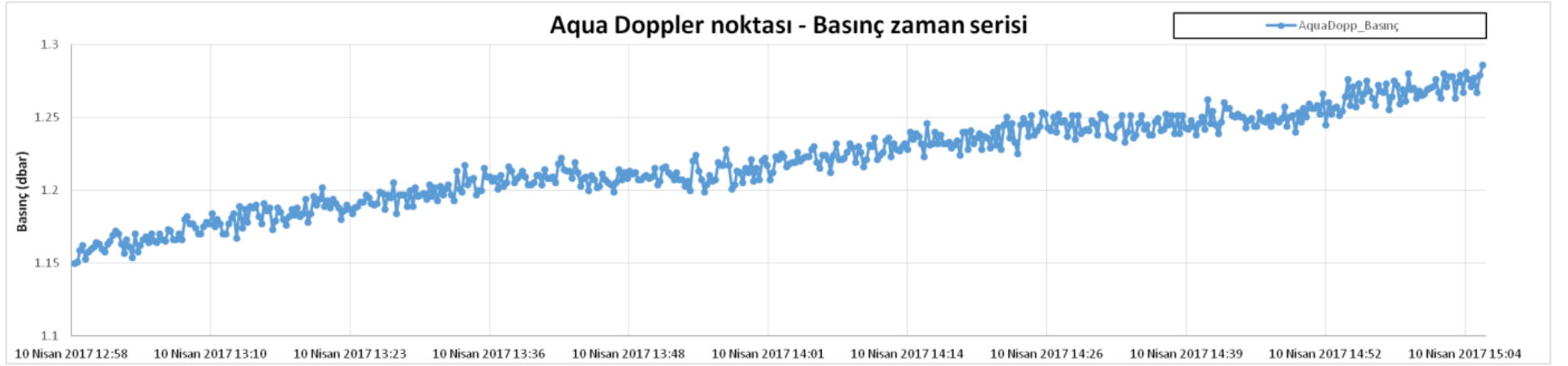
Şekil 56. AquaDoppler noktasında Aqua Doppler tarafından yüzeyden yaklaşık 1 m aşağıda kaydedilen (a) akıntı hızları ve yönleri, (b) basınç değişimi
