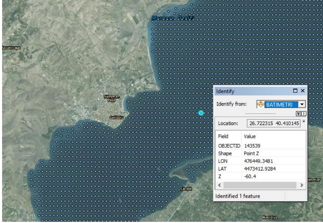
Şekil 10. Çanakkale Boğazı Marmara Denizi Girişi Batimetri Noktaları
