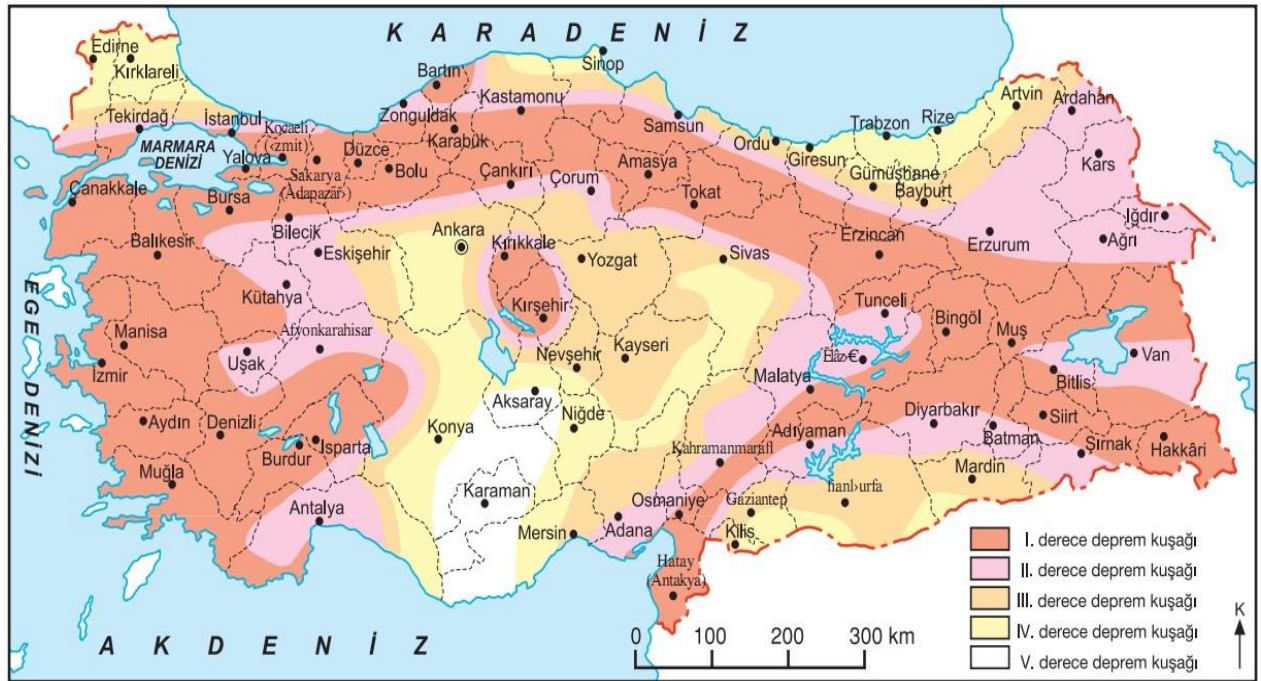
Şekil 24 Türkiye Deprem Bölgeleri Haritası
