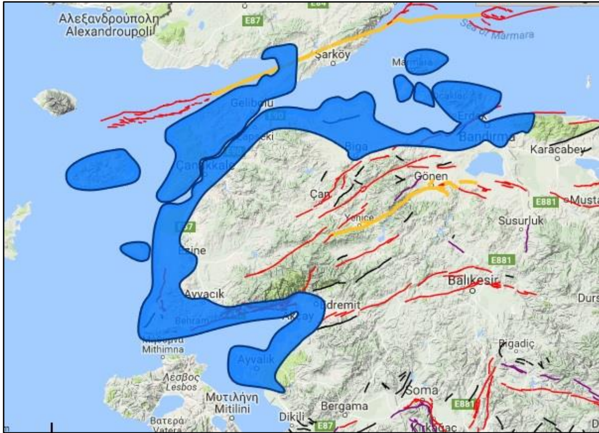
Şekil 25. Çanakkale-Balıkesir Planlama Bölgesine Ait Diri Fay Haritası
