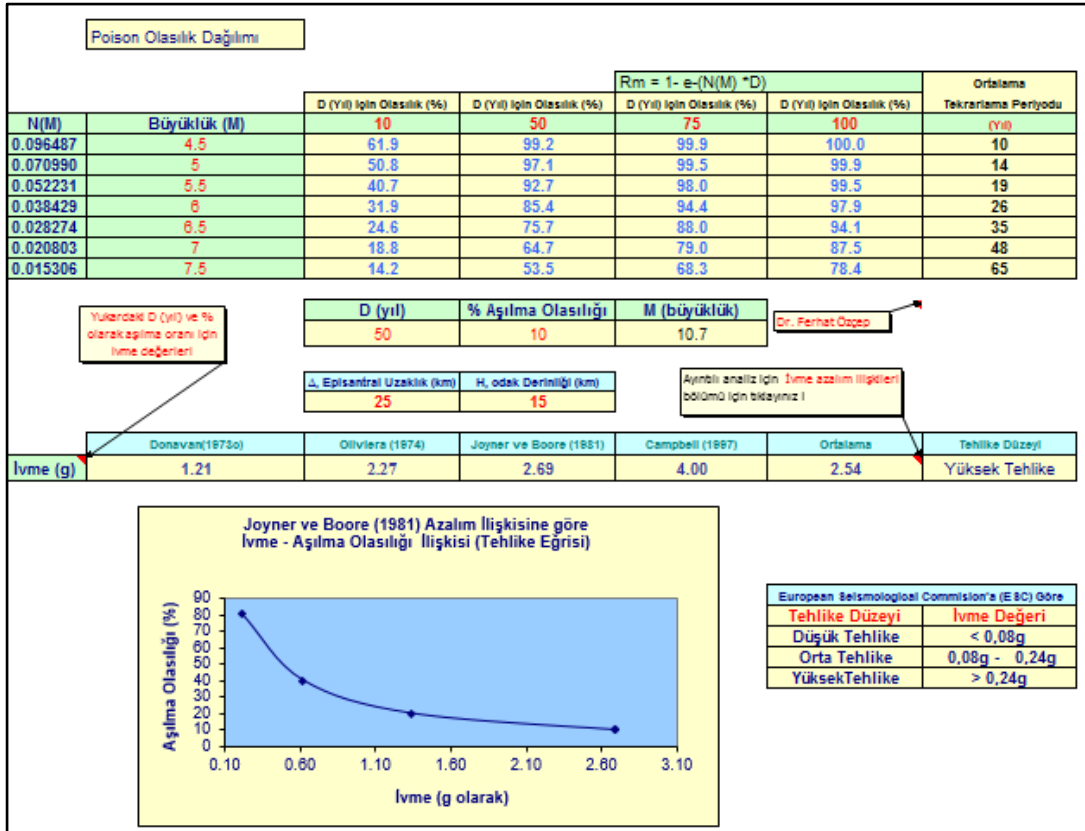
Şekil 30: 2. Bölge Poisson olasılık dağılımına göre deprem risk analizi ( M_s \geq 4,5 )
