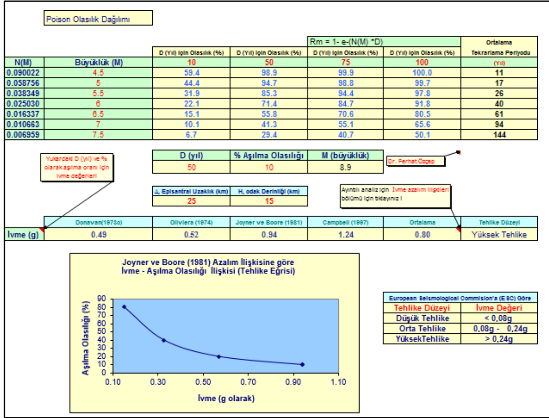
Şekil 36: 5. Bölgeye ait Poisson olasılık dağılımına göre deprem risk analizi ( M_s \geq 4,5 )
