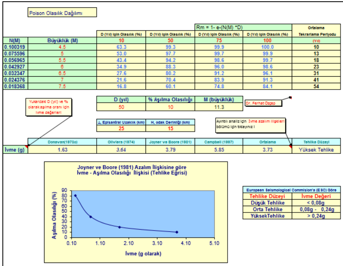
Şekil 32: 3. Bölge Poisson olasılık dağılımına göre deprem risk analizi (Ms≥4,5)
