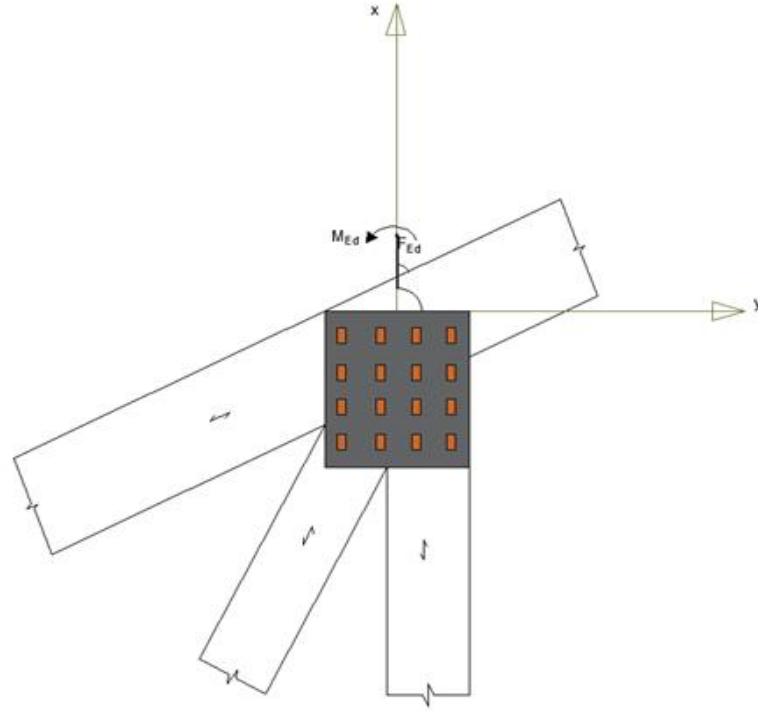
Şekil 6.6 Plaka geometrisi
