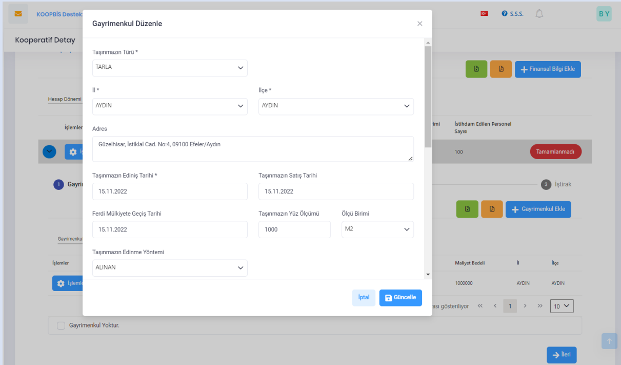
Şekil 8: Gayrimenkul Düzenle
