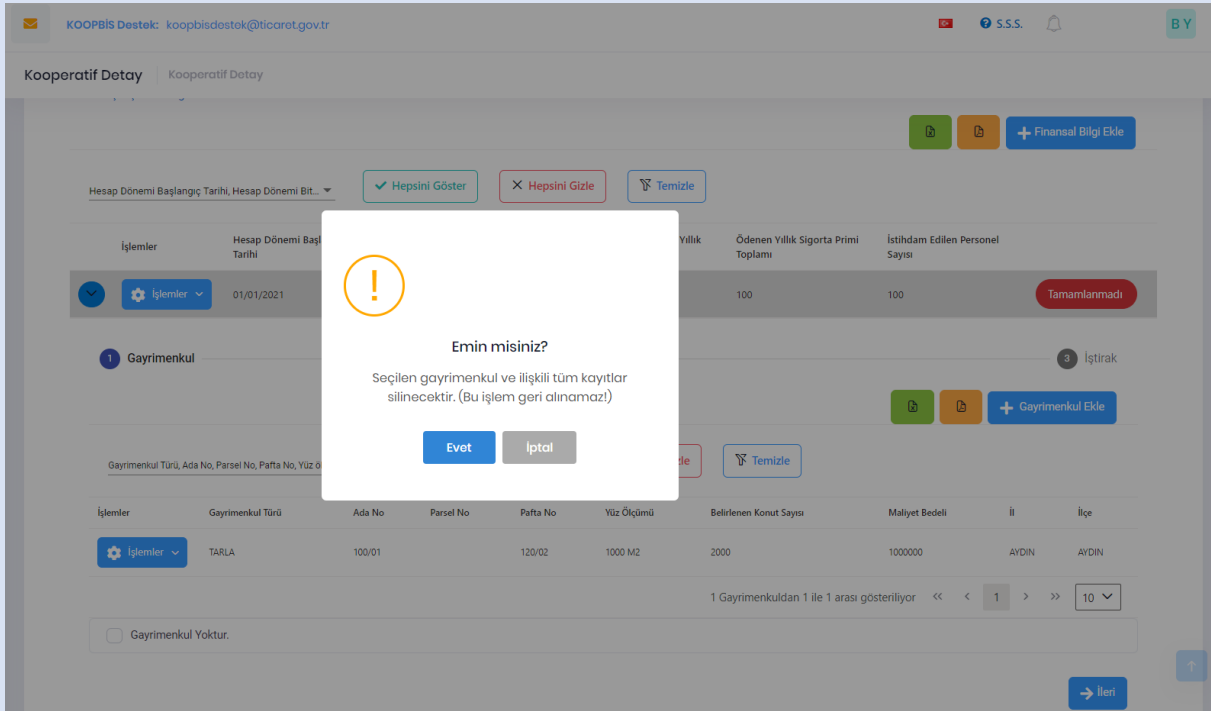
Şekil 9: Gayrimenkul Sil
