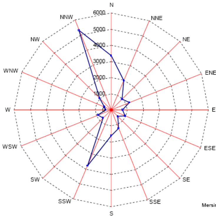
MERSİN UZUN YILLARA AİT RÜZGAR DİYAGRAMI ( RASAT SÜRESİ 23 YIL )
