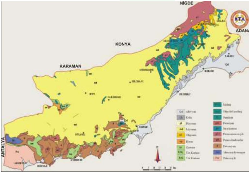
Harita 6: Mersin İli Jeoloji Haritası
