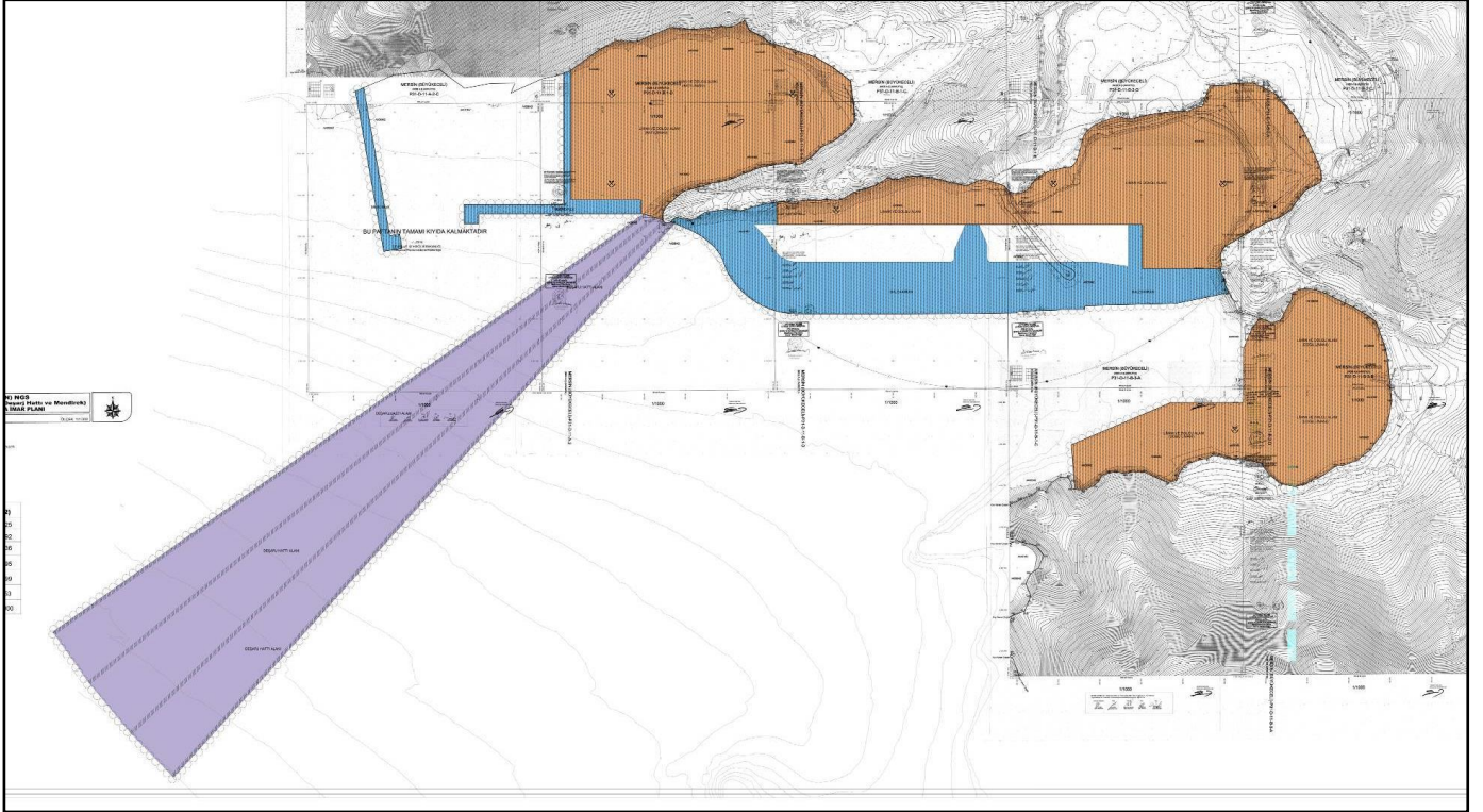
HARİTA 19: 10/02/2015 ONAY TARİHLİ AKKUYU NÜKLEER GÜÇ SANTRALİ LİMAN VE DOLGU ALANI 1/1000 ÖLÇEKLİ UYGULAMA İMAR PLANI
