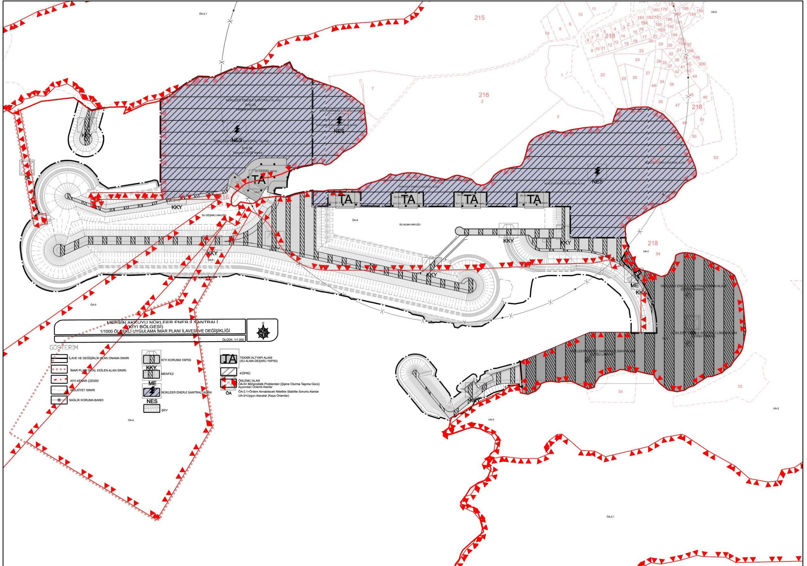
HARİTA 25: MERSİN AKKUYU NÜKLEER ENERJİ SANTRALİ (KIYI BÖLGESİ) UYGULAMA İMAR PLANI İLAVESİ VE DEĞİŞİKLİĞİ
