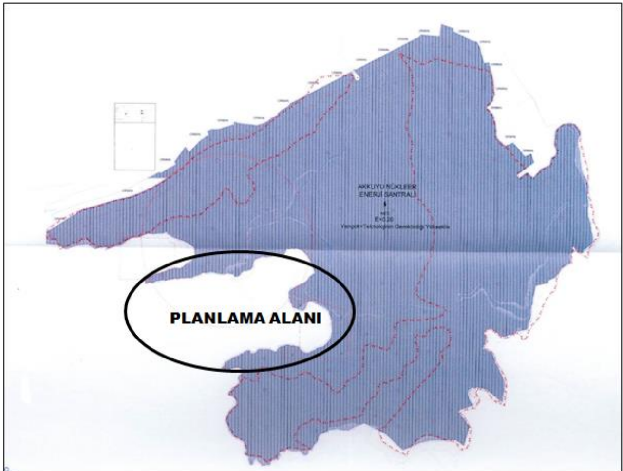
HARİTA 18: 22/03/2017 ONAY TARİHLİ AKKUYU NÜKLEER ENERJİ SANTRALİ (NES) 1/1000 ÖLÇEKLİ UYGULAMA İMAR PLANI
