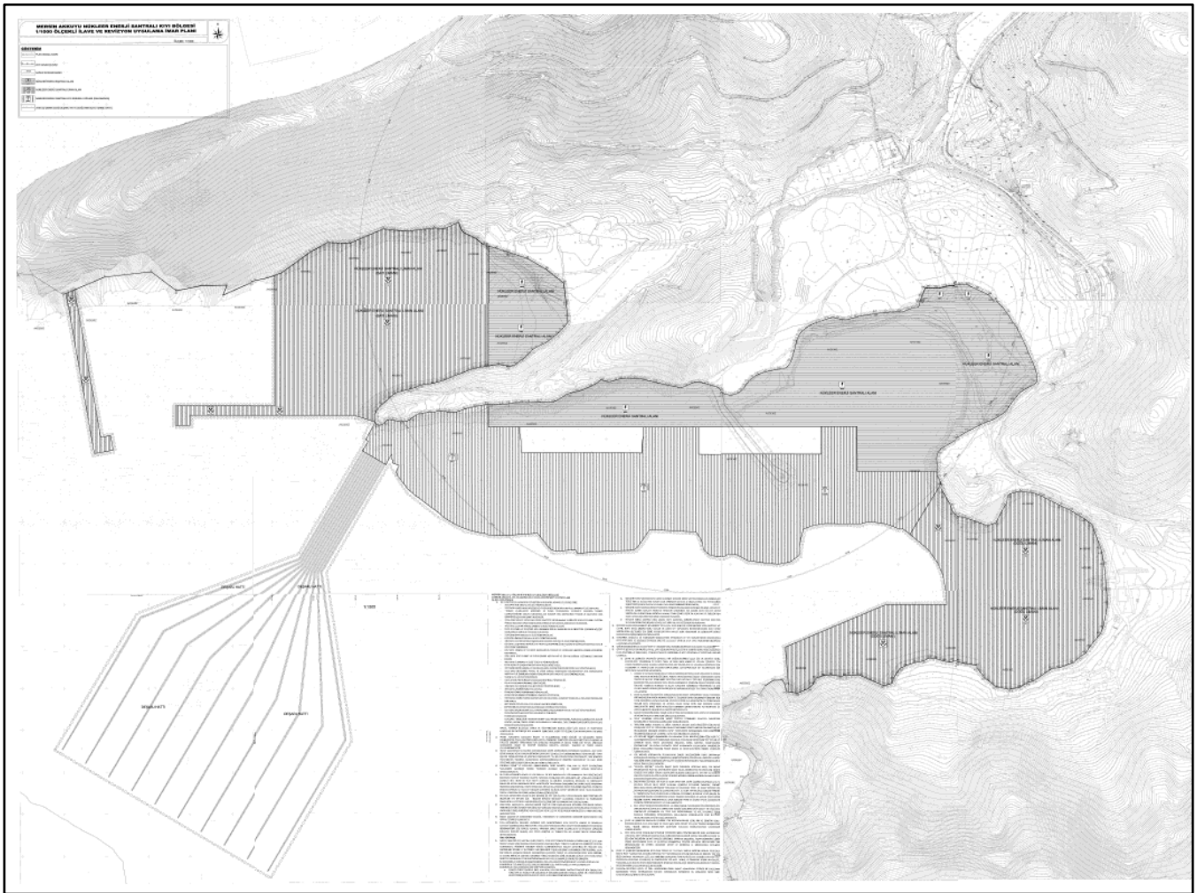
HARİTA 20: 13/03/2017 ONAY TARİHLİ MERSİN AKKUYU NÜKLEER ENERJİ SANTRALİ KIYI BÖLGESİ 1/1000 ÖLÇEKLİ İLAVE VE REVİZYON UYGULAMA İMAR PLANI
