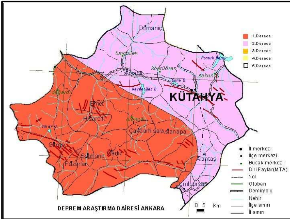
Şekil 4: Parsel alanına ait deprem bölgeleri haritası
