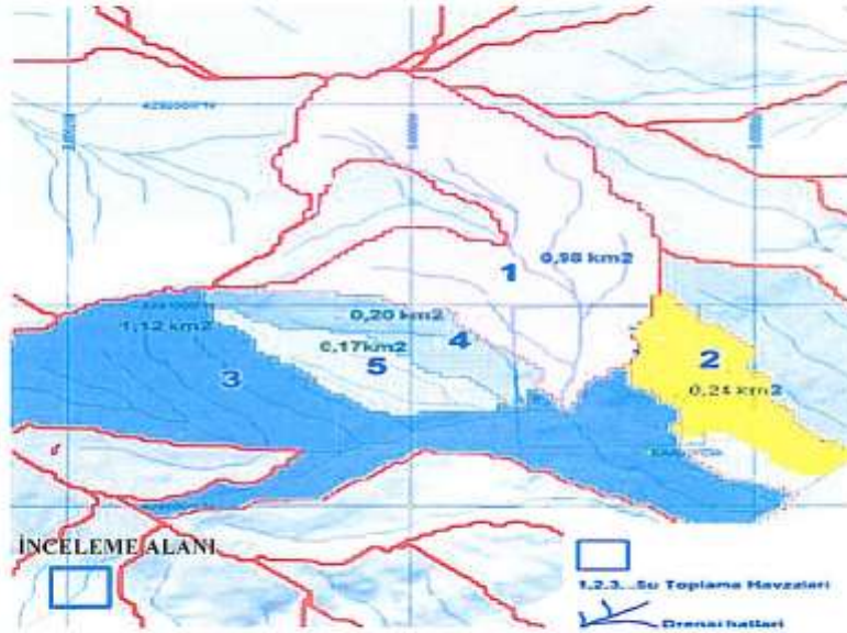
Şekil 12: İnceleme Alanı ve Yakın Civarının Drenaj Ağı ve Su Toplama Havzaları Haritası. (M.K. Tüfekçi ve G.S. Çolak, 2011 Tarihinde Üretilmiştir.)
