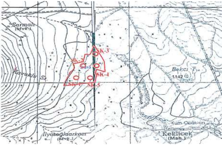
Şekil 11: Sondaj Kuyuları Yerleşim Planı
