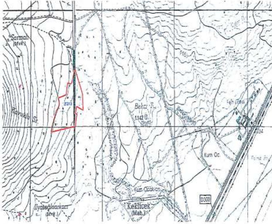
Şekil 3: İnceleme Alanın 1/25000 Topoğrafik Haritası
