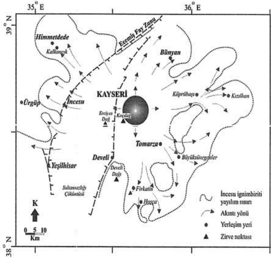
Şekil 6: İncesu İğnimbiritinin Alan Dağılım Haritası (Schumacher et al. 2004'den)
