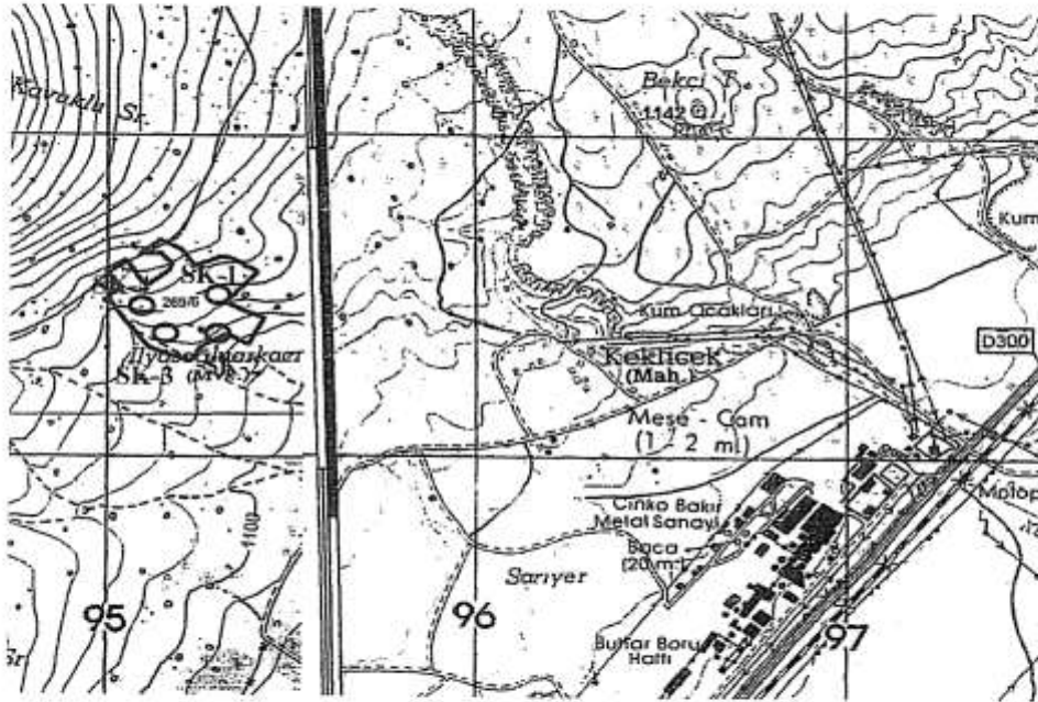
Şekil 11: Sondaj Kuyuları Yerleşim Planı
