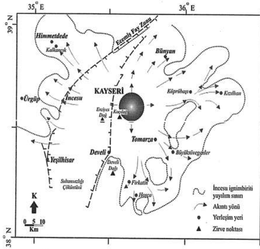
Şekil 6: İncesu İgnimbritinin Alan Dağılım Haritası (Schumacher et al. 2004'den)
