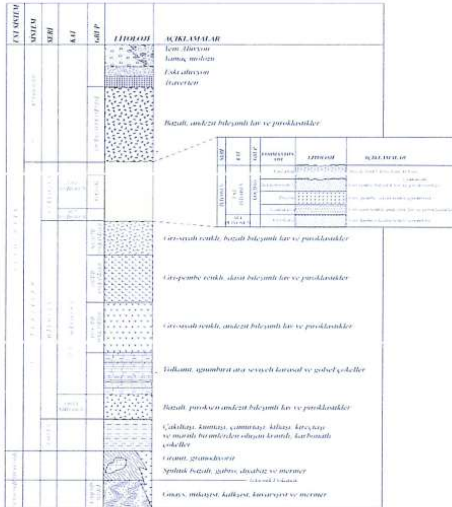
Şekil 8: Kayseri ve Çevresinin Genelleştirilmiş Stratigrafik Dikme Kesiti ve İncesü İlgimbiritinin Bu Kesitteki Yeri. (Dönmez vd. 2005'den değiştirilerek alınmıştır.)
