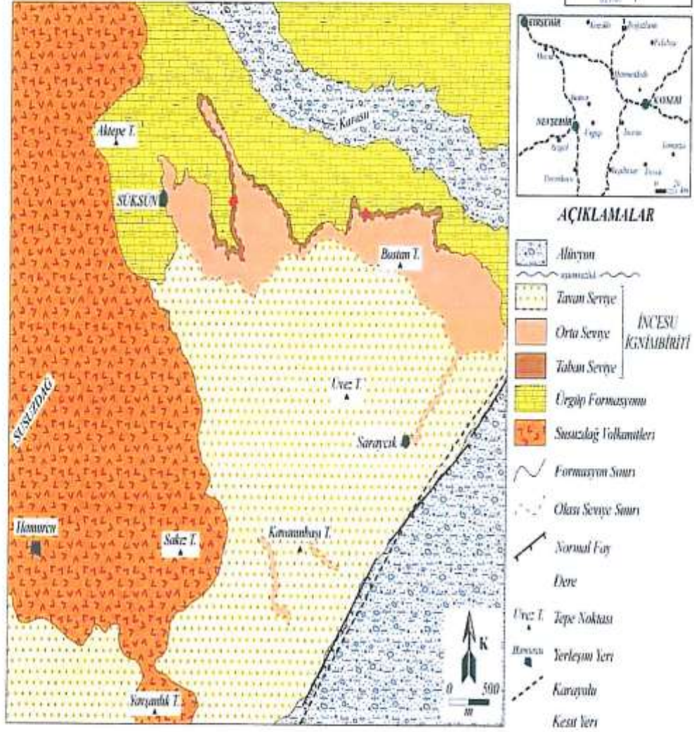
Şekil 7: İnceleme Alanı ve Yakın Cıvırı Jeolojı Harıtası
