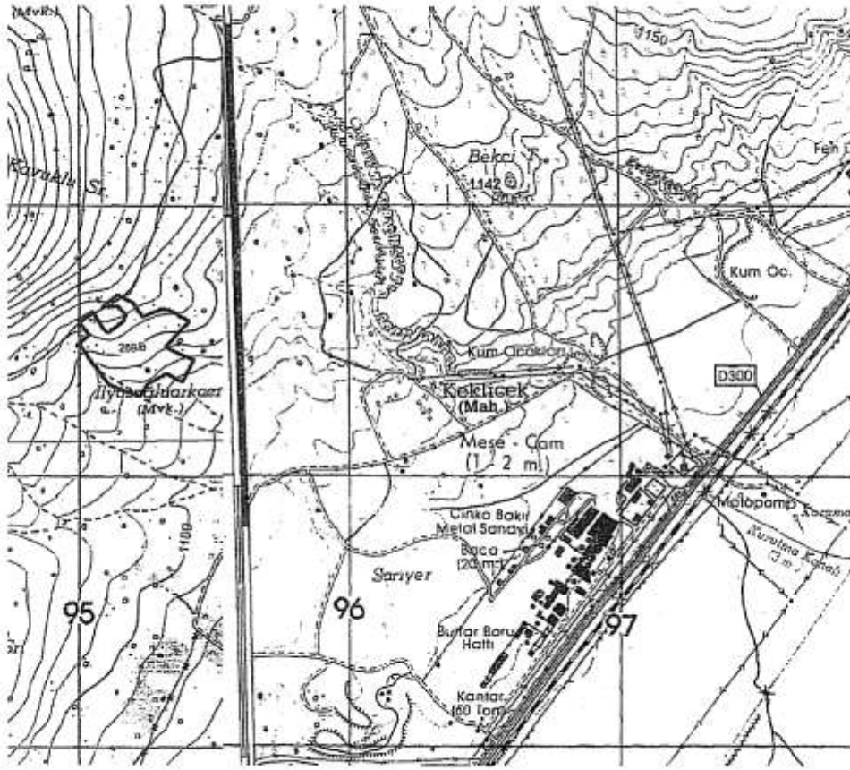
Şekil 3: İnceleme Alanın 1/25000 Topoğrafik Haritası
