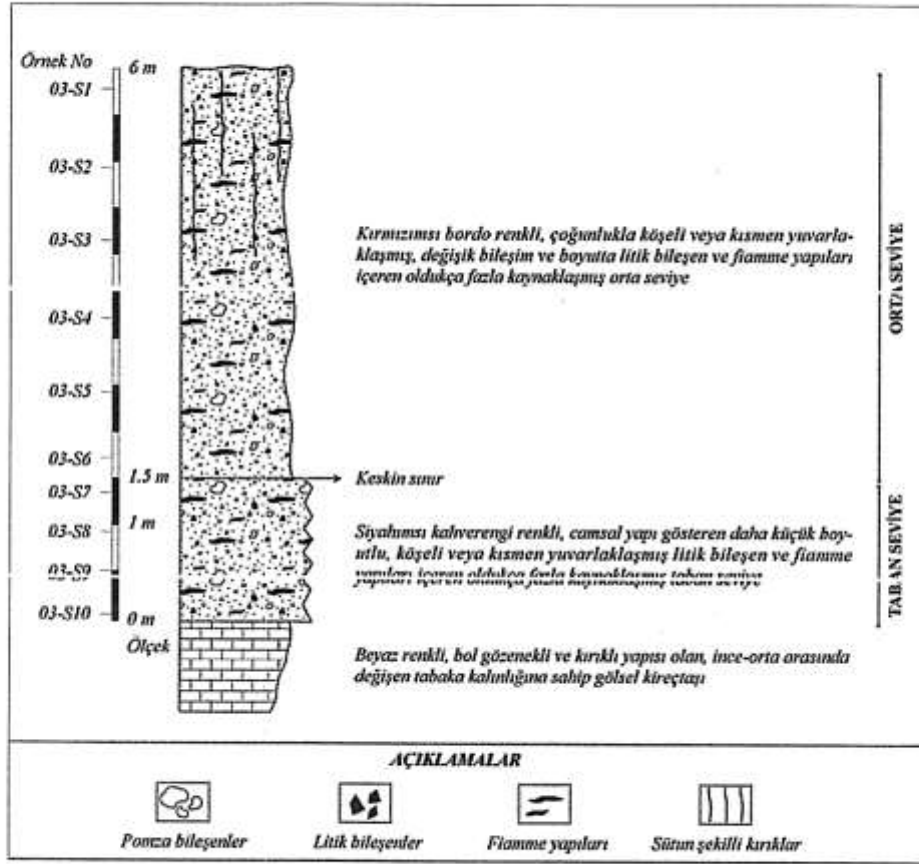
Şekil 5: İncesu İgnimbiritinin Hamurcu Köyü ve çevresindeki kolon kesiti
