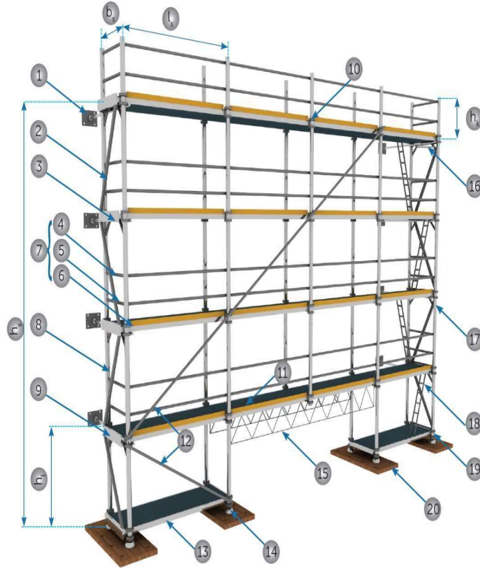
Şekil 10 Dış Cephe İskele Örnek Görseli
