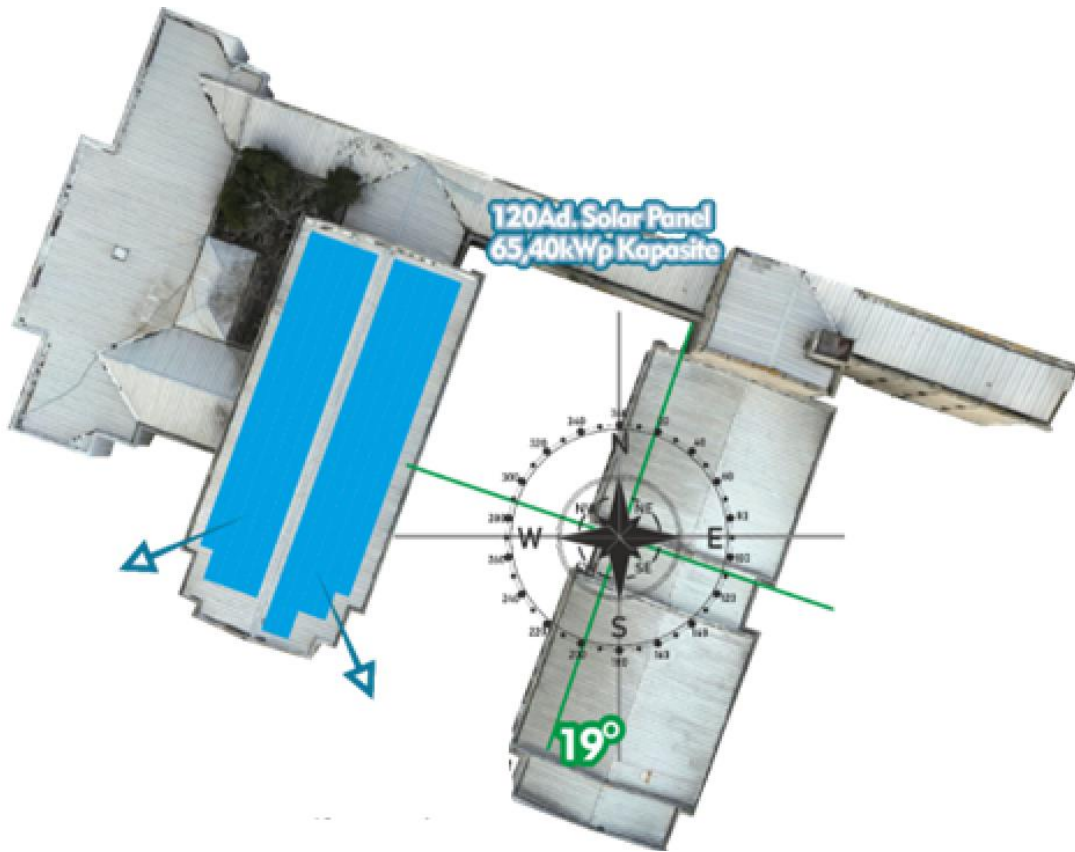
Şekil 12 Öğrenci Kültür Merkezi Çatı Üstü PV Yerleşim Planı
