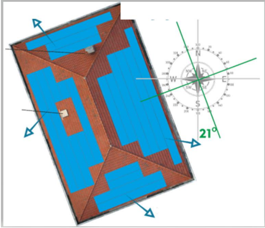
Şekil 11 Rektörlük İdari Binası Çatı Üstü PV Yerleşim Planı
