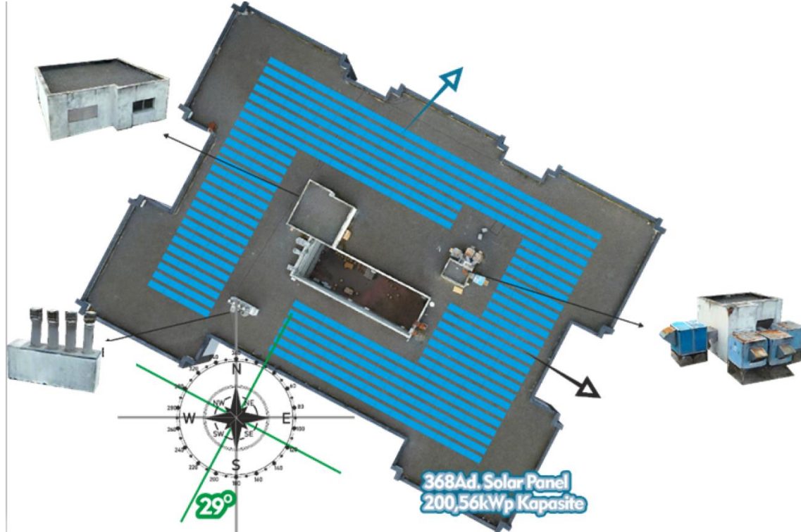
Şekil 12 Öğrenci Kültür Merkezi Çatı Üstü PV Yerleşim Planı
