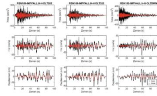
Şekil E. 3-12. Kayın-1 için ivme, hız ve deplasman zaman serileri (2475 s).
