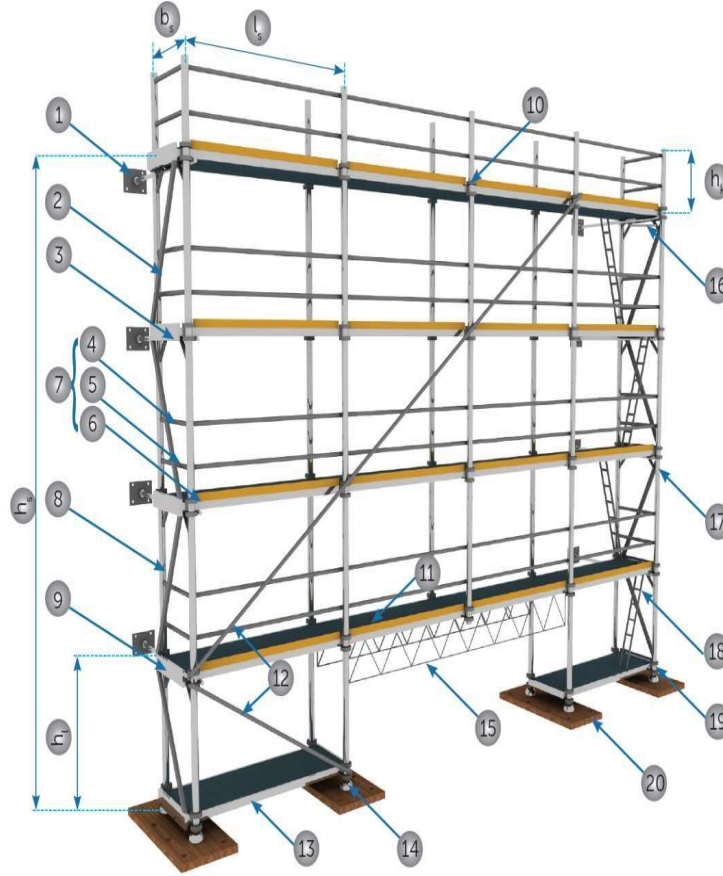
Şekil 15 Dış Cephe İskele Örnek Görseli
