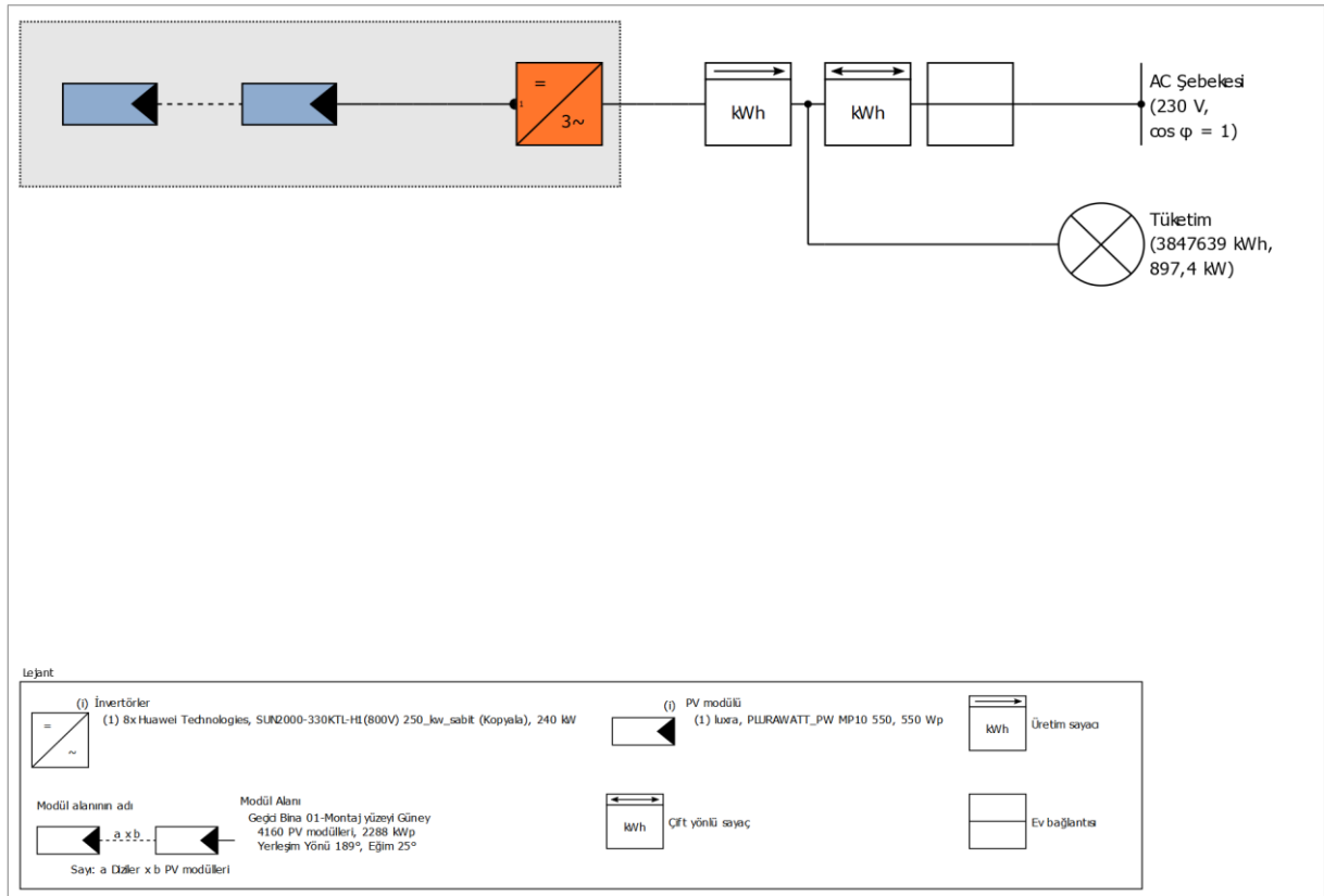
Şekil 3 2 Şematik Diyagram
