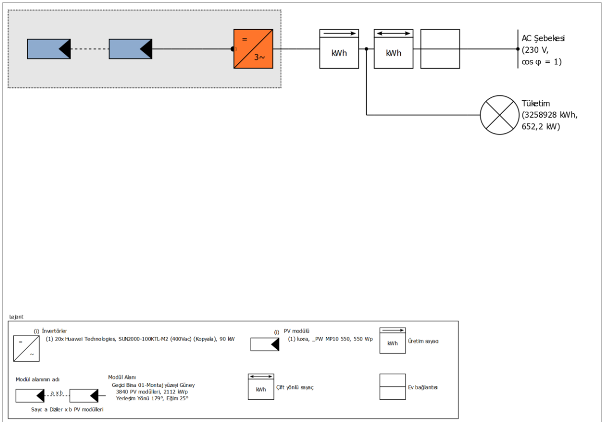
Şekil 3 2 Şematik Diyagram
