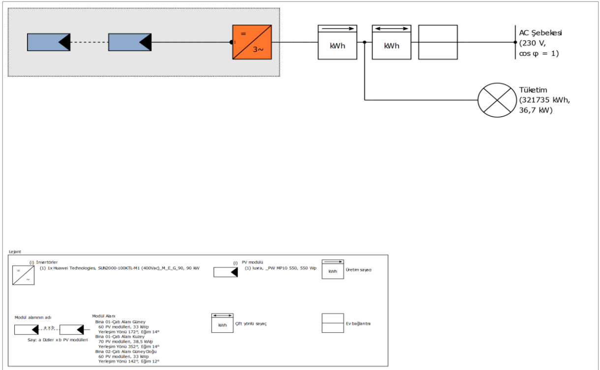
Şekil 3 2 Şematik Diyagram
