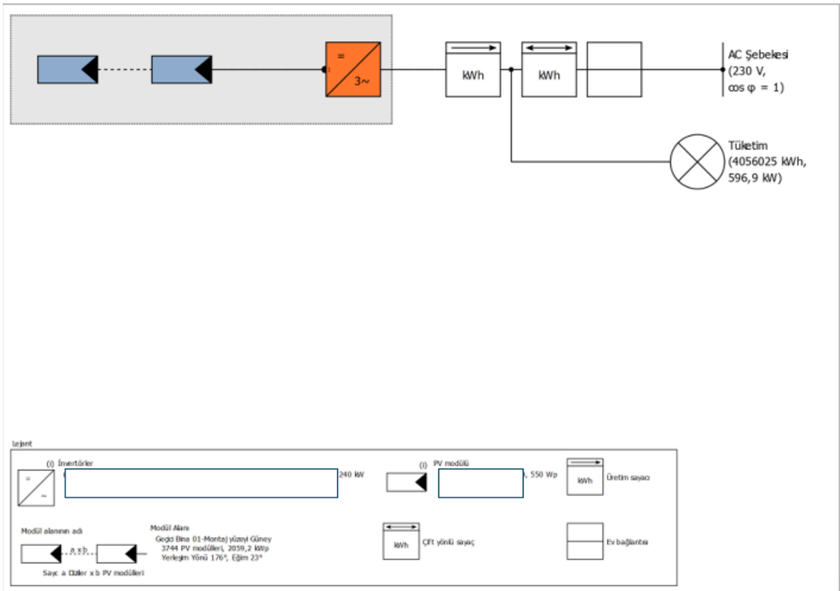
Şekil 3 2 Şematik Diyagram
