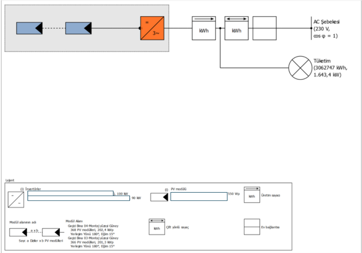
Şekil 3 2 Şematik Diyagram
