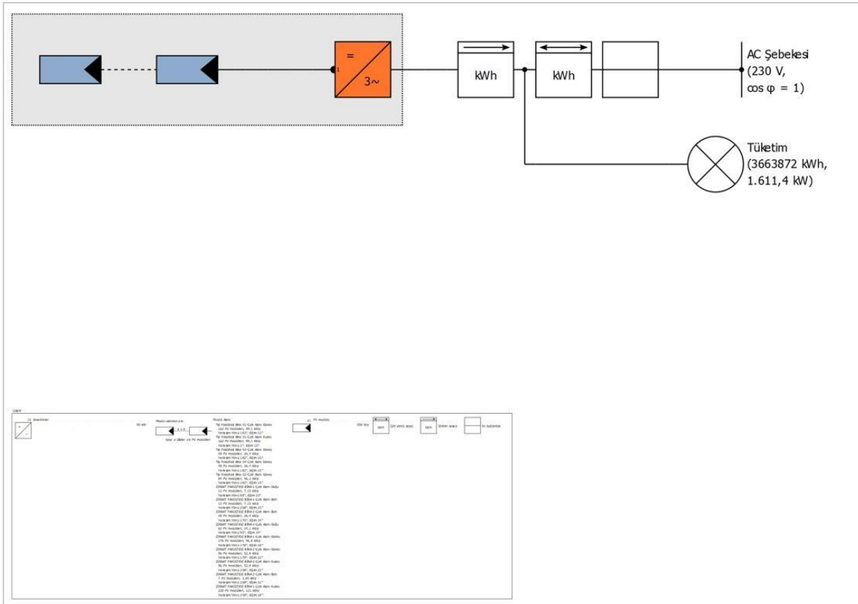
Şekil 3 2 Şematik Diyagram
