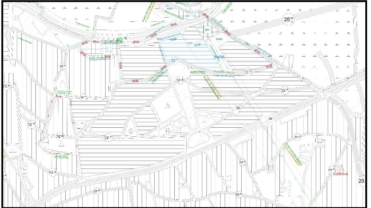
Şekil 6- 1/5000 Ölçekli Nazım İmar Planı
