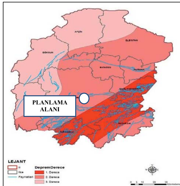
Şekil 3: Kahramanmaraş İli Deprem Bölgeleri Haritası
