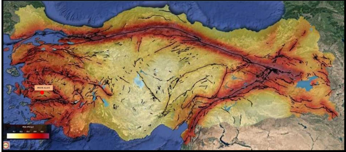
Şekil 21 Türkiye Sismik Tehlike Haritası
