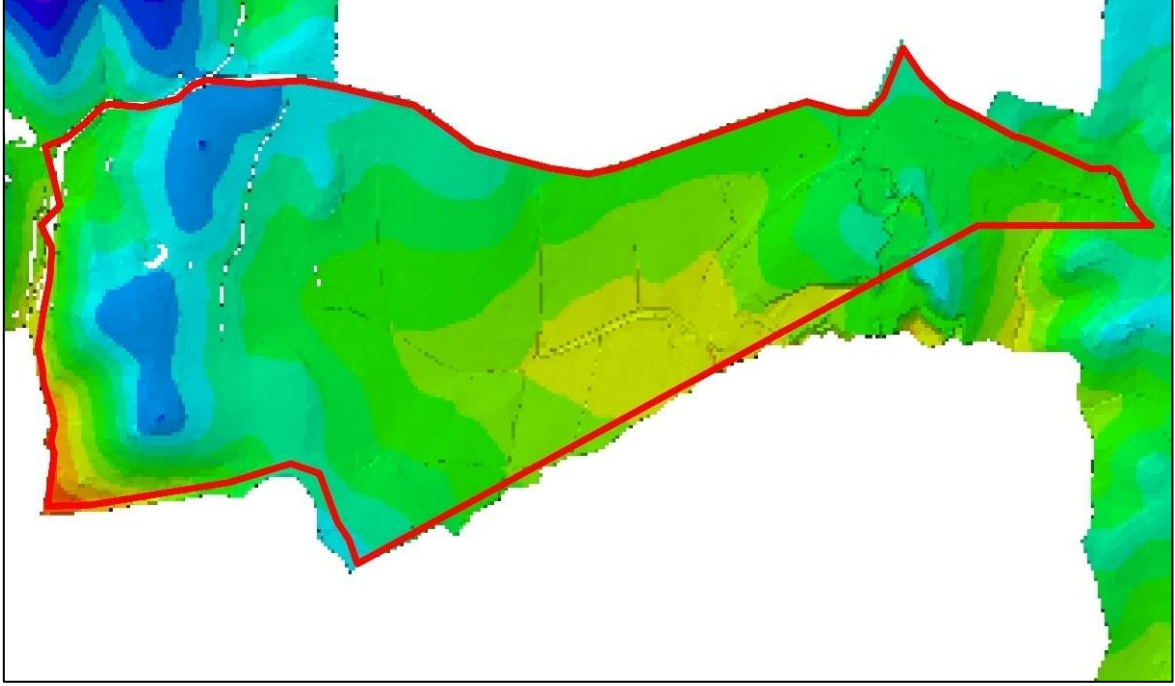
Harita 7: Rölöf Analizi
