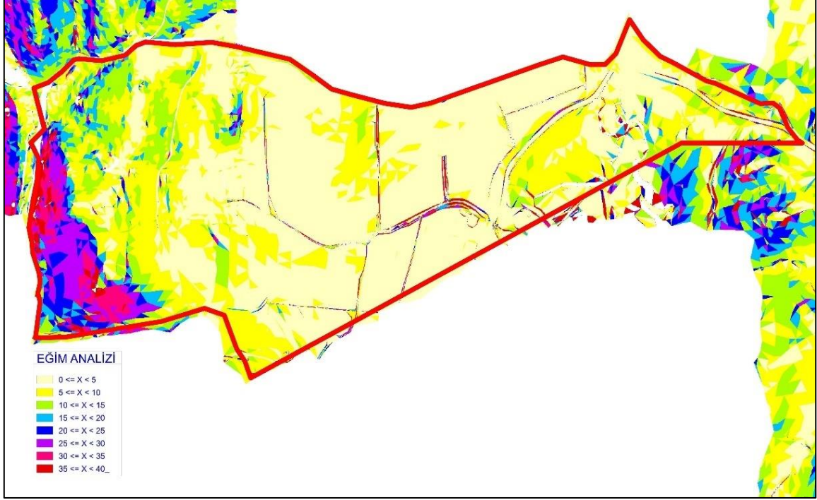
Harita 5: Eğim Analizi
