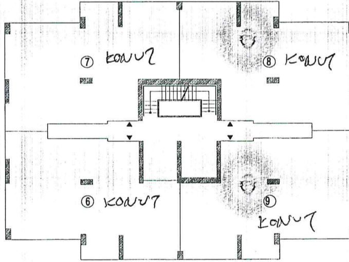
H3 BLOK 2. KAT PLANI Ö:1/200
