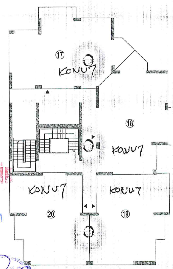
F2 BLOK 5. KAT PLANI Ö:1/200
