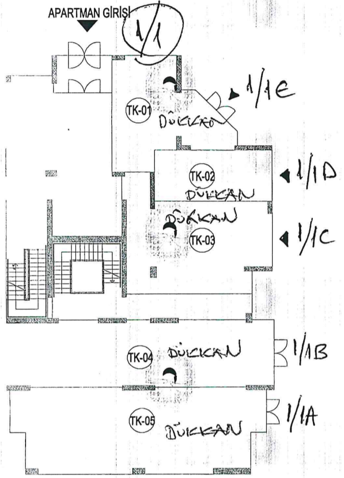
F2 BLOK ZEMİN KAT PLANI Ö:1/200
