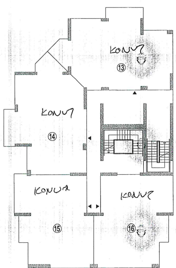
F1 BLOK 4. KAT PLANI Ö:1/200
