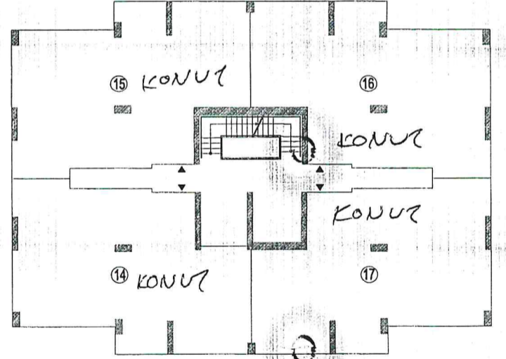
H3 BLOK 4. KAT PLANI Ö:1/200
