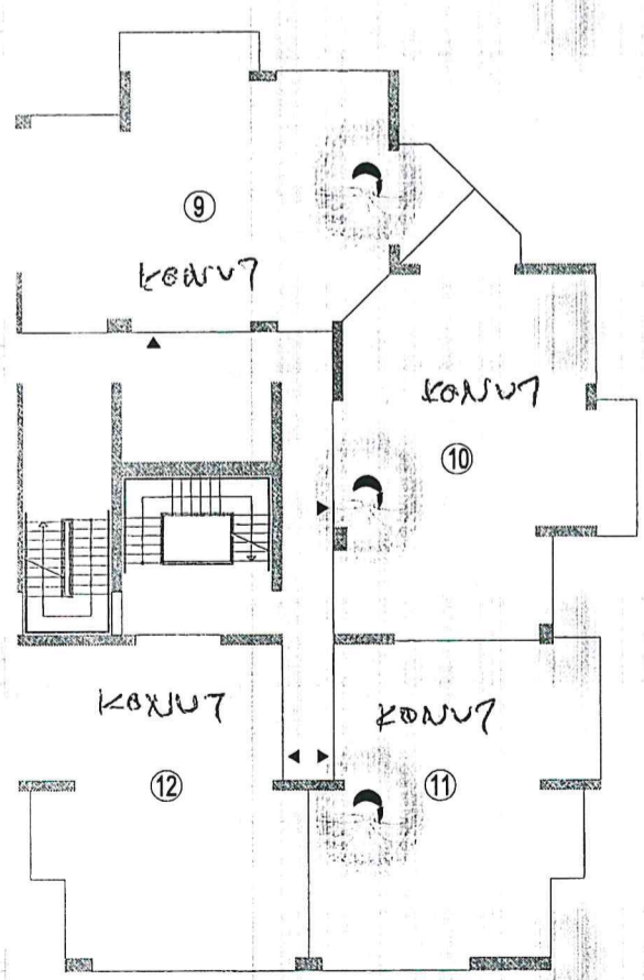
F2 BLOK 3. KAT PLANI Ö:1/200
