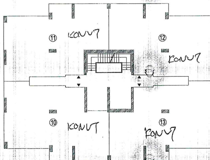
H3 BLOK 3. KAT PLANI Ö:1/200
