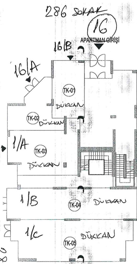
F1 BLOK ZEMİN KAT PLANI Ö:1/200
