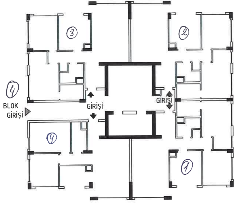
ZEMİN KAT
