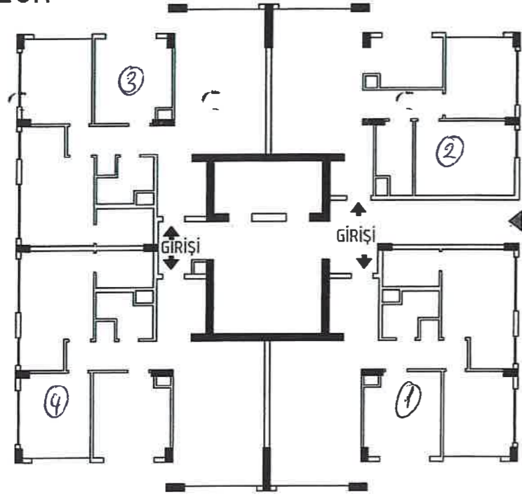
ZEMİN KAT
