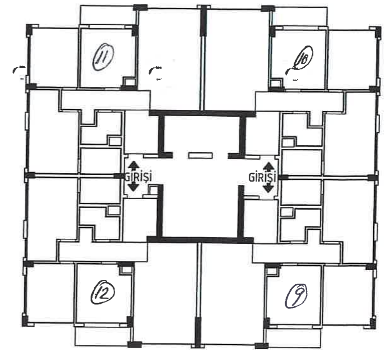
2.KAT
