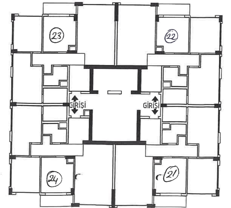
5.KAT
