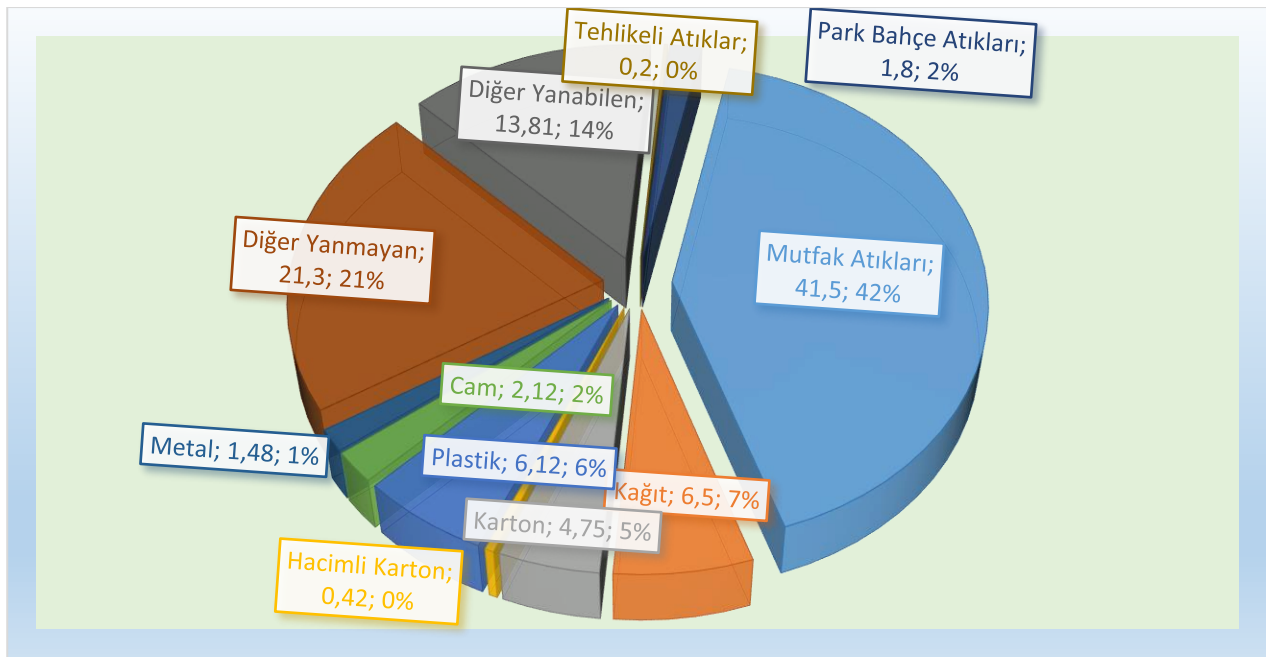
Grafik 18 - 2021 Yılı İtibariyle Katı Atık Kompozisyonu (Giresun İli Katı Sıvı Atık ve İçme Suları Birliği,2022)
