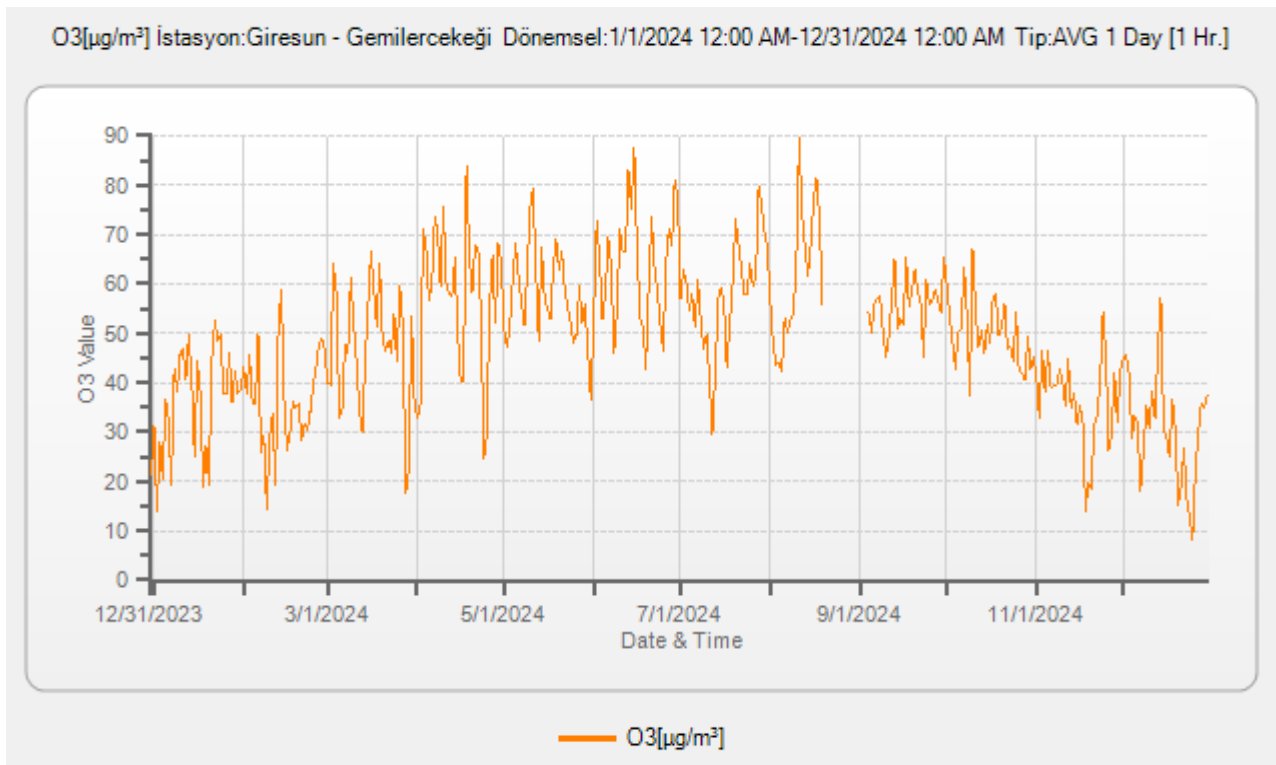
Grafik 10 -2024 Yılında Gemilercekeği İstasyonu O 3 Parametresi Günlük Ortalama Değer Grafiği (havaizleme.gov.tr, 2025)
