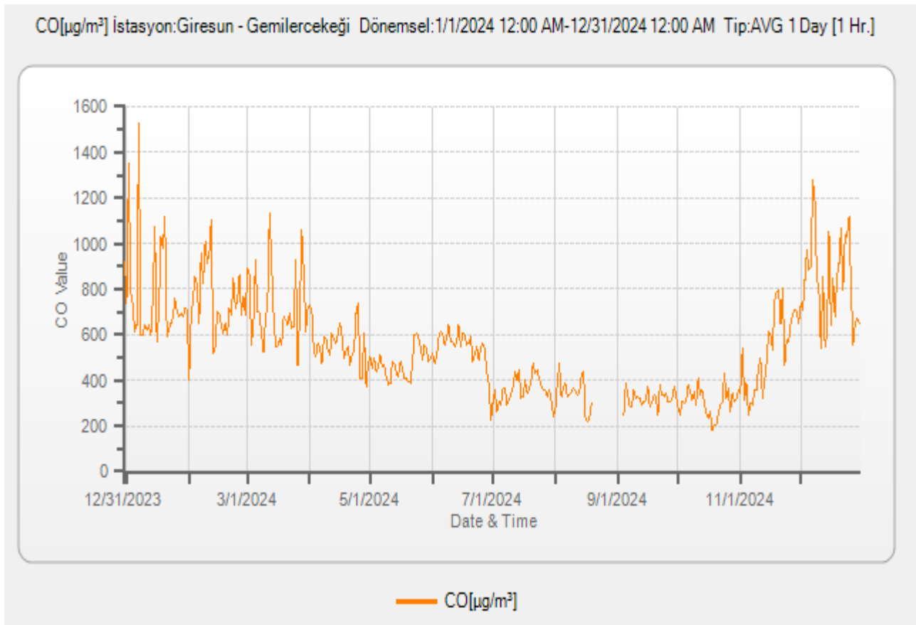
Grafik 9 2024 Yılında Gemilercekeği İstasyonu CO Parametresi Günlük Ortalama Değer Grafiği (havaizleme.gov.tr, 2025)
