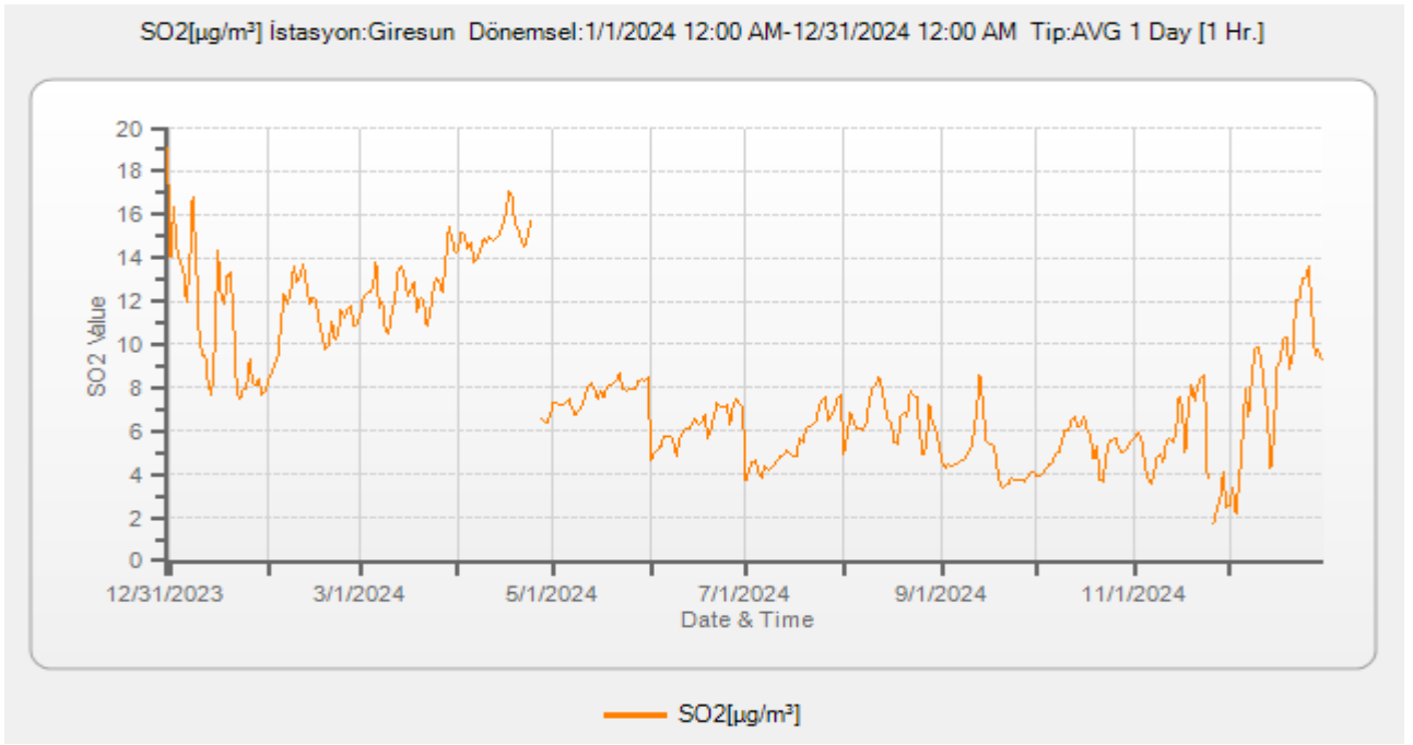
Grafik 2 - 2024 Yılında Giresun İstasyonu SO 2 Parametresi Günlük Ortalama Değer Grafiği (havaizleme.gov.tr, 2025)
