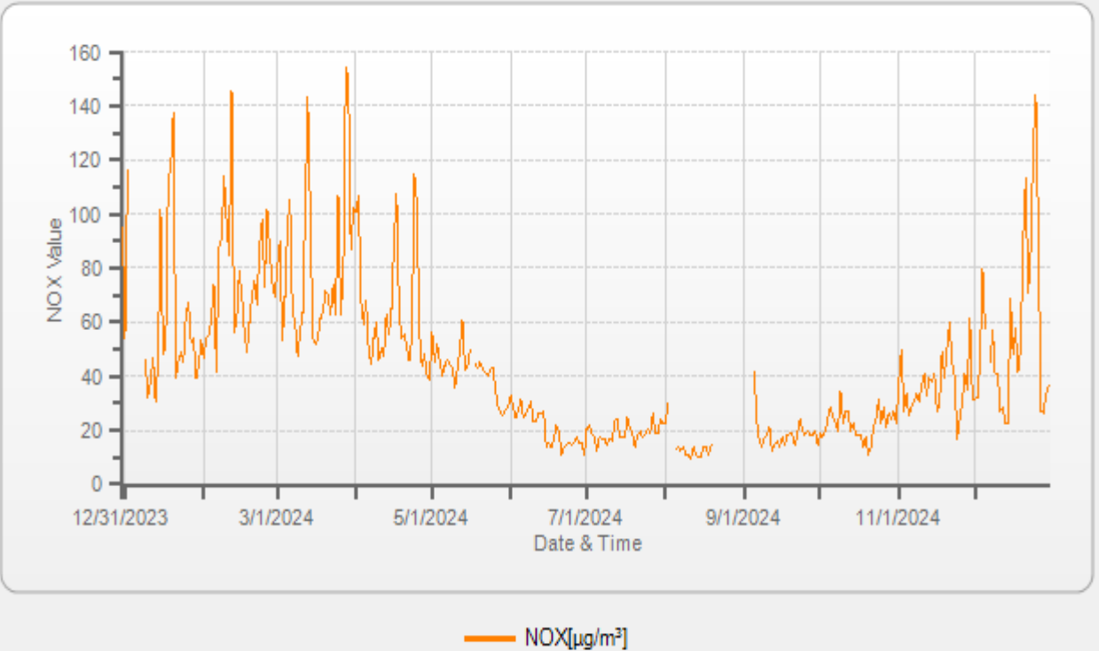
Grafik 8 - 2024 Yılında Gemilercekeği İstasyonu NO x Parametresi Günlük Ortalama Değer Grafiği (havaizleme.gov.tr, 2025)
