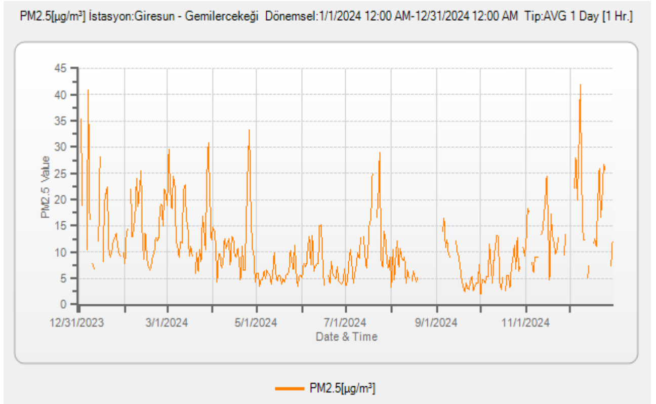
Grafik 4 - 2024 Yılında Gemilercekeği İstasyonu PM 2,5 Parametresi Günlük Ortalama Değer Grafiği (havaizleme.gov.tr, 2025)
