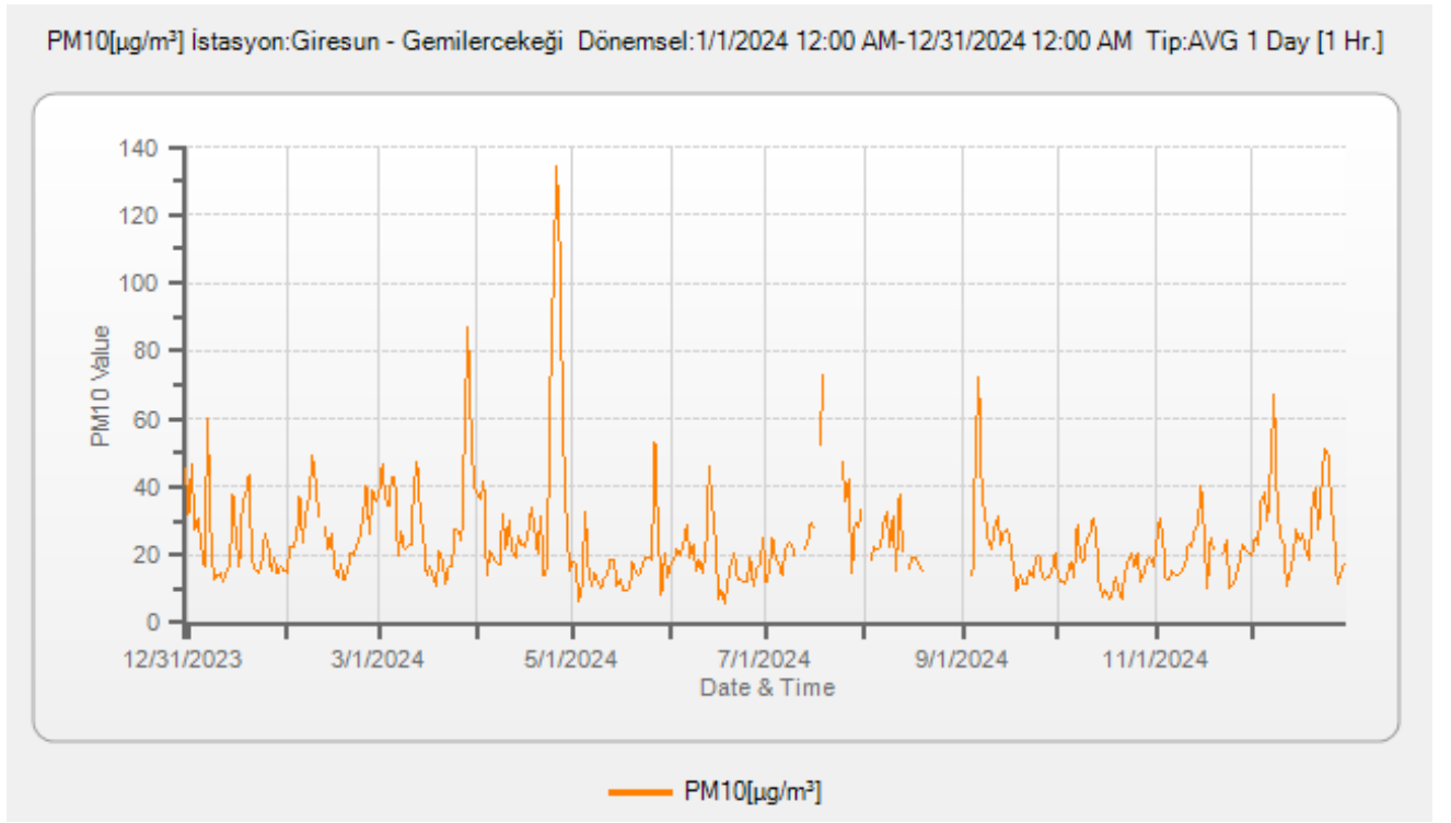
Grafik 3 - 2024 Yılında Gemilercekeği İstasyonu PM 10 Parametresi Günlük Ortalama Değer Grafiği (havaizleme.gov.tr, 2025)
