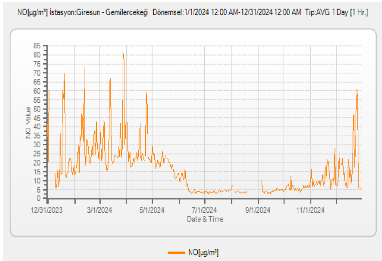
Grafik 6 - 2024 Yılında Gemilercekeği İstasyonu NO Parametresi Günlük Ortalama Değer Grafiği (havaizleme.gov.tr, 2025)
