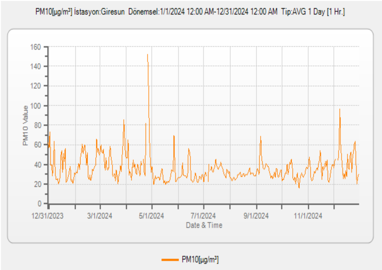
Grafik 1 - 2024 Yılında Giresun İstasyonu PM 10 Parametresi Günlük Ortalama Değer Grafiği (havaizleme.gov.tr, 2025)
