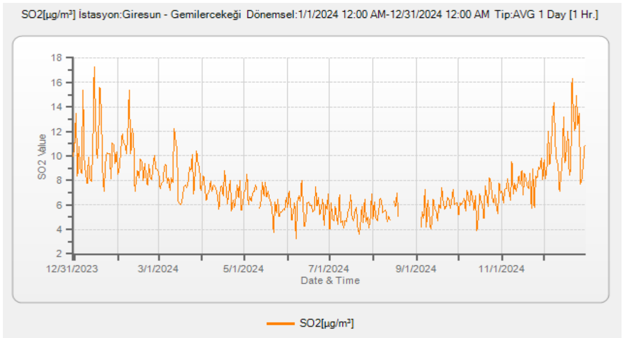
Grafik 5 2024 Yılında Gemilercekeği İstasyonu SO 2 Parametresi Günlük Ortalama Değer Grafiği (havaizleme.gov.tr, 2025)
