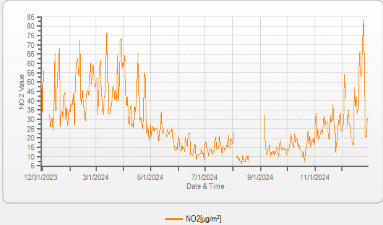
Grafik 7 - 2024 Yılında Gemilercekeği İstasyonu NO 2 Parametresi Günlük Ortalama Değer Grafiği (havaizleme.gov.tr, 2025)
