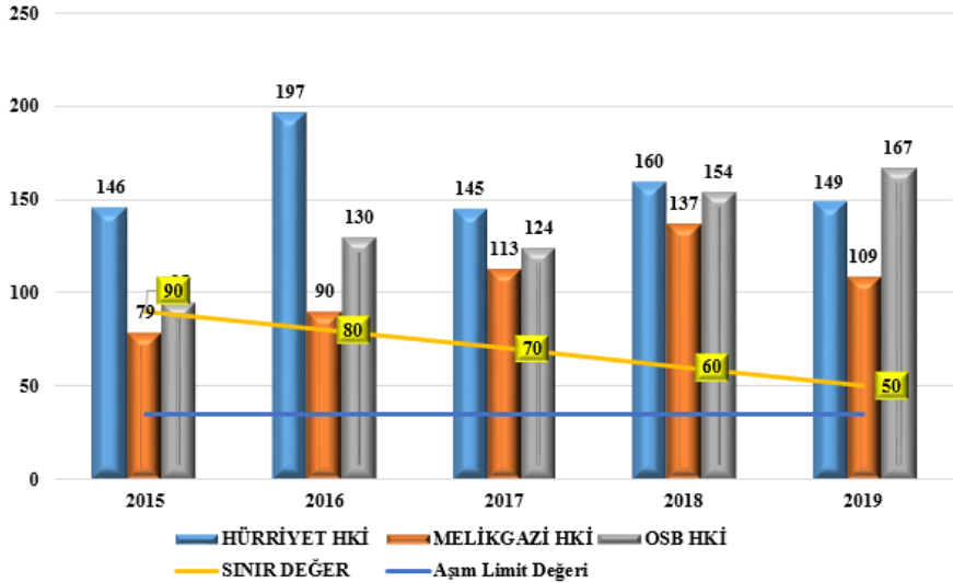
2015-2019 Yılları Arasında HKKY limit Aşım Değerlerine göre PM10 (24 saatlik) Aşım sayıları
