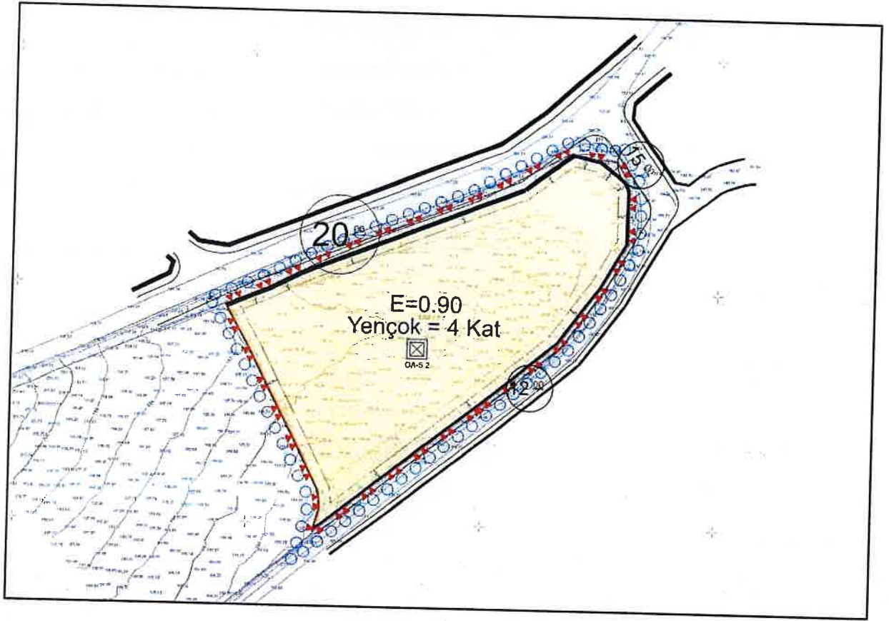
Harita 11: 1/1000 Ölçekli Uygulama İmar Planı
